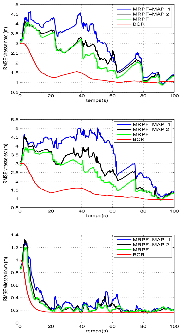
FIGURE 4.29 – RMSE en vitesse
