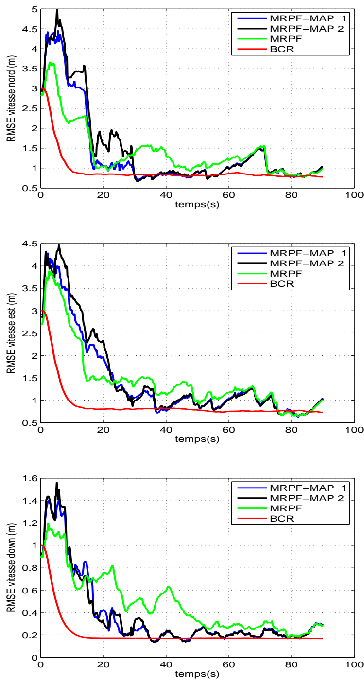
FIGURE 4.25 – RMSE en vitesse
