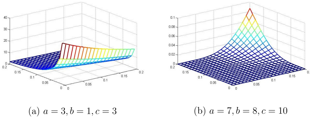
FIG. 2.3 – Représentation de la densité d'une loi Bêta bivariée de deuxième espèce.
