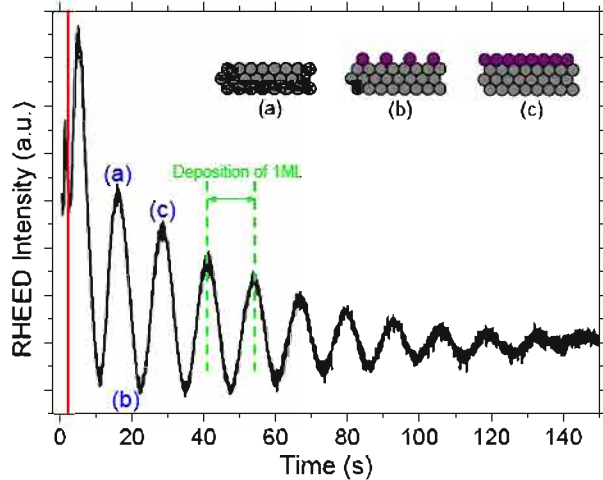
FIGURE 2.5: Oscillations en fonction du temps de l'intensité RHEED de la tache spéculaire. La ligne rouge représente l'instant de l'ouverture du cache de la cellule. En (a) et (c), la dernière couche atomique est remplie tandis qu'en (b), la couche est à moitié remplie. L'intensité des oscillations décroît en fonction du temps à cause de la rugosification de la surface. La première oscillation, plus courte à cause du "burst", n'est pas prise en compte.
