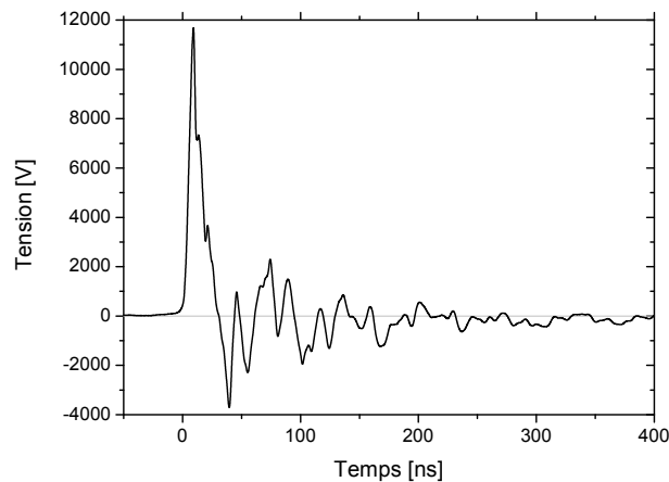
FIGURE 3.11 – Profil typique de tension mesurée aux bornes de la décharge NRP, en régime spark (défini dans la section 4.2.2).
