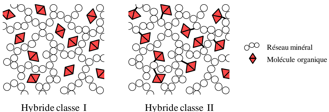
Figure 15 : Représentation schématique d'hybrides de classe I et de classe II.
