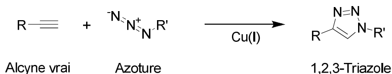
Schéma 15 : Schéma général de la réaction CuAAC
