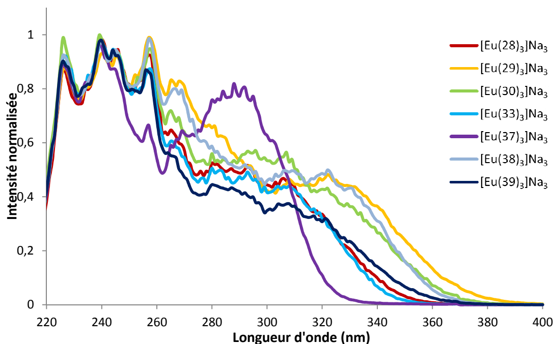
Figure 43 : Spectres d'excitation des complexes d'euprimum issus des diacides 28-30 , 33 , 37-39 .
