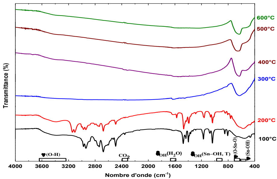
Figure II.14 : Spectres IR des poudres SnO 2 (al) en fonction de la température de calcination durant 1h.
