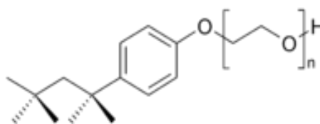
Figure II.13 : Formule chimique du Triton X-100 ® (TX-100).
