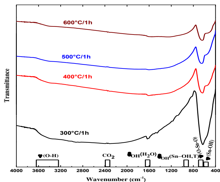
Figure II.26 : Spectres IR des poudres SnO 2 (al)-TX 0,3μl recuites pendant 1h à différentes températures.
