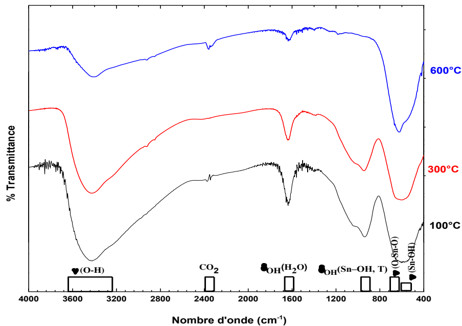
Figure II.16 : Spectres IR des poudres SnO 2 (aq) en fonction de la température de calcination pendant 1h.
