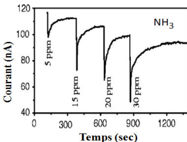
Figure I.19 : Réponses à température ambiante du capteur \text{SnO}_2 à différentes concentration de \text{NH}_3 [61].
