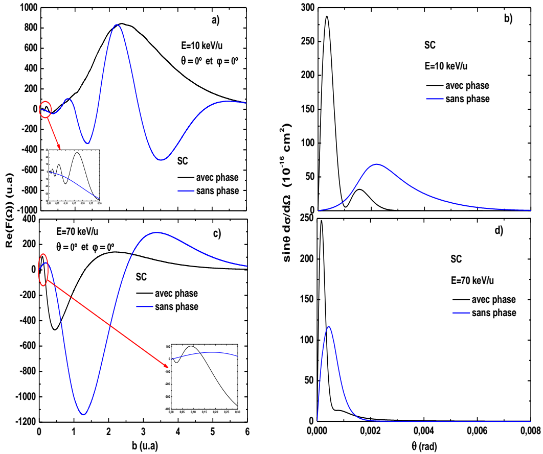
Figure 6.18 – Mêmes que la figure 6.16 mais pour le système H^+ - He .
