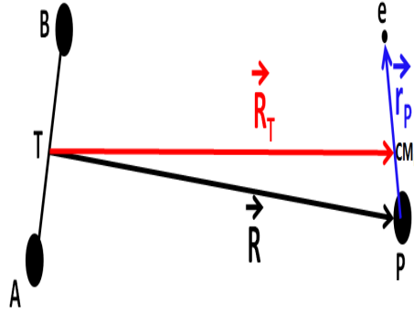
Figure 2.5 – Schéma après la collision s'il s'agit de capture où l'électron est lié au projectile P . CM_P : est le centre de masse de (P + e) .
