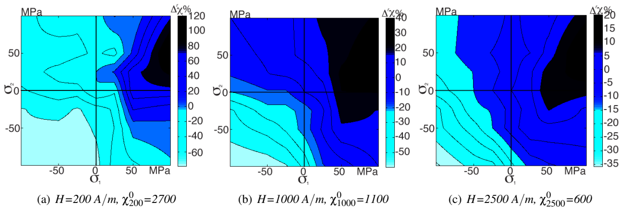
FIGURE 2.47: FeCo-2V R : Variation relative de la susceptibilité anhystérique sécante sous chargement mécanique biaxial \vec{H}/45^\circ .
