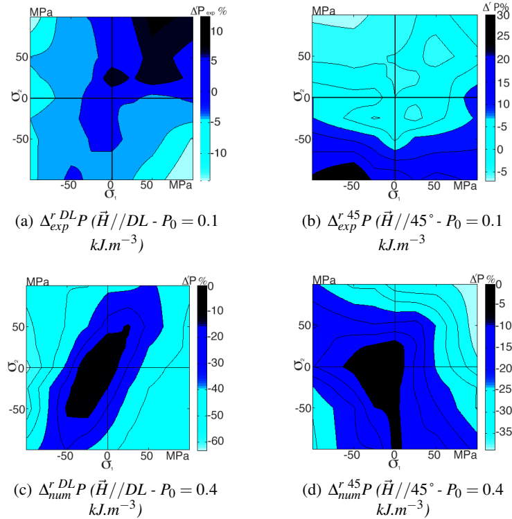
FIGURE 3.35: Fe-3%Si NO : Variations relatives des pertes \Delta^r P expérimentales (figs. a et b) et modélisées (figs. c et d) sous chargement mécanique biaxial ( H_{max} = 500 A/m).
