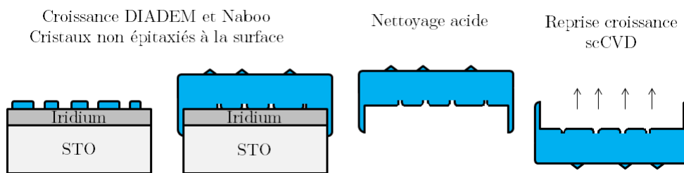
FIGURE 5.7 – Schéma explicatif du processus de recyclage et nettoyage acide des échantillons Ir/SrTiO 3 présentant des cristaux non épitaxiés.
