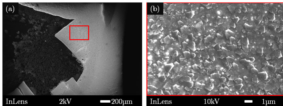
FIGURE 5.5 – (a) Film de diamant hétéroépitaxié délaminé au refroidissement et (b) surface présentant de nombreux cristaux non épitaxiés après la croissance de 4h avec les conditions scCVD dans Naboo.
