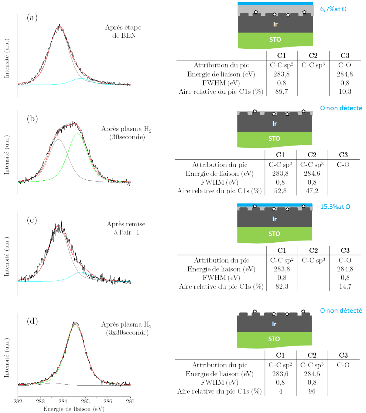
FIGURE 3.20 – Spectres XPS C1s déconvolués avec la représentation schématique associée de la surface de l'iridium lors de la gravure séquentielle de la couche de carbone amorphe des domaines.
