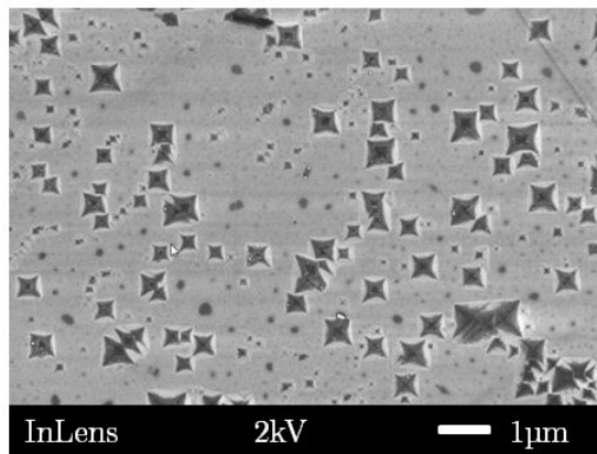
FIGURE 5.17 – Mise en évidence de la présence de dislocation par attaques acides chaudes.
