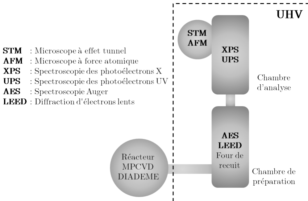
FIGURE 2.28 – Détails des outils d'analyse dans la partie UHV.
