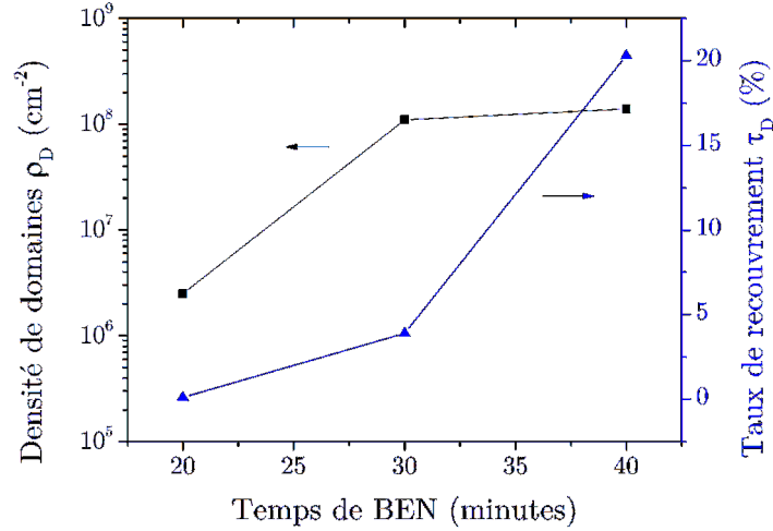
FIGURE 4.5 – Évolution temporelle (a) de la densité des domaines à la surface de l'iridium ainsi que (b) du taux de recouvrement au cours du BEN.
