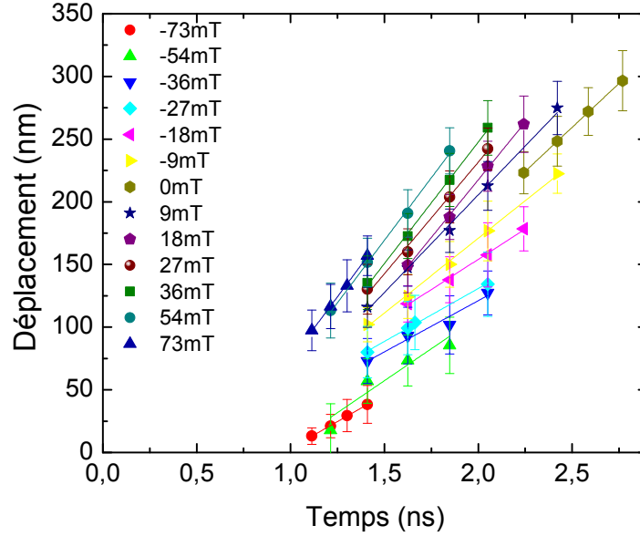
Figure III.4 – Déplacement de la paroi en fonction de la longueur d’impulsion pour différentes valeurs de champ longitudinal à courant constant ( J = 1,75 \times 10^{12} \text{ A/m}^2 ). Les déplacements sont donnés en valeur absolue et sont obtenus pour une paroi up/down soumise à l’action d’un courant négatif. La pente des ajustements linéaires (lignes continues) indique la vitesse de déplacement de la paroi.
