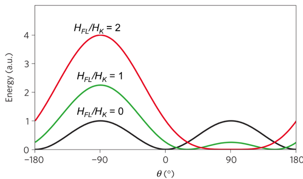
Figure I.19 – Profil d'énergie E(\theta) d'un matériau à anisotropie perpendiculaire illustrant la probabilité de renversement de l'aimantation en présence d'un champ effectif \mathbf{H}_{\text{FL}} orienté dans le plan de la couche. Le profil d'énergie est tracé pour différents rapports entre le champ effectif H_{\text{FL}} et le champ d'anisotropie effectif H_K . L'angle \theta représente l'angle entre l'aimantation et l'axe z de facile aimantation.
