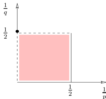
FIGURE 1.4 – zone admissible pour \mathbb{T}
