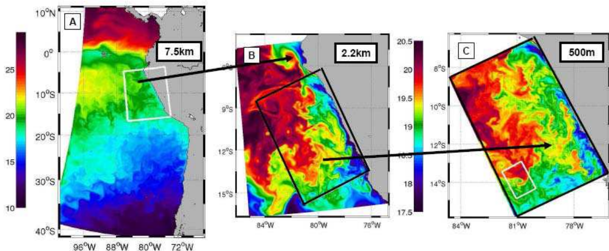
Fig. 4.1: Schéma d'une stratégie d'emboîtement multiple de grilles pour le HCS, allant des processus grande échelle aux processus sub-mésoéchelle: (A) configuration au 1/15° du modèle ROMS pour l'ESP utilisée par Colas et al. (2008); (B) grille emboîtée (résolution 2.2km) de l'océan côtier au Nord et au centre du Pérou; (C) grille de résolution 500m emboîtée dans (B) pour la côte centrale du Pérou. Les cartes représentent la TSM simulée (°C). L'échelle de couleurs pour (A) (resp. pour (B) et (C)) est indiquée sur le côté gauche (resp. droit) de la figure. F. Colas, communication personnelle.
