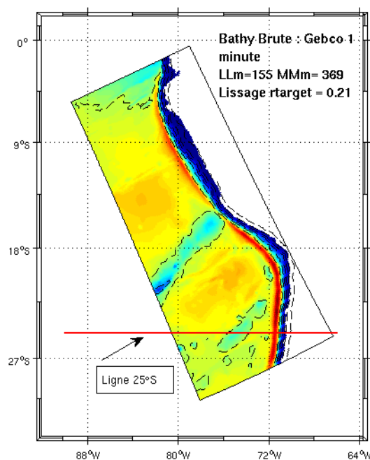
Fig. 4.9: grille curvilinéaire au 1/12^\circ emboîtée pour la configuration du modèle ROMS utilisée dans le programme PEPS. L'image d'arrière-plan représente la bathymétrie (m). G. Cambon, communication personnelle.
