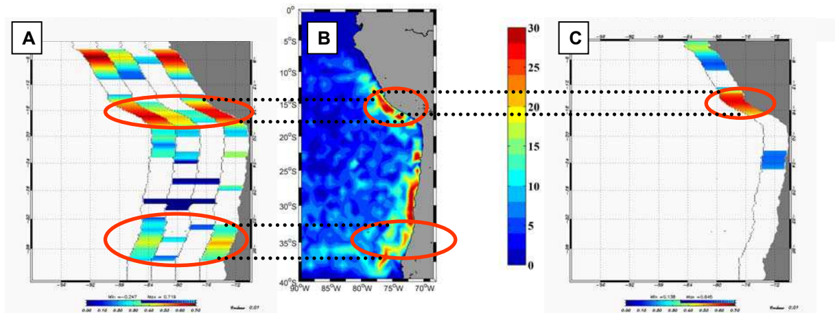
Fig. 4.7: (A) Maximum de la corrélation retardée (%) entre les variations à basse fréquence de l'énergie de l'ondelette dans la bande (50-80 \text{ jours})^{-1} pour respectivement les 3 premiers modes baroclines de l'EKW et le nombre de tourbillons côtiers, en fonction de la latitude; (B) carte de génération de tourbillons; (C) idem (A) mais pour la tension de vent méridional le long de la côte et le nombre de tourbillons côtiers pour la bande de fréquence (10-120 \text{ jours})^{-1} . Les 4 bandes en (A) correspondent à (resp. de gauche à droite) la somme des trois premiers, le troisième, le second, et le premier mode barocline de l'EKW. Seules les corrélations significatives sont tracées en (A) et (C).
