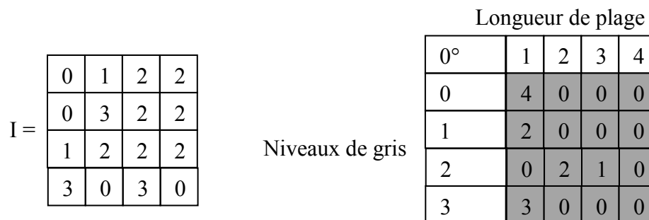
Figure 2.8 Exemple simple montrant la formation d'une matrice de longueur de plage. À gauche, une image de 4x4 pixels avec 4 niveaux de gris seulement. À droite, la matrice de longueur de plage résultante à 0^\circ . Le tableau en gris représente la matrice de longueur de plage.
