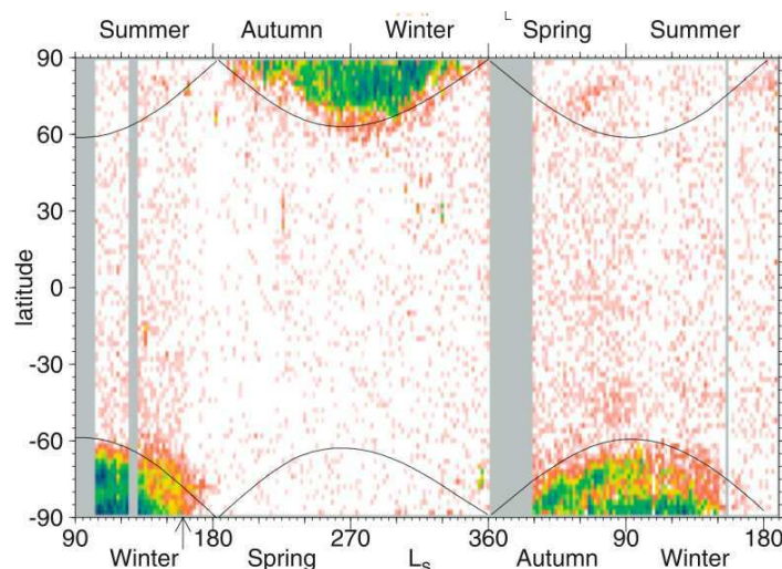
FIGURE I.27 – Cartographie des détections (par altimétrie laser) de nuages polaires (eau et \text{CO}_2 ) selon la latitude et la longitude solaire (Neumann et al., 2003). L'échelle de couleur, du rouge au bleu, correspond à un pourcentage croissant de retour d'échos par des nuages troposphériques (voir l'article de la référence pour détails).
