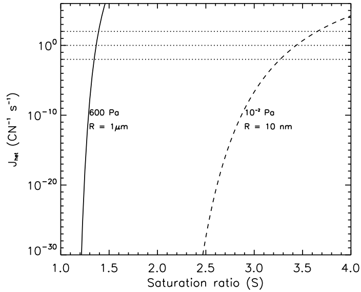
FIGURE II.9 – Taux de nucléation hétérogène ( J_{het} ) par particule (CN) et par unité de temps ( \text{s}^{-1} ) pour deux pressions atmosphériques différentes et deux tailles de CN différents : R = 1 \mu\text{m} à la surface ( 600 \text{ Pa} ) et R = 10 \text{ nm} dans la mésosphère à 10^{-2} \text{ Pa} ( \sim 80\text{-}90 \text{ km} ). On retrouve bien la saturation critique de 1,35 pour R = 1 \mu\text{m} (effet de courbure négligeable), valeur déterminée expérimentalement par Glandorf et al. (2002).
