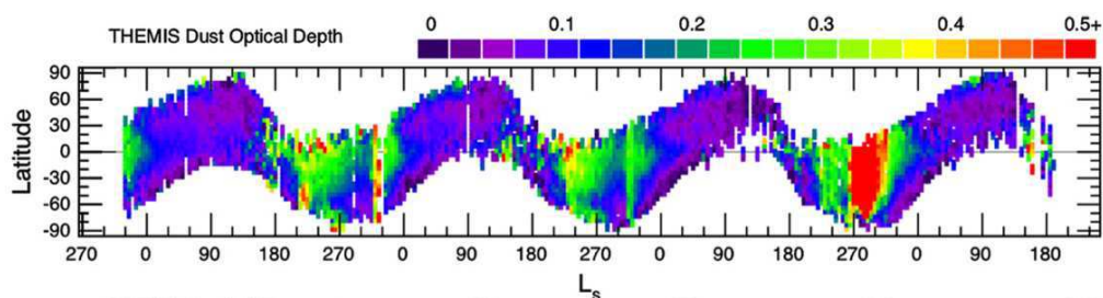
FIGURE I.19 – Variations latitudinales et saisonnières (en fonction de L_s ) de la profondeur optique des poussières en infrarouge (Smith, 2009). Le premier zéro en abscisse correspond au début de l'année MY26 (Mesures THEMIS, Mars Odyssey).
