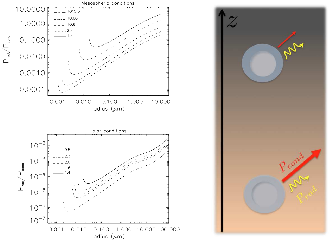
FIGURE II.39 – Rapport P_{rad}/P_{cond} de l'énergie dissipée par refroidissement radiatif P_{rad} et de l'énergie dissipée par conduction thermique P_{cond} , en fonction du rayon du cristal ( \mu m ), dans la nuit polaire à une pression de 80 Pa (en bas à gauche), et dans la mésosphère à une pression de 0,02 Pa (en haut à gauche). Chaque courbe correspond à différents rapports de saturations indexés sur les graphes. Termes évalués à partir des températures de surface T_a obtenues pour les taux de croissance CLASSIC montrés dans les Figures II.27 et II.28. A droite : schéma illustrant qualitativement l'importance relative du refroidissement radiatif ( P_{rad} ), par rapport au refroidissement par conduction thermique ( P_{cond} ) à deux altitudes distinctes.
