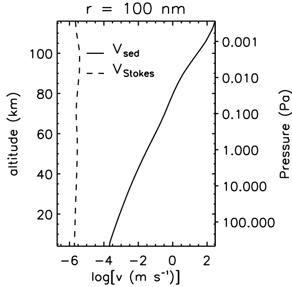
FIGURE III.3 – Vitesse de sédimentation v_{sed} ( m s^{-1} ) pour une particule de poussière de 100 nm, de densité \rho_d = 2500 \text{ kg m}^{-3} .
