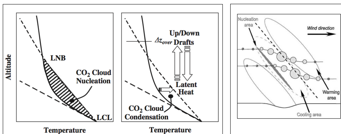
FIGURE I.28 – Deux modes de formation différents (mais non exclusifs) pour les nuages polaires de \text{CO}_2 . Un mode conjuguant l'effet d'ondes orographiques et des vents (à droite, schéma extrait de Tobie et al., 2003) et un mode privilégiant le potentiel convectif des nuages, à la manière des cumulus/cumulonimbus terrestres (à gauche, schémas extrait de Colaprete et al., 2008). Le schéma de gauche indique l'altitude minimale où la condensation peut déclencher une ascension de parcelle d'air (niveau LCL, pour Lifting Condensation Level) et celle où l'ascension de la parcelle doit en théorie cesser (niveau LNB, pour Level of Neutral Buoyancy), à l'endroit où l'adiabatique humide suivie par la parcelle rejoint le profil de température d'environnement. Mais des vitesses verticales peuvent entraîner des overshoot d'une hauteur \Delta z_{\text{over}} .
