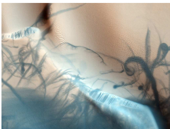
FIGURE I.16 – Traces laissées par le passage des dust devils, photographiées par HiRISE en août 2009. (Source :NASA/JPL/University of Arizona.)
