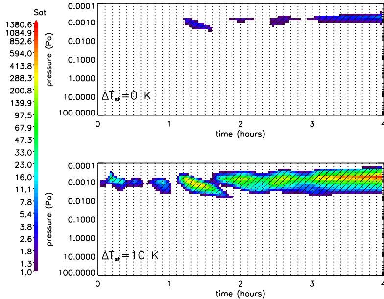
FIGURE IV.4 – Rapport de saturation S (en couleur) en fonction du temps écoulé (en heure) représentés là où S \geq 1 , pour les températures de nuit (Figure IV.2, droite) avec \Delta T_{shift} = 0 K (haut) et \Delta T_{shift} = 10 K (bas).
