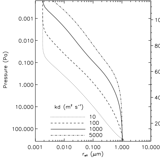
FIGURE III.13 – Profils verticaux du rayon effectif de la poussière pour les différents scénarios de mélange turbulent.
