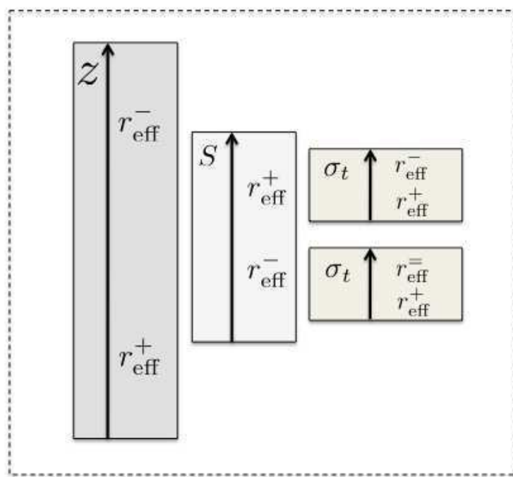
FIGURE III.24 – Schéma illustrant les influences principales de quelques variables sur le rayon effectif r_{\text{eff}} des cristaux : l'altitude z , le rapport de saturation S maximal atteint, et la durée de la poche froide \sigma_t . Les hauteurs relatives des blocs correspondent de façon qualitative à l'importance relative des variables dans l'évolution de r_{\text{eff}} (« + » : augmentation ; « - » : diminution ; « = » : pas d'effet particulier).
