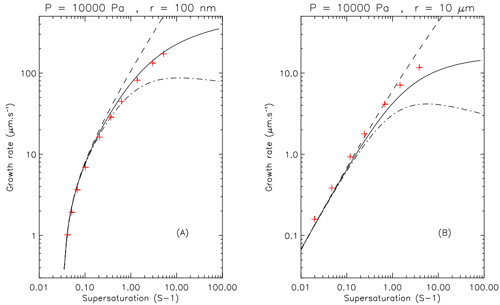
FIGURE II.36 – Idem que la figure II.34 dans des conditions caractéristiques d'une Mars primitive ( p \sim 10^4 Pa), pour deux rayons, 100 nm (A), et 10 \mu m (B).
