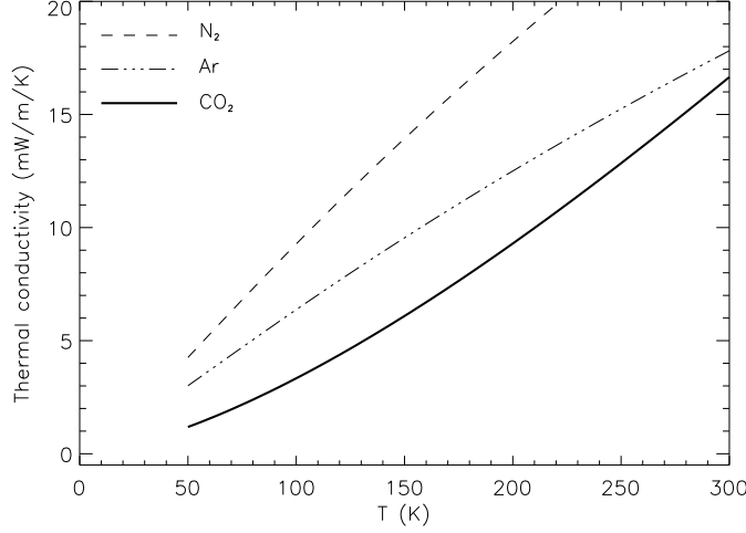
FIGURE II.23 – Conductivités thermiques ( \text{mW m}^{-1} \text{K}^{-1} ) du \text{CO}_2 , \text{N}_2 et Ar
