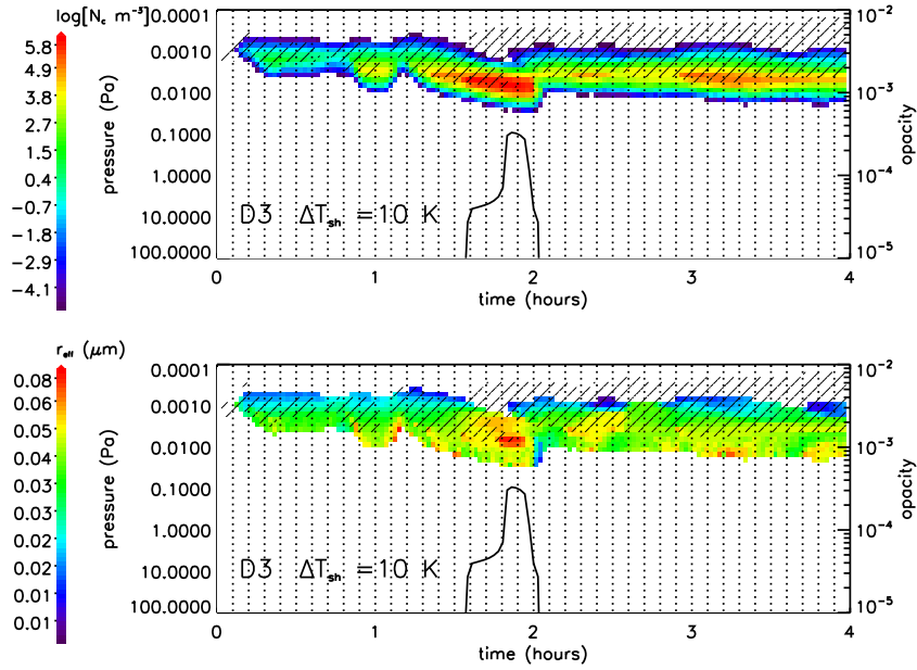
FIGURE IV.19 – Concentrations de cristaux (haut) et rayons effectifs (bas) obtenus à partir du profil D3 et \Delta T_{shift} = 10 K.
