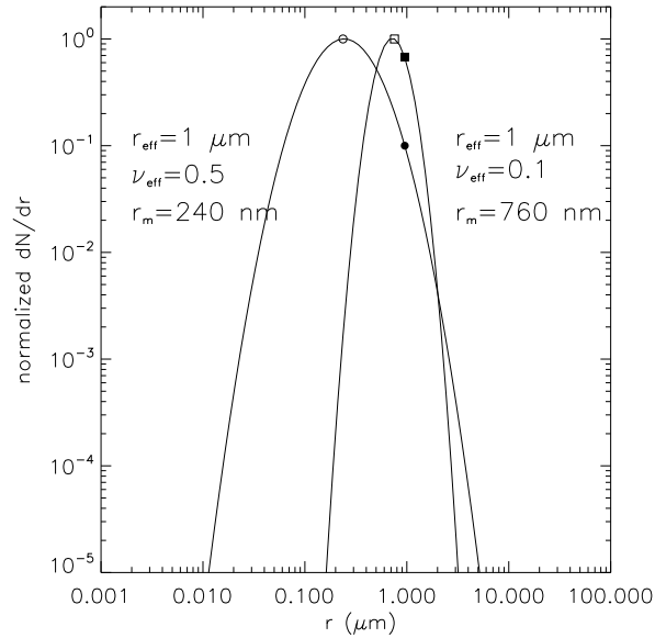
FIGURE III.10 – Une simple illustration de l'écart entre mode (symbole creux) et rayon effectif (symbole plein) de distributions log-normales
