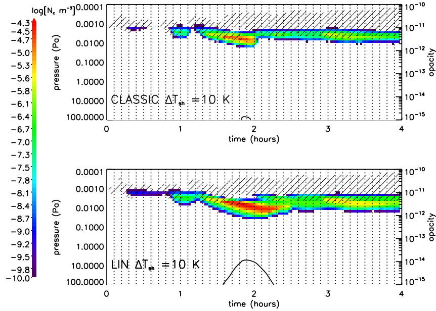
FIGURE IV.9 – Concentration volumique de cristaux ( \text{m}^{-3} , échelle log), correspondant au nuage illustré sur la Figure IV.8, pour le modèle CLASSIC (haut), et le modèle LIN (bas).
