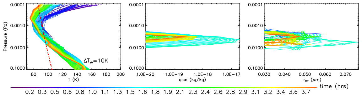
FIGURE IV.10 – Profils verticaux de (de gauche à droite) la température atmosphérique, le rapport de mélange de la glace ( \text{kg/kg} ) et le rayon effectif ( \mu\text{m} ) du nuage de nuit montré sur les parties supérieures des figures IV.9 et IV.8. Le point de condensation du CO 2 est indiqué (tirets).
