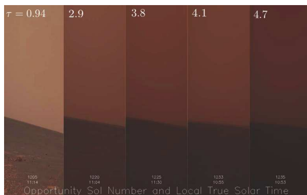
FIGURE I.2 – Mosaïque de clichés pris par Opportunity lors d’une tempête de poussière. L’opacité \tau de l’atmosphère est indiquée sur chaque cliché avec (en bas) le jour de la mission et l’heure locale. La période d’observation couvre ici 30 sols ou jours martiens, soit environ 31 jours terrestres. (Source : NASA/JPL.)
