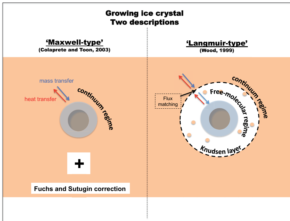
FIGURE II.14 – Schéma représentant les deux façons principales de décrire la croissance d'un cristal. A gauche : l'approche de Maxwell qui suppose un régime continu environnant et corrige les coefficients de transport pour rendre compte d'un éventuel régime transitoire ou cinétique. C2003 a opté pour cette approche en utilisant le modèle de croissance de Toon et al. (1989). A droite : l'approche de type Langmuir où deux régions sont considérées autour du cristal : une zone où le régime cinétique prévaut, et une zone, plus éloignée du cristal, où le régime est considéré comme étant continu (W1999 a utilisé cette approche). Ce deuxième mode de représentation est valable pour n'importe quel type de régime, et ne nécessite pas de correction des coefficients de transports. Source : Listowski et al. (2013)
