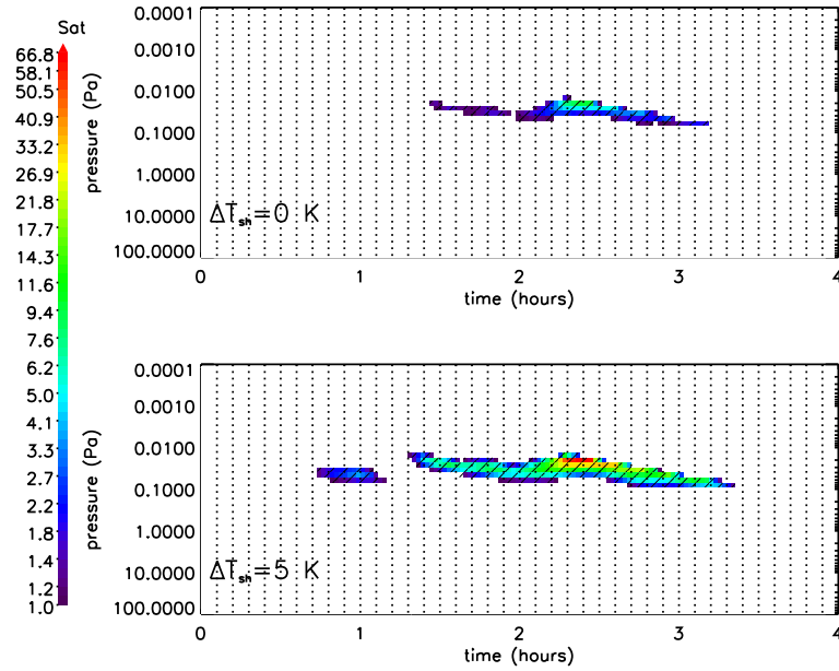
FIGURE IV.3 – Rapport de saturation S (en couleur) en fonction du temps écoulé (en heure) représenté là où S \geq 1 , pour les températures de jour (Figure IV.2, gauche) avec \Delta T_{shift} = 0 K (haut) et \Delta T_{shift} = 5 K (bas). L'axe vertical représente la pression atmosphérique. La partie hachurée représente les endroits où S > 1 et sera utilisée pour indiquer les zones sursaturées dans les figures suivantes.
