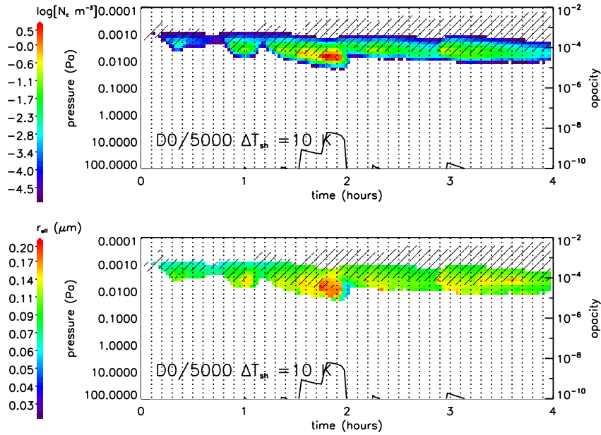
FIGURE IV.20 – Concentrations de cristaux (haut) et rayons effectifs (bas) obtenus à partir du profil D0/5000 et \Delta T_{shift} = 10 K.
