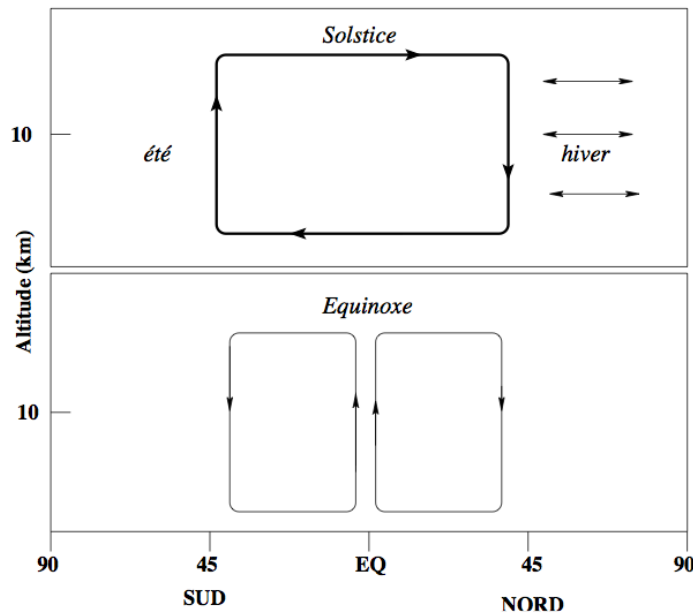
FIGURE I.18 – La circulation moyenne sur Mars (extrait de Montmessin, 2002). Autour des solstices une unique cellule de Hadley permet de représenter la circulation moyenne, d'un hémisphère à l'autre. Autour des équinoxes, deux cellules permettent de représenter la circulation atmosphérique (comme sur Terre).
