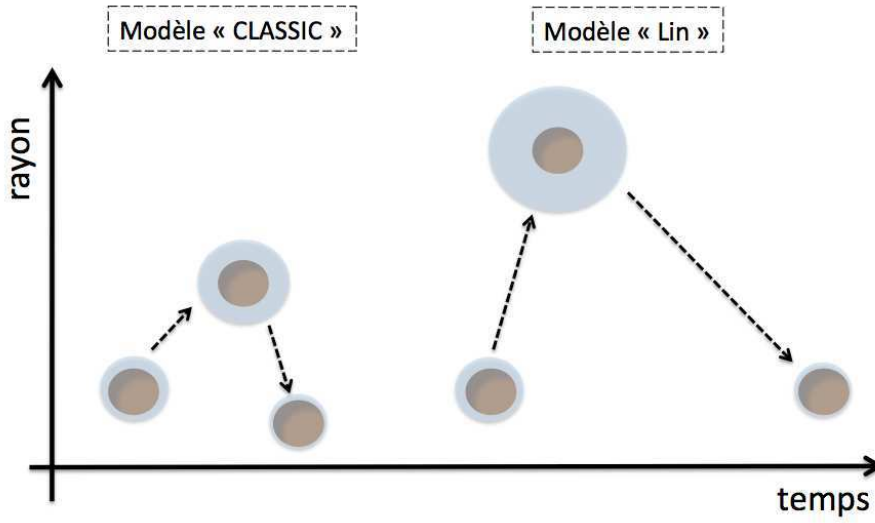
FIGURE II.30 – Schéma illustrant les différences qualitatives entre le modèle de croissance CLASSIC et le modèle linéarisé (LIN) sur la croissance et l'évaporation des cristaux de \text{CO}_2 .
