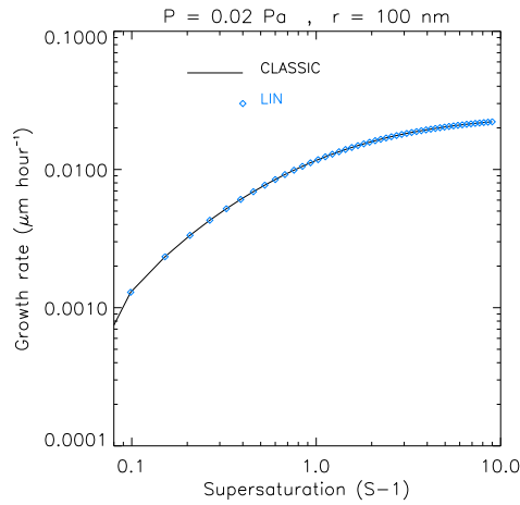
FIGURE II.31 – Accord des modèles CLASSIC (trait continu) et LIN (losanges) pour un gaz trace comme \text{H}_2\text{O} ( \mu\text{m}/\text{heure} ) dans des conditions mésosphériques pour une abondance x_v \ll 1 ( x_v = 100\text{ppm} ).
