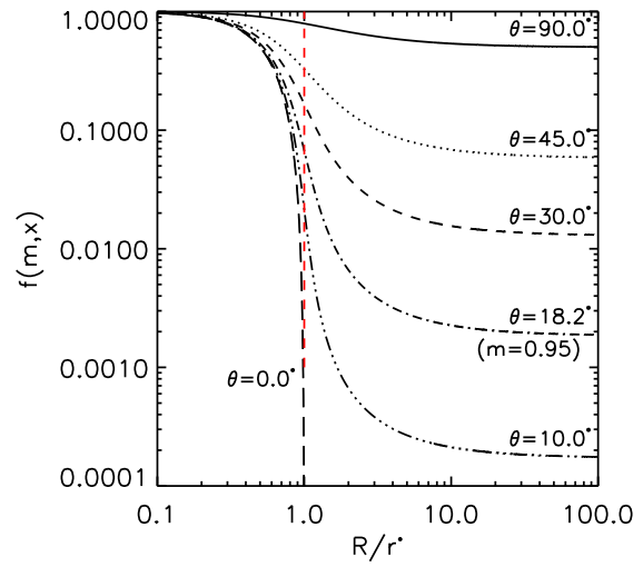
FIGURE II.5 – Fonction f(m, x) tracée en fonction de x = R/r^* pour plusieurs valeurs de l'angle \theta . L'angle correspondant au paramètre de contact de la glace de \text{CO}_2 ( m = 0,952 ) sur de la glace d'eau (Glandorf et al., 2002) est également indiqué.
