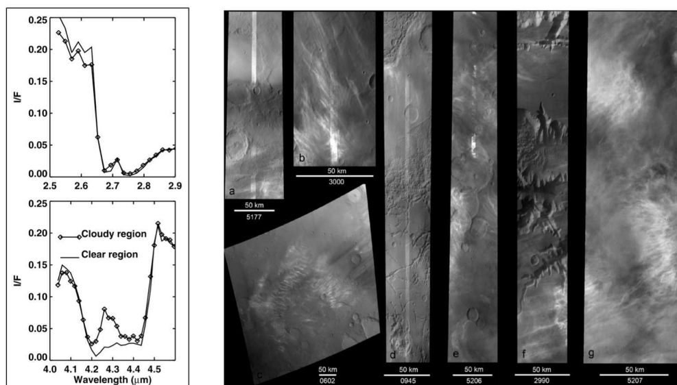
FIGURE I.30 – Nuages observés par HRSC (Mex) et identifiés comme étant des nuages de CO 2 (Määttänen et al., 2010) à l'aide de OMEGA, grâce à une signature spectral à 4,26μm (Montmessin et al., 2007). On distingue principalement des structures cirriformes (voir aussi plus bas au sujet des morphologies de nuages, et notamment Figure I.34).
