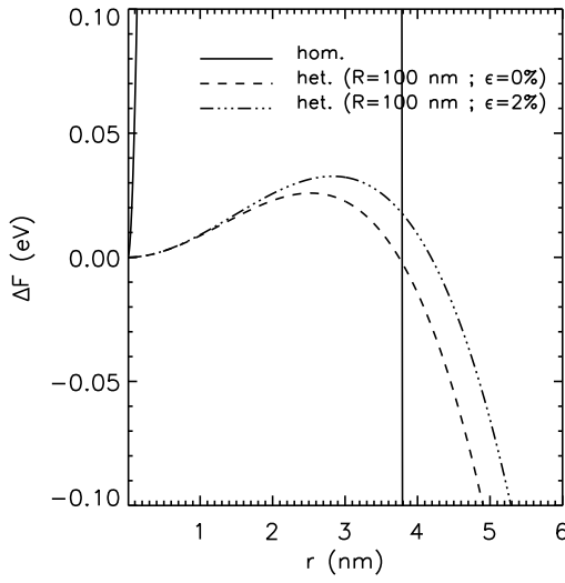
FIGURE II.6 – Conditions mésosphériques : p = 0.01 Pa et S = 10 . Energies de nucléation homogène (trait plein), hétérogène (pointillés), et hétérogène avec misfit (2%). La courbe de nucléation homogène, avec un seuil énergétique très haut, se devine à gauche et à droite.
