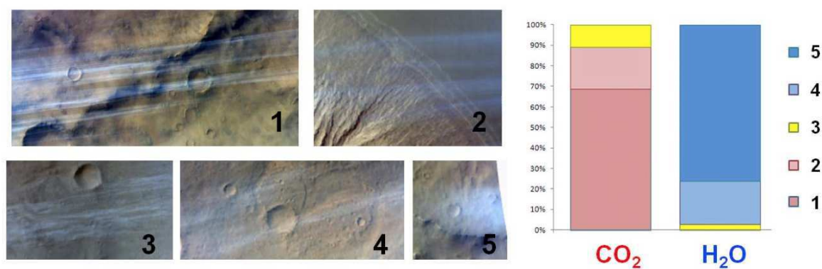
FIGURE I.34 – Comment classer les nuages d’eau et de CO 2 observés par CRISM? Proposition de cinq catégories de morphologies apparentes par Vincendon et al. (2011) : filaments droits et nets (1), filaments estompés (2), filaments ondulés (3), filaments diffus et très étirés (4), et formations ronde et diffuse (5). Les nuages de CO 2 appartiennent essentiellement aux catégories (1) et (2). Les nuages d’eau essentiellement aux catégories (4) et (5). Tous les nuages observés, notamment les nuages d’eau, ne sont pas nécessairement dans la mésosphère.
