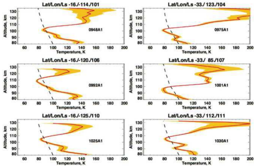
FIGURE I.38 – Profils sursaturés dans la mésosphère de Mars, obtenus par occultation stellaires. Les tirets indiquent le point de condensation du CO 2 . Source : Montmessin et al. (2011).
