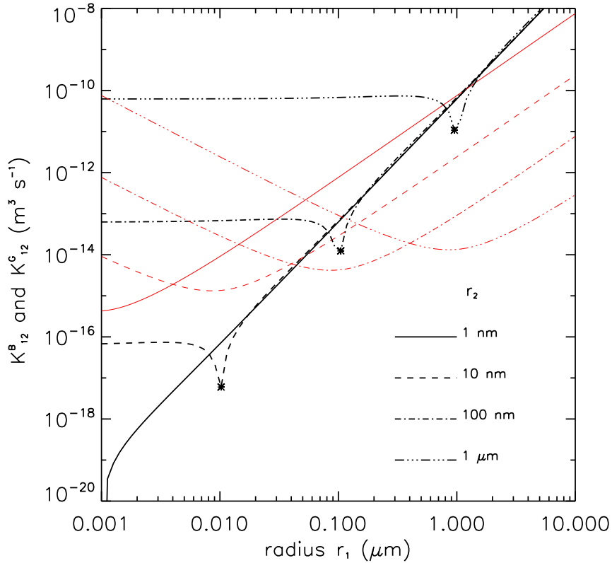
FIGURE III.9 – Coefficients de coagulation brownien ( K_B , en rouge) et gravitationnel ( K_G , en noir) en conditions mésosphériques ( p \sim 0.02 Pa soit \sim 70 -80 km.) pour différentes combinaisons de rayons r_1/r_2 , le premier correspondant à l'axe des abscisses. Les astérisques signalent une valeur tendant vers zéro pour K_G lorsque r_1 = r_2 .
