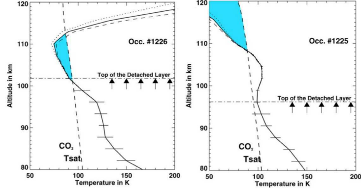
FIGURE I.32 – Profils de température obtenus par occultations stellaires en UV (SPICAM/ME) et montrant des poches sursaturées en CO 2 au dessus de couches d’aérosols dont l’altitude est reportée ici (Montmessin et al., 2006a). Les tirets indiquent le point de condensation du CO 2 .
