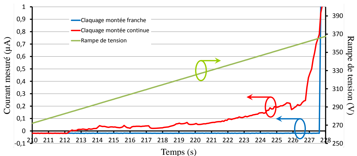
Figure 111 : Evolution typique du courant lors de deux essais ( d=1\mu m, plan Ru, à T_{\text{ambiante}} , sous air)
