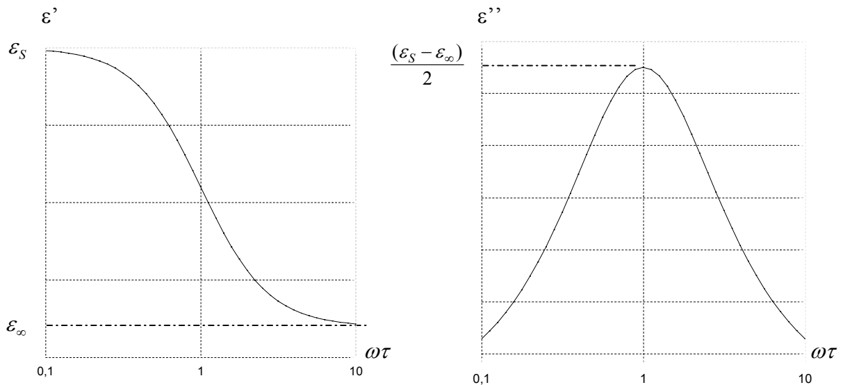
Figure II. 8 : variations théoriques de \epsilon'(\omega) et de \epsilon''(\omega)
