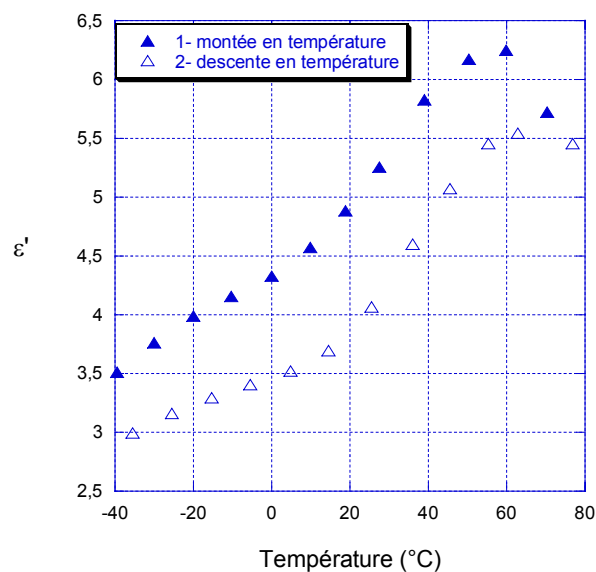
Figure II. 10 : variation de \varepsilon' du PVB en fonction de la température à 1kHz pour un cycle complet
