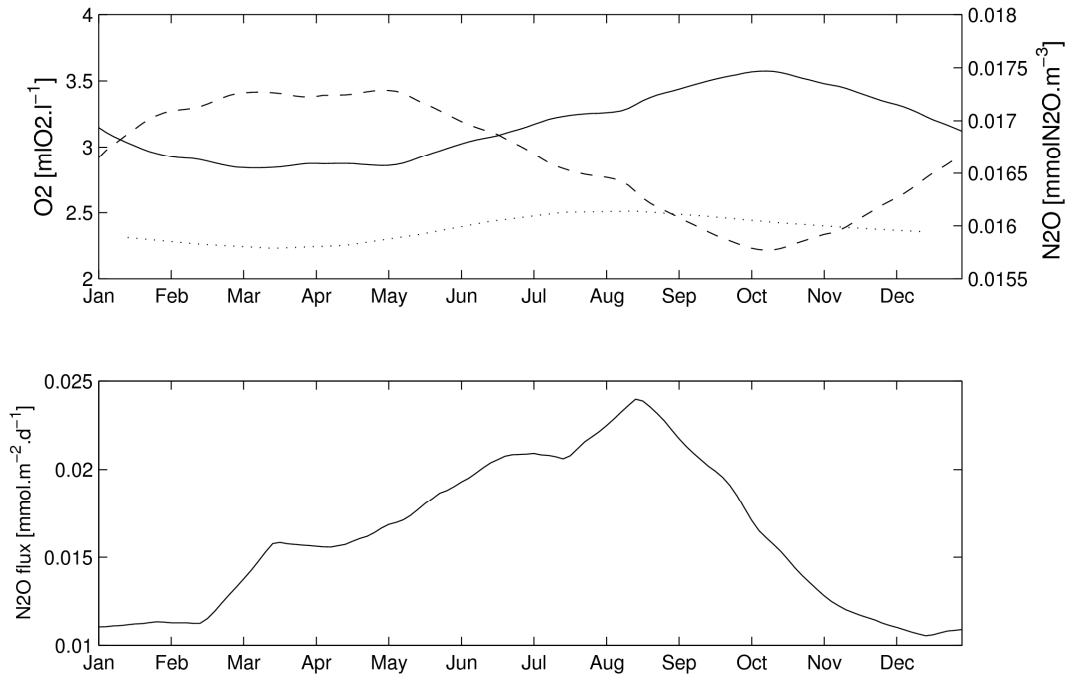
Figure 4.6: Cycle saisonnier des concentrations en oxygène (axe de gauche et ligne pleine : modèle, ligne pointillée : CARS 2006 ; mlO 2 .l -1 ) et en protoxyde d'azote (axe de droite et ligne tiretée ; mmolN 2 O.m -3 ) (en haut), moyennées entre 100 et 600 m, entre 22°S et 24°S et de la côte à la fin du talus continental (isobathe 2500 m). Cycle saisonnier du flux de N 2 O à l'interface océan-atmosphère (mmolN 2 O.m -2 .d -1 ), moyenné sur la même zone.
