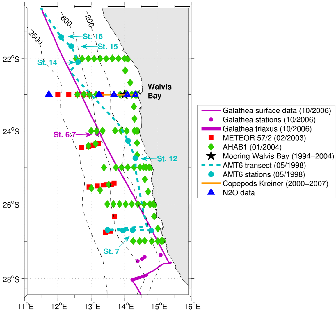
Figure 2.11: Stations et sections des campagnes utilisées pour la comparaison modèle-données: l'expédition danoise Galathea (Octobre 2006), l'expédition METEOR M57/2 (Février 2003), l'expédition AHAB1 (Janvier 2004), la campagne AMT 6 (Mai 1998), le mouillage à Walvis Bay entre 1994 et 2004 (Monteiro and van der Plas, 2006), la série temporelle d'abondance de copépodes au large de Walvis Bay de la côte (14.5°E) à 70 miles nautiques (13.23°E) entre 2000 et 2007 (Kreiner and Ayon, 2008), et les données de N 2 O issues de la campagne FRS Africana (Décembre 2009). Les lignes noires pointillées indiquent la bathymétrie (en mètres).
