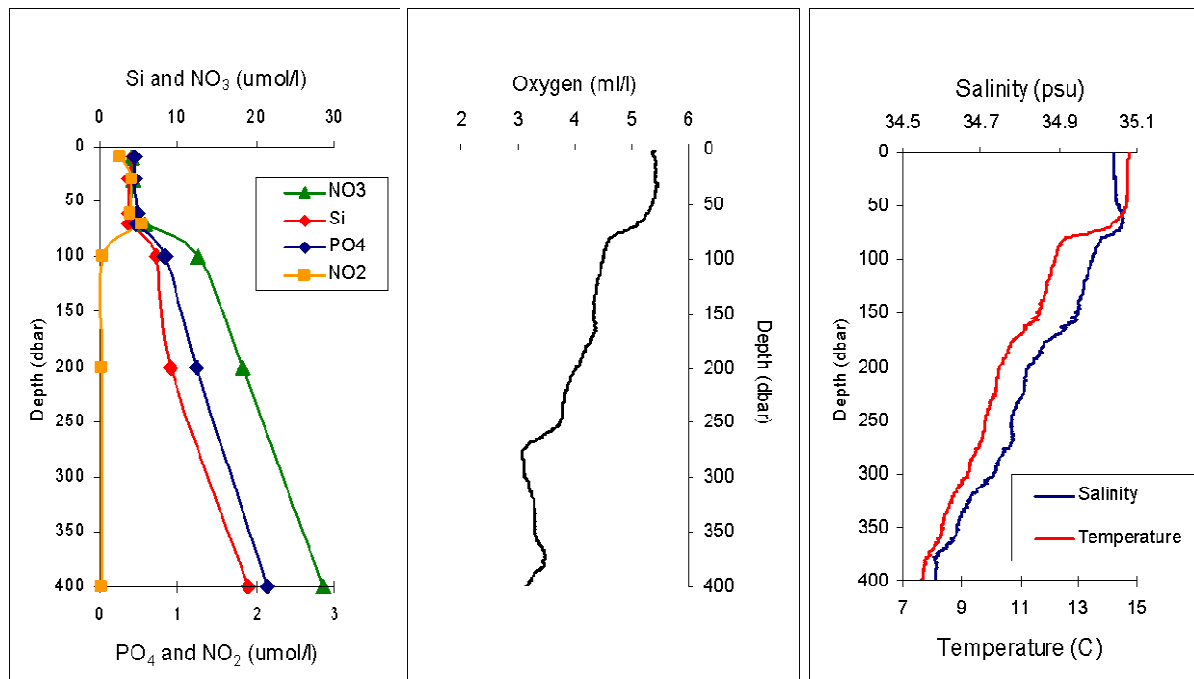
Figure 2.18: Profils verticaux de Si, NO 2 - , NO 3 - , PO 4 3- , O 2 , salinité et température à la station 6.17, échantillonnée le 13/10/2006, 27.53°S - 14.39°E.
