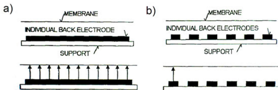
FIGURE 1.27 – a) Électrode continue rencontrée dans le cas d'un HPA. b) Partitionnement de l'électrode pour une utilisation en mode digital. Images tirées de [55]
