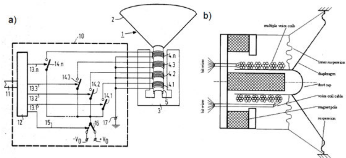
FIGURE 1.24 – a) Exemple d'un MCVDL possédant des bobines placées les unes derrières les autres. Image tirée de [51]. b) Exemple d'un MCVDL possédant des bobines placées les unes sur les autres. Image tirée de [40].
