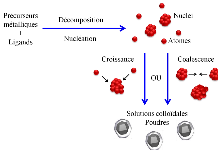
Figure 1-1 : Schéma illustrant les deux mécanismes de croissance (croissance ou coalescence de nuclei) de NPs en solution.
