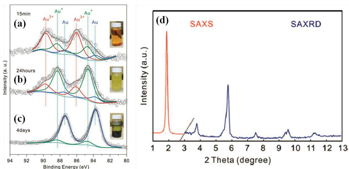
Figure 1-13 : (a-c) Analyses XPS des espèces d'or présentent à différents temps de réaction, en insert : photos de la solution pour chaque temps de réaction ; (b) Spectres combinés de SAXRD (bleu) et de SAXS (rouge) enregistrés sur le gel \text{Au}^{\text{+}} -oleylamine ( t = 24 \text{ h} ) 14 .
