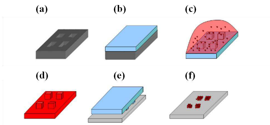
Figure 2-11 : Schéma représentant les différentes étapes de la technique de microcontact printing (a) Fabrication d'un moule en silicium ; (b) Moulage du timbre en élastomère (PDMS) ; (c) Encrage du timbre avec une goutte de solution ; (d) Séchage du timbre ; (e) Impression du timbre sur le substrat ; (f) Motifs moléculaires imprimés sur le substrat. (Extrait de la thèse de J.-C. Cau 126 )
