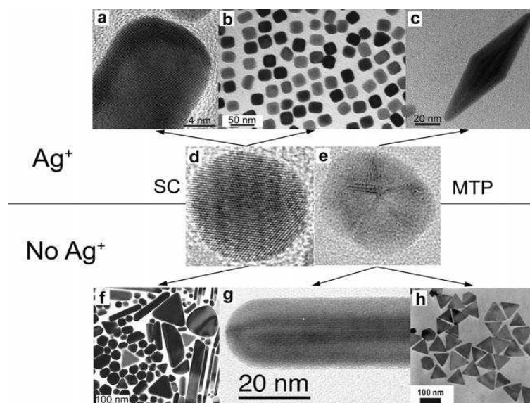
Figure 1-2 : Différentes morphologies de nanoparticules d'or formées à partir de germes (d) monocristallins (SC) ou (e) polycristallins (MTP), en (a-c) présence ou (f-h) absence de nitrate d'argent 24 .
