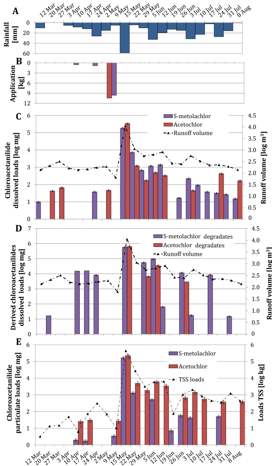
Figure 4. Variabilité temporelles des charges du S-métolachlore, de l'acétochlore et de leurs produits de dégradation dans la phase dissoute (<0,7 μm) et dans la phase particulaire (> 0,7 μm) à l'exutoire du bassin versant (Alteckendorf, Alsace, France). L'erreur totale a été estimée par propagation d'erreurs basée sur les incertitudes analytiques, ainsi que sur les incertitudes liées aux mesures des matières en suspension et des mesures de volume d'eau.
