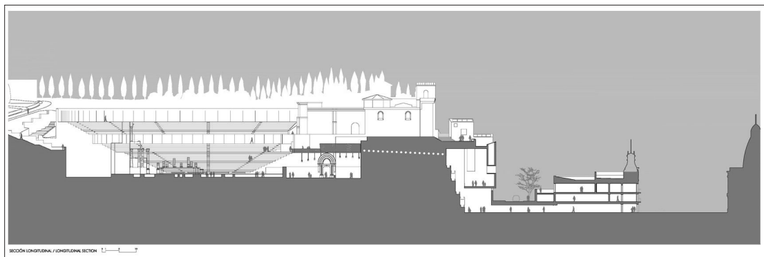
Figure 4.14 Section du musée du Théâtre romain. On peut voir les différents niveaux qui totalisent une différence de 25 mètres. (Archives du studio Rafael Moneo.)
