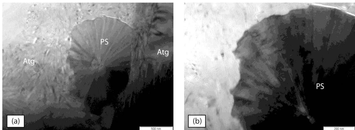
Figure II.7: (a) Image au MET d'un résidu de serpentinite océanique dans une serpentinite du massif du Lanzo. La photo montre la coexistence d'un cristal de serpentinite polygonale (PS) et de cristaux d'antigorite (b) Le cristal de serpentinite polygonale présente des secteurs dentelés de manière irrégulière suggérant sa dissolution et recristallisation en antigorite.
