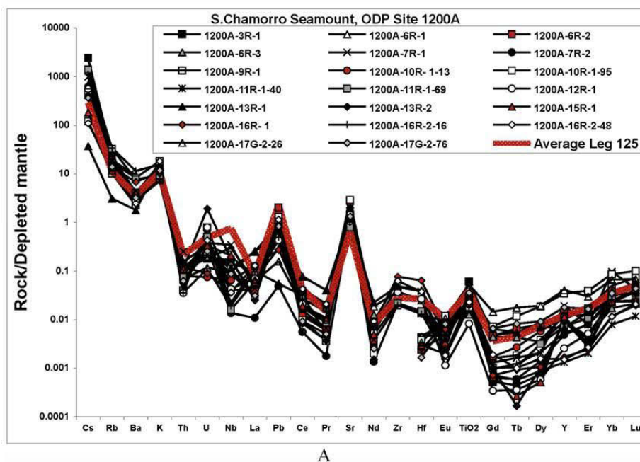
Figure I.20 : Exemple de spectres en éléments en trace des serpentinites des Mariannes, normalisés au manteau appauvri (Savov et al., 2007).
