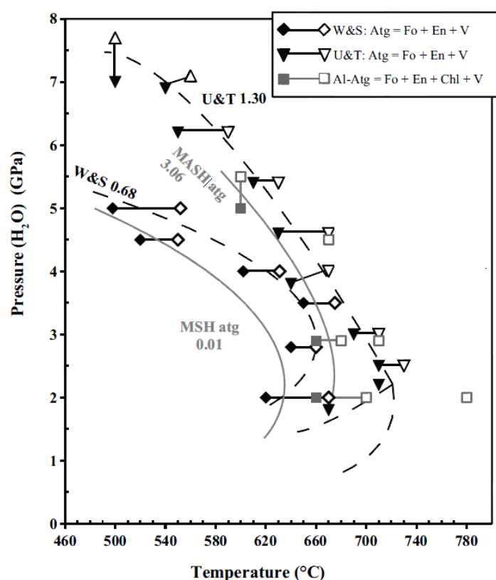
Figure 1.15 : Comparaison des différentes courbes de déshydratation de l'antigorite en fonction de la teneur en Al du minéral (Bromiley & Pawley, 2003). W&S : Wunder & Schreyer, 1997 ; U&T : Ulmer & Trommsdorff, 1995. Les chiffres sur les courbes indiquent les teneurs en \text{Al}_2\text{O}_3 des antigorites. Les résultats de l'étude de Ulmer & Trommsdorff, 1995 divergent de ceux de l'étude de Bromiley & Pawley (2003) ce qui suggère que la présence d'Al n'est pas le seul paramètre contrôlant la stabilité de l'antigorite à HT.
