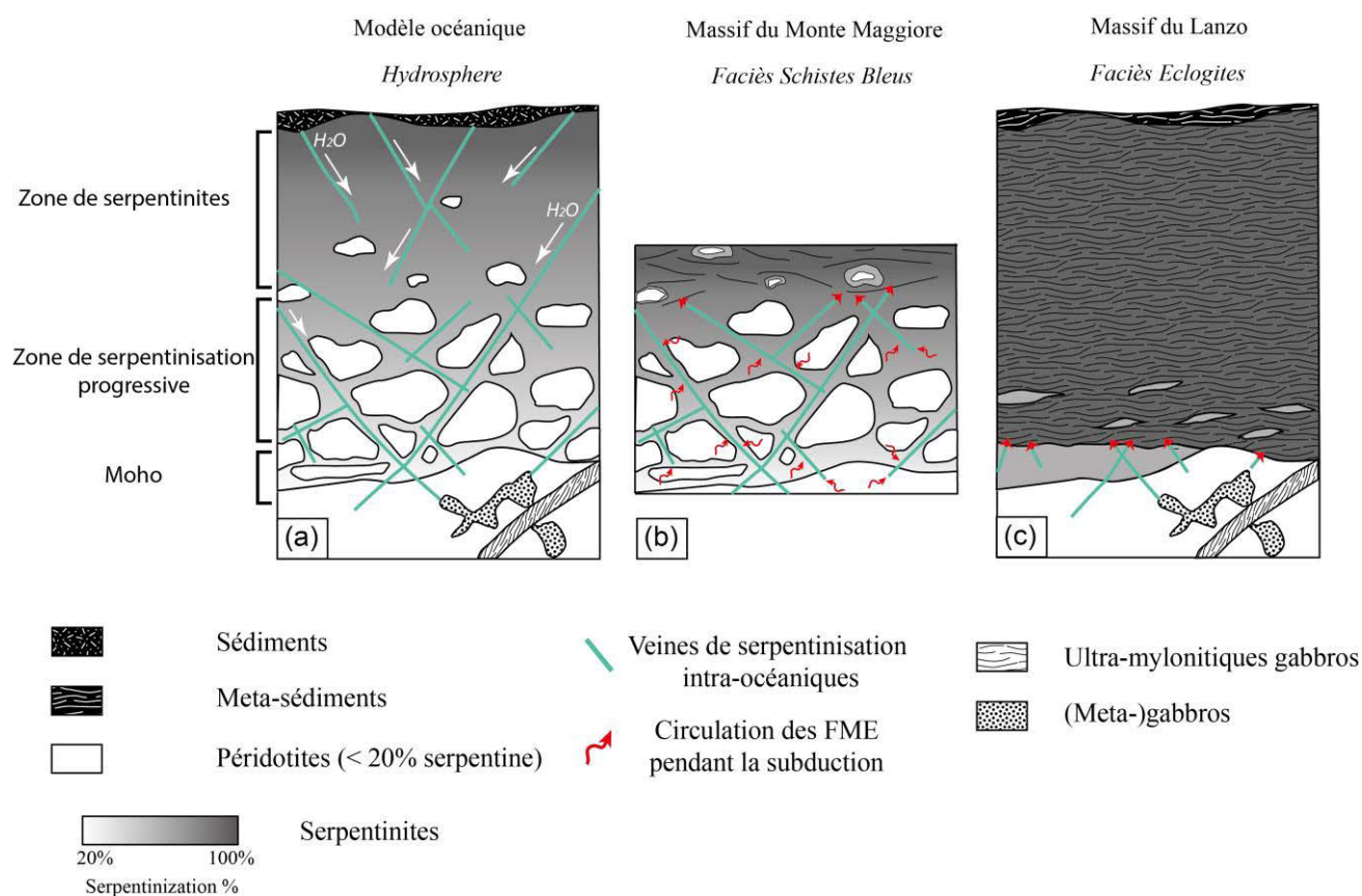
Figure IV.13 : Modèle du front de serpentinisation et du MOHO océanique comparé aux exemples alpins du Monte Maggiore et du Lanzo. Les représentations schématiques de la lithosphère sont basées (a) sur le modèle intra-océanique, sur les observations réalisées sur les ophiolites du (b) Monte Maggiore et du (c) Lanzo.
