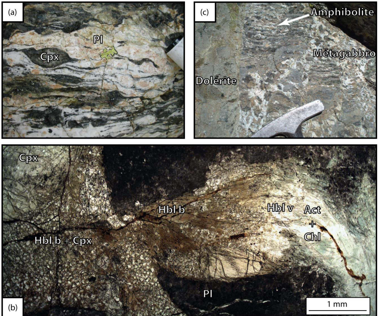
Figure II.11 : (a) Métagabbro folié présentant des porphyroclastes de clinopyroxène avec une couronne noire d'amphibole et une matrice blanche (site du plagioclase). (b) Photo en LPNA montrant les différents stades de recrystallisation du métagabbro. Le porphyroclaste de clinopyroxène est entouré d'une couronne de clinopyroxènes granoblastiques avec de la hornblende brune interstitielle. Le bord de la couronne est composé de cristaux de hornblende brune progressivement transformé en hornblende verte puis en un assemblage à actinote, chlorite et épidote en allant vers la bordure. Le site du plagioclase est composé d'un assemblage finement recrystallisé à épidote et albite. (c) Métagabbro contenant des enclaves d'amphibolite et recoupé par un filon de dolérite.
