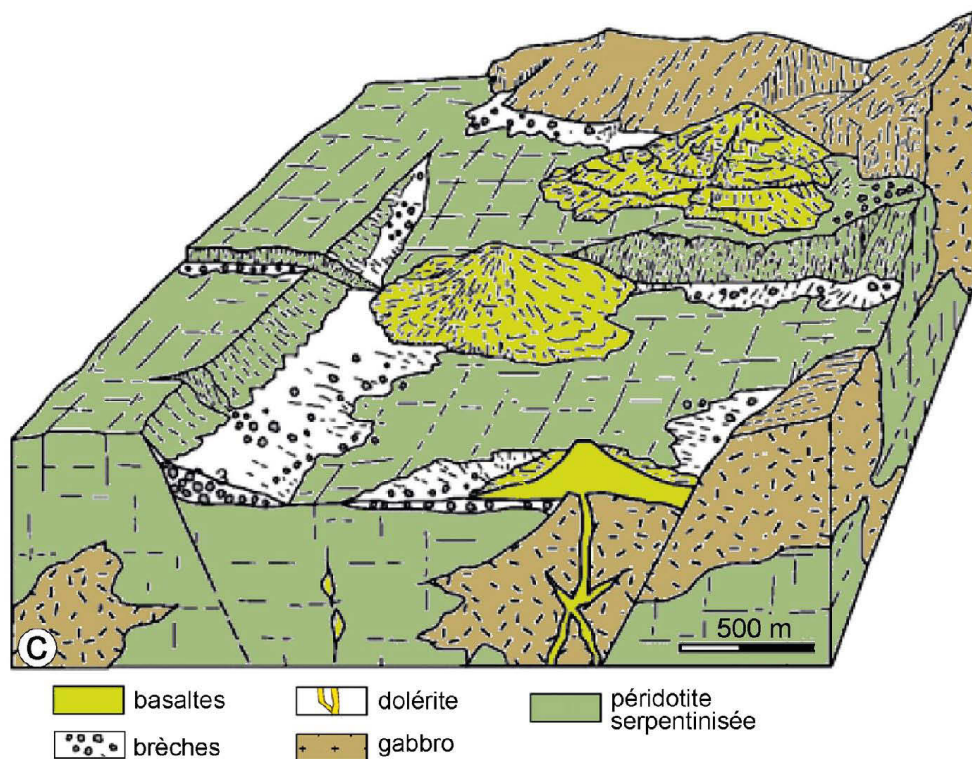
Figure I.7 : Reconstruction schématique des années 90 des parties superficielles de l'océan Ligure. Les formations magmatiques sont isolées et séparées par un manteau serpentinsé (Lagabrielle & Cannat, 1990).
