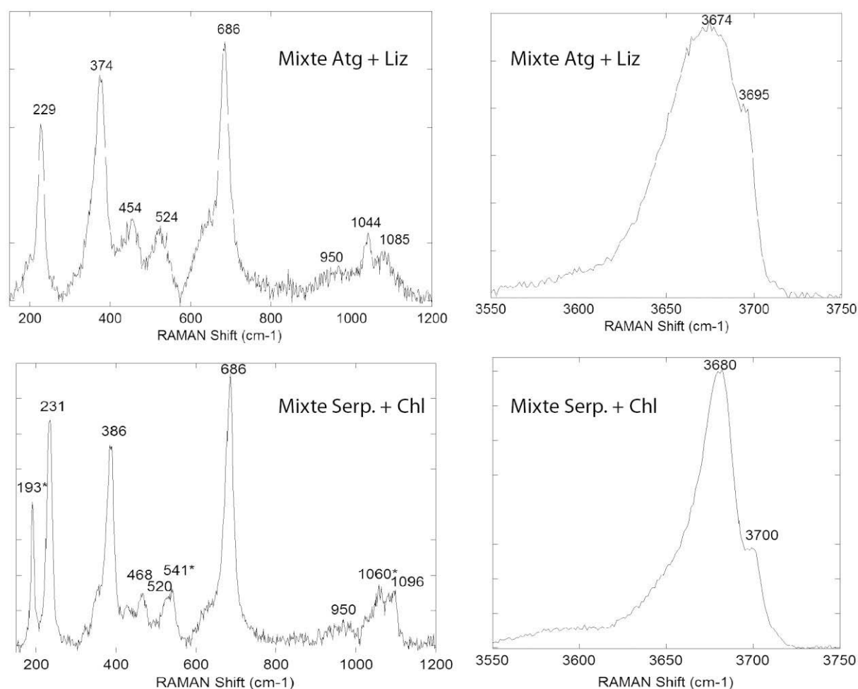
Figure IV.10 : Spectres RAMAN mixtes analysés dans les veines de serpentine et chlorite du Sud de la coupe de Germagnano. * pics correspondant à la chlorite.
