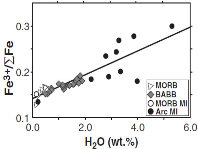
Figure 1.21 : Diagramme comparant la composition en Fe^{3+}/Fe^{Tot} et en H_2O des MORB et des laves d'arrière arc (BABB) et des inclusions magmatiques (MI) des MORB et des laves d'arc (Kelley & Cottrell, 2009).
