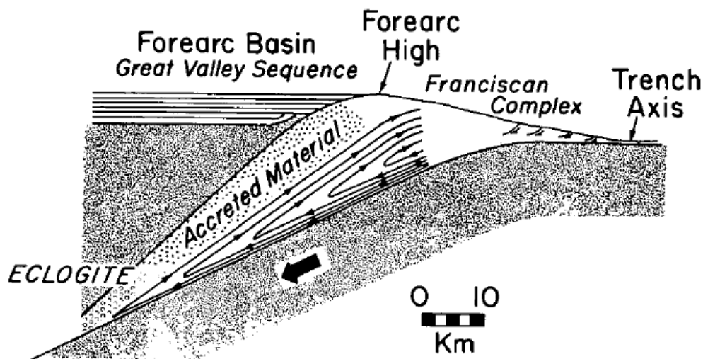
Figure I.8 : Schéma des années 80 illustrant la dynamique des flux de matière à l'intérieur du prisme d'accrétion (Cloos, 1982).
