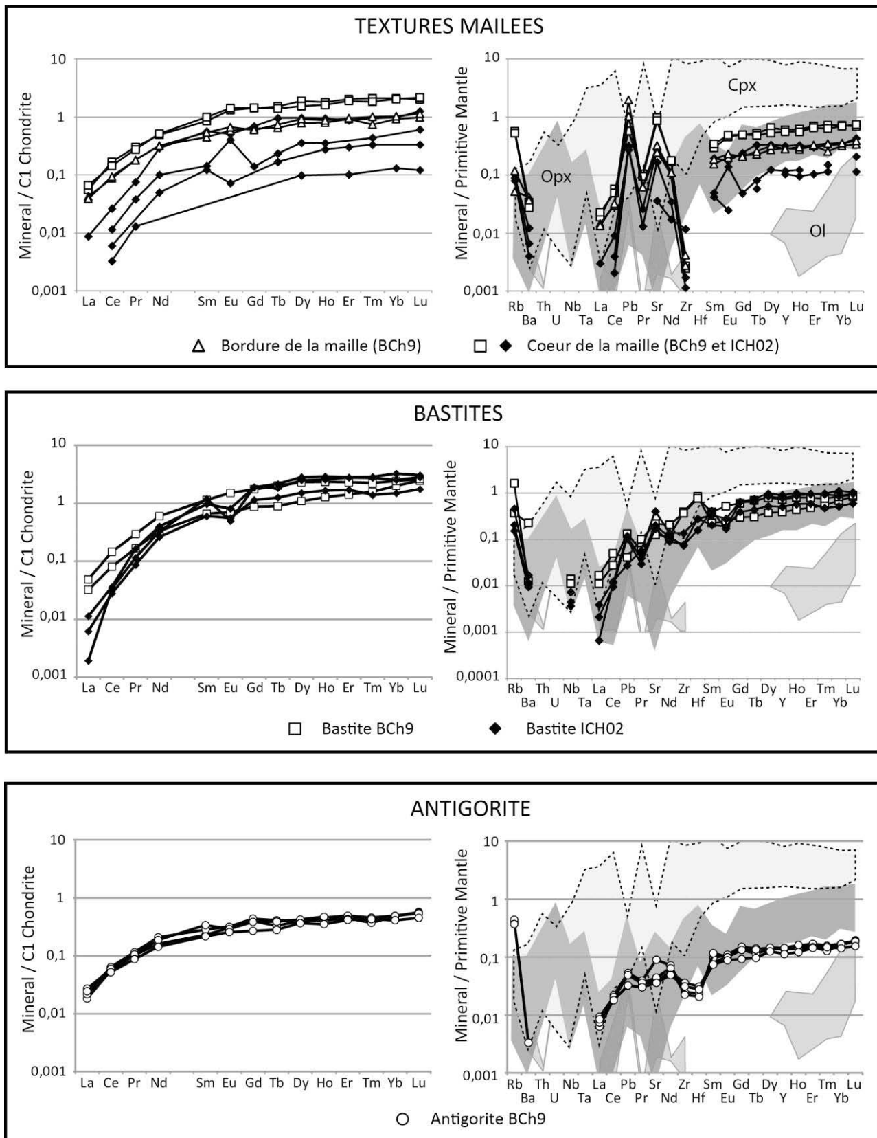
Figure II.16 : Spectres en REE et étendues aux éléments en trace des serpentines des échantillons BCh9 et ICH02 normalisés aux chondrites à gauche et au manteau primitif à droite (valeurs de Sun & McDonough, 1989). Les champs en gris dans les diagrammes de droite indiquent la composition des
