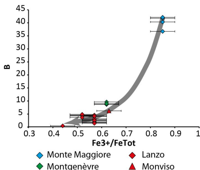
Figure VII.14 : Diagramme montrant la concentration des antigorites alpines en Bore en fonction de leur rapport \text{Fe}^{3+}/\text{Fe}^{\text{Tot}} .
