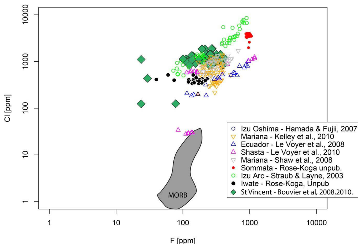
Figure VI.1 : Diagramme F vs Cl montrant les compositions des inclusions magmatiques primaires analysées dans des olivines. Les inclusions primaires analysées dans les basaltes d’arc ont des compositions en F et Cl plus élevées que les inclusions primaires des MORB (Champ gris).
