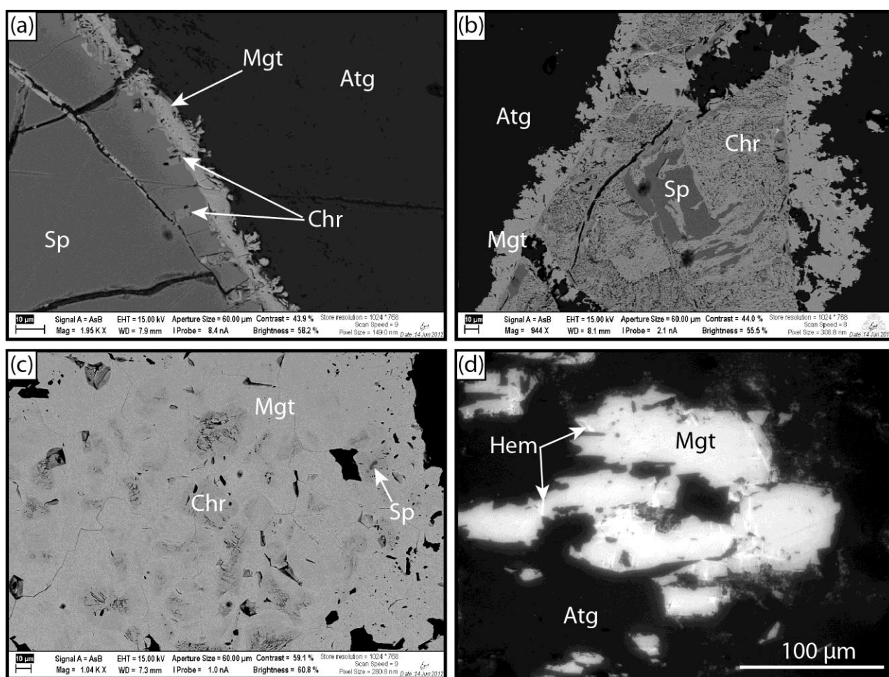
Figure VII.5 : Photographies BSE obtenues au MEB (a-c) et en lumière rétrodiffusée au microscope optique (d) des minéraux ferromagnésien associés à l'antigorite. Les photographies (a) à (c) permettent d'observer la recrystallisation progressive du spinelle mantellique en chromite et magnétite lors de la subduction. (a) Atg/Liz-serpentinite du Montgenèvre où le spinelle mantellique possède une fine couronne à chromite puis magnétite. (b) Atg/Liz-serpentinite du Monte Maggiore où le spinelle mantellique possède une épaisse couronne à chromite et magnétite. (c) Atg-serpentinite du Lanzo où le spinelle à quasi-disparu et où la magnétite est présente en plus grande quantité que la chromite. (d) Grains de magnétites associés à de l'antigorite dans une Atg-serpentinite du Lanzo. La magnétite est traversée par des baguettes d'hématite.
