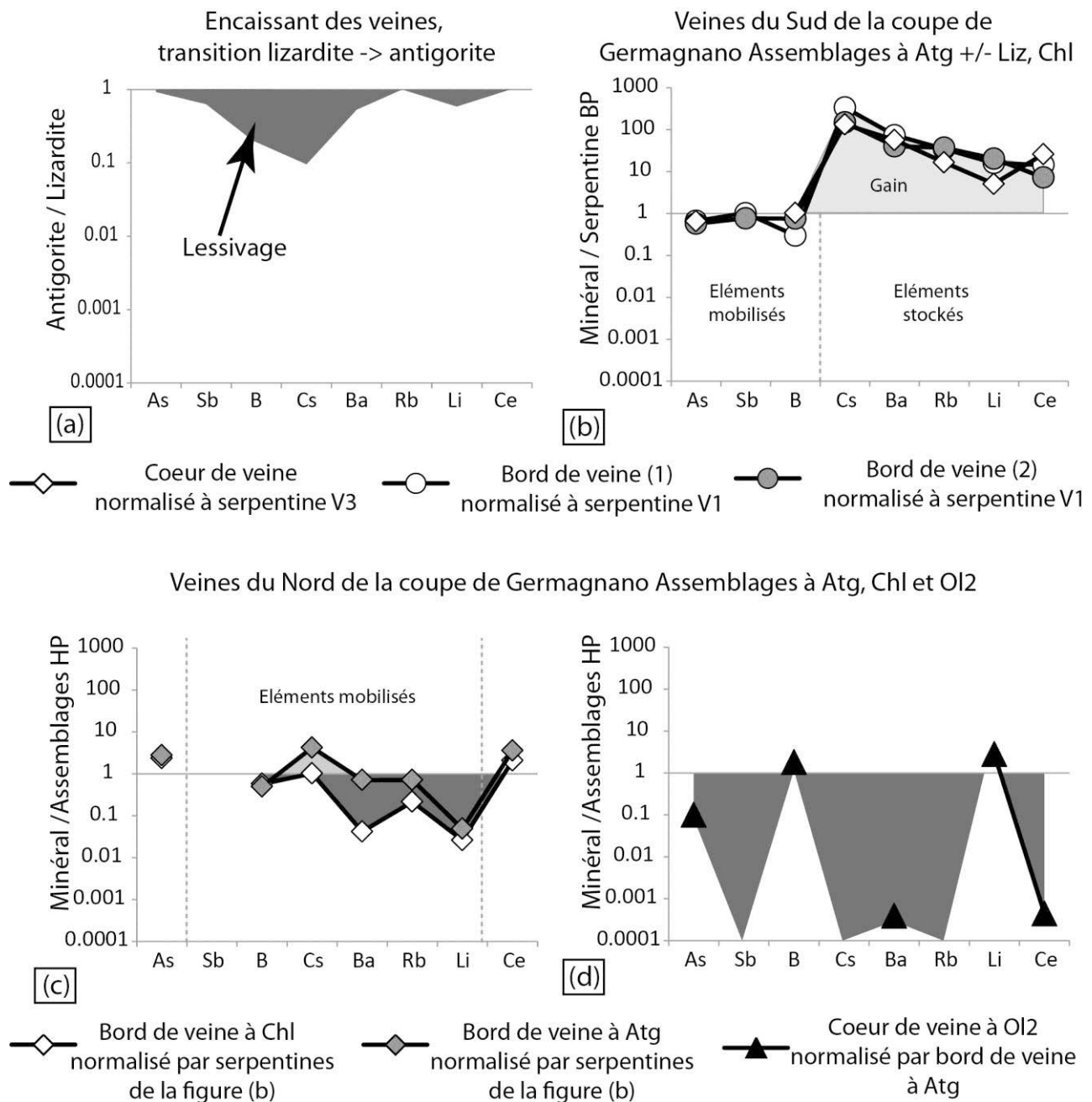
Figure IV.12 : Bilan élémentaire en FME lors des différentes transitions de phase de la serpentine dans (a) la péridotite peu serpentinisée et les veines métamorphiques au (b) Sud et au (c) Nord de la coupe de Germagnano. (a) Composition en FME de l'antigorite normalisée à celle de la lizardite. (b) Compositions des assemblages de HP des veines du Sud de la coupe de Germagnano normalisées aux serpentines de BP océaniques des veines de serpentinisation du Monte Maggiore (V1, V2 et V3). (c) Composition des antigorites et chlorites des veines du Nord de la coupe de Germagnano normalisés à la composition moyenne des assemblages de HP des veines du Sud de la coupe de Germagnano. (d) Composition moyenne des olivines de déserpentinisation normalisée à la composition des antigorites formant la bordure des veines du Nord de la coupe de Germagnano.
