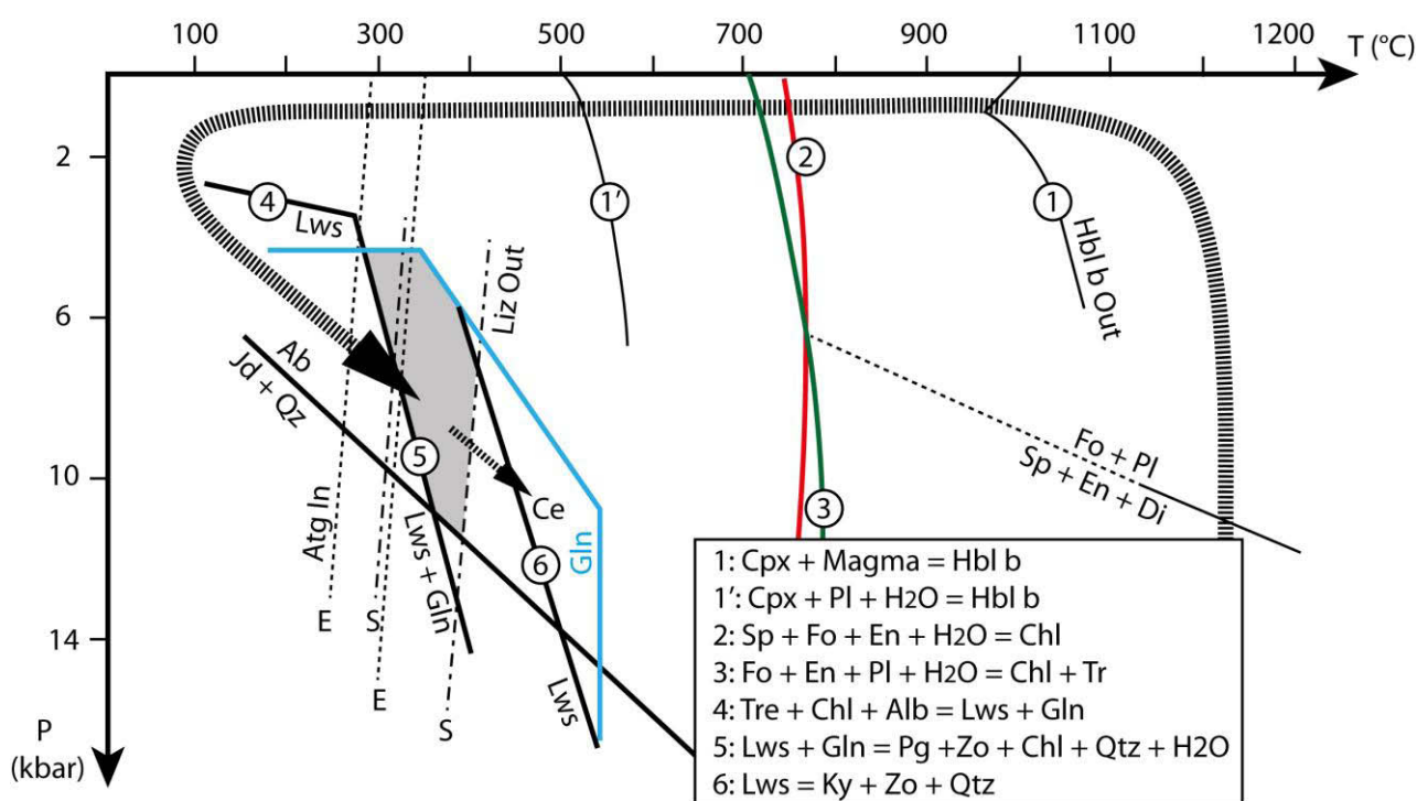
Figure III.19 : Chemin P-T du massif du Monte Maggiore. Lors du refroidissement intra-océanique, les gabbros cristallisent du clinopyroxène, du plagioclase, de l'olivine et éventuellement de la hornblende brune par réaction périclitique (Hbl B out). A plus BT, l'amphibole métamorphique croît jusqu'à des températures de 500°C. A partir de ~ 700°C, l'olivine est recristallisée en un assemblage à trémolite et chlorite en contact avec l'orthopyroxène et le plagioclase. Sur le chemin P-T, les conditions en pression et températures de la lithosphère lors de son refroidissement intra-océanique sont fixées arbitrairement. Celles-ci varient entre 5°C / 0.2-0.3 kb au niveau du plancher océanique et ~ 2 kb / ~ 350°C au niveau du Moho. Lors des premiers stades de la subduction, l'amphibole est transformée en glaucophane et le plagioclase est recristallisé en jadéite et zoisite. L'absence de lawsonite et de quartz permet de restreindre les conditions du pic de métamorphisme à un champ s'étalant de 300 à 400°C. Le pic en P-T du massif est compris dans le champ divariant de la transition lizardite vers antigorite. A l'opposé, dans l'ophiolite de Centuri (Ce), la lizardite est totalement recristallisée en antigorite suggérant que cette ophiolite a enregistré des conditions P-T de plus haut degré métamorphique. E et S : champs divariants de la transition lizardite vers antigorite d'après E : Evans et al. (2004) et S : Schwartz et al. (2013). 2, 3 : Nicollet et al. (2001) ; 4, 5 : Schmidt et Poli (1995) ; 1 et 1', 6 : Nicollet (2010).
