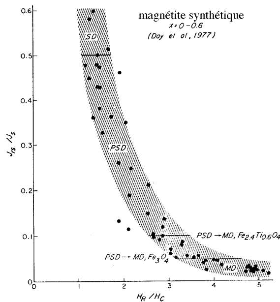
Figure VII.3 : Diagramme montrant la variation des rapports \mathbf{J}_{rs}/\mathbf{J}_s en fonction de \mathbf{H}_{cr}/\mathbf{H}_c (Day et al., 1977). Les grains de magnétite SD (single domaine) hébergent un seul domaine magnétique de petite taille égale à la taille du grain. Cette dernière est estimée entre 0.06 et 0.08 \mu\text{m} (Evans, 1972). Les grains PSD (Pseudo-Single Domain) ont des tailles variant de 0.08 à 15 \mu\text{m} (Dunlop & Özdemir, 1997). Les grains MD (Multi-Domains) sont divisés en différents domaines magnétiques séparés par une paroi appelée paroi de Bloch. Il s'agit de gros grain de taille allant de 15 \mu\text{m} à plusieurs millimètres.
