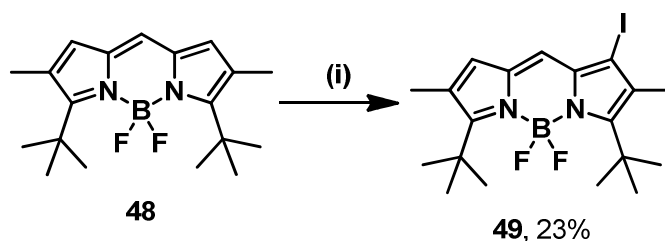
Figure 4.22 : Synthèse du composé 49 . (i) PIFA (0,3 équiv), \text{BF}_3\cdot\text{OEt}_2 (0,6 équiv), \text{CH}_2\text{Cl}_2 , -78 à 25\text{ }^\circ\text{C} , 2 h.
