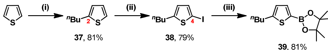
Figure 3.32 : Synthèse des composés 37 à 39 . (i) (a) n -BuLi (1,1 équiv), THF, -78 °C, 1 h ; (b) 1-bromobutane (1 équiv), 25 °C, 16 h ; (ii) HgO (1,1 équiv), I 2 (1,1 équiv), toluène, 0 °C, 4 h ; (iii) Pinacolborane (2 équiv), CuI (10% mol.), NaH (1,5 équiv), THF, 25 °C.
