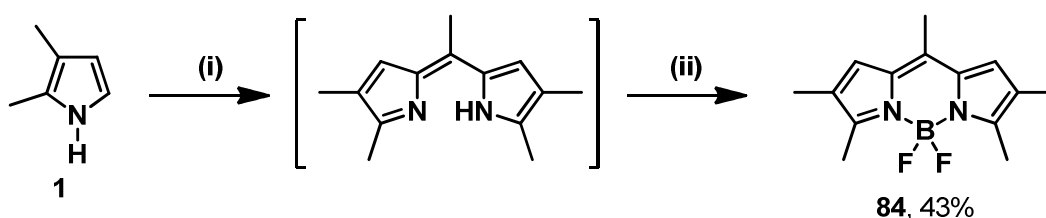
Figure 5.40 : Synthèse du composé 84 . (i) MeC(OEt) 3 (15 équiv), TFA (6 équiv), CH 2 Cl 2 , 25 °C, 1,5 h ; (ii) NEt 3 (6 équiv), BF 3 ·OEt 2 (8 équiv), CH 2 Cl 2 , 25 °C, 18 h.
