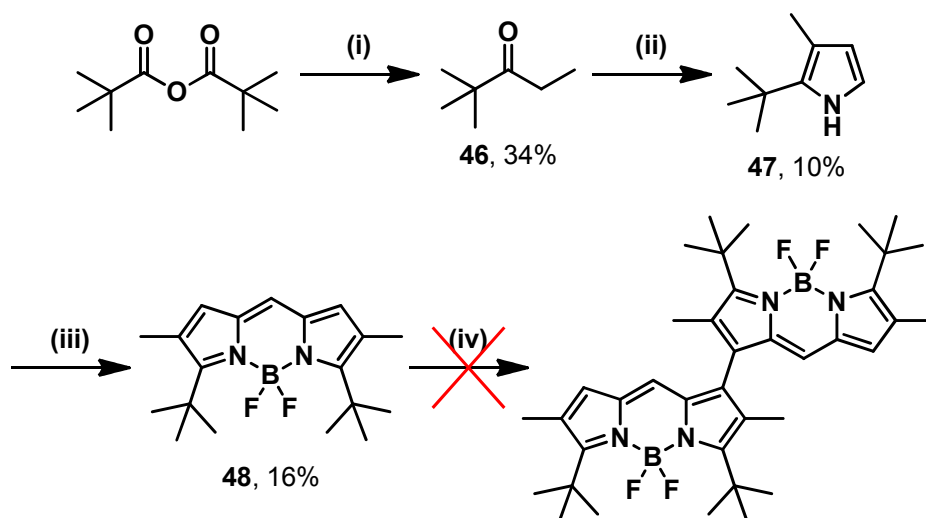
Figure 4.21 : Synthèse des composés 46 à 48 . (i) \text{EtMgCl} (0,7 équiv), THF, -40\text{ }^\circ\text{C} à 25\text{ }^\circ\text{C} , 18 h ; (ii) (a) \text{NH}_2\text{OH} , HCl (1 équiv), \text{NaHCO}_3 (1 équiv), DMSO, 25\text{ }^\circ\text{C} , 18 h ; (b) acétylène, 100\text{ }^\circ\text{C} , 30 min puis KOH (1,5 équiv), 5 h ; (iii) (a) \text{HC}(\text{OEt})_3 (15 équiv), TFA (6 équiv), \text{CH}_2\text{Cl}_2 , 25\text{ }^\circ\text{C} , 45 min ; (b) \text{NEt}_3 (6 équiv), \text{BF}_3\cdot\text{OEt}_2 (8 équiv), \text{C}_2\text{H}_4\text{Cl}_2 , 100\text{ }^\circ\text{C} , 2 jours ; (iv) PIFA (0,3 équiv), \text{BF}_3\cdot\text{OEt}_2 (0,6 équiv), \text{CH}_2\text{Cl}_2 , -78 à 25\text{ }^\circ\text{C} , 2 h.
