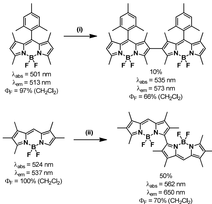
Figure 4.7 : Dimérisation de BODIPYs en positions 2 et 6 et en positions 3 et 5. (i) FeCl 3 (4 équiv), CH 2 Cl 2 , 25 °C, 25 min ; (ii) FeCl 3 (2 équiv), CH 2 Cl 2 , 0 °C, 1,5 min.
