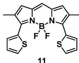
Figure 5.1 : Structure du 3,5-dithiényl-BODIPY 11 précédemment obtenu.
