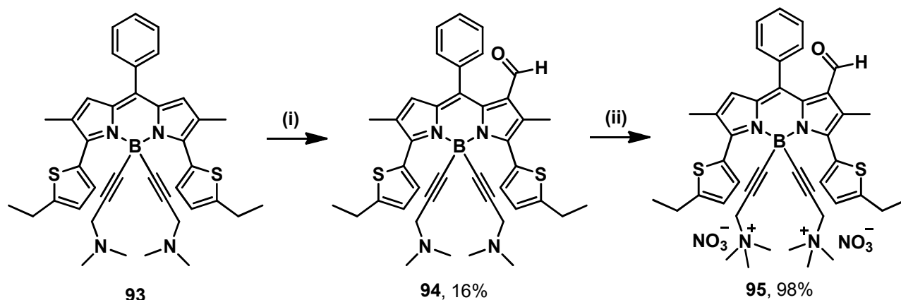
Figure 5.59 : Synthèse des composés 94 et 95 . (i) (a) \text{POCl}_3 (130 équiv), DMF, \text{C}_2\text{H}_4\text{Cl}_2 , 50 °C, 18 h ; (b) \text{NaHCO}_3 , 25 °C, 2 h ; (ii) (a) \text{CH}_3\text{I} (20 équiv), THF, 25 °C, 2 h ; (b) DOWEX 1×8-100.
