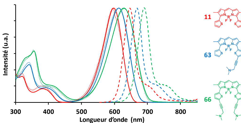
Figure 5.11 : Spectres d'absorption (trait plein), d'émission (tirets) et d'excitation (trait pointillé) pour les composés 11 (en rouge), 63 (en bleu) et 66 (en vert) à 25 °C dans CH 2 Cl 2 à \epsilon = 1 à 10 \times 10^{-5} M pour l'absorption, \epsilon = 1 à 10 \times 10^{-7} M pour l'émission ( \lambda_{\text{exc}} = 570 à 590 nm) et \epsilon = 1 à 10 \times 10^{-7} M pour l'excitation ( \lambda_{\text{em}} = 669 à 690 nm).
