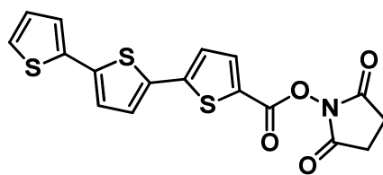
Figure 3.28 : Oligothiophène fonctionnalisé par l'ester N -succinimidyle.
