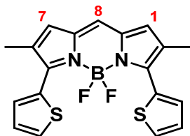
Figure 2.29 : Structure du 4,4'-difluoro-2,6-diméthyl-3,5-di-(thiényl-2-yl)-4-bora-3a,4a-diaza-s-indacène.
