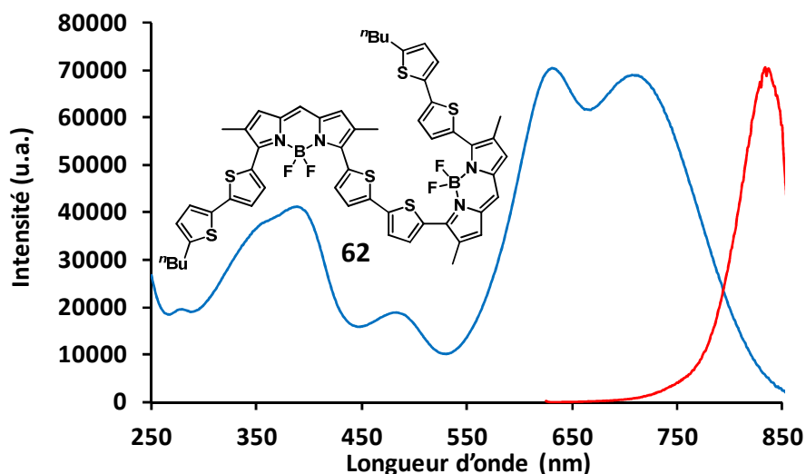
Figure 4.43 : Spectres d'absorption (en bleu) et d'émission (en rouge) pour le composé 62 à 25 °C dans \text{CH}_2\text{Cl}_2 à c = 2,16 \times 10^{-5}\text{ M} pour l'absorption et c = 2,16 \times 10^{-5}\text{ M} pour l'émission ( \lambda_{\text{exc}} = 620\text{ nm} ).
