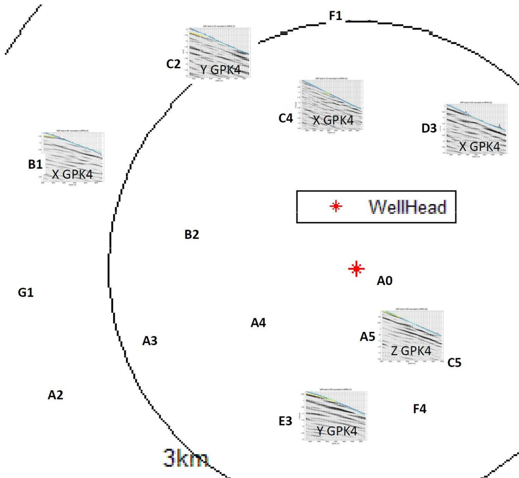
Figure 5.3.3: Ensemble des champs d'ondes réfléchies descendants extraits pour imager la structure sis1 . On utilise le puits GPK4.
