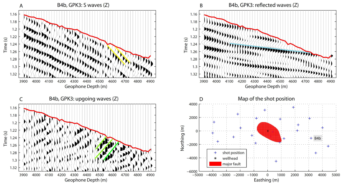
Figure 3.2.8: Différents champs d'onde extraits du tir B4b enregistré dans le puits GPK3, a : champ d'onde S descendant (conversion P-S = droite jaune), b : champ d'onde réfléchi (onde réfléchie = droite bleue claire), c : champ d'onde montant (onde montante = droite verte) et d : carte des positions de tir avec la faille majeure.
