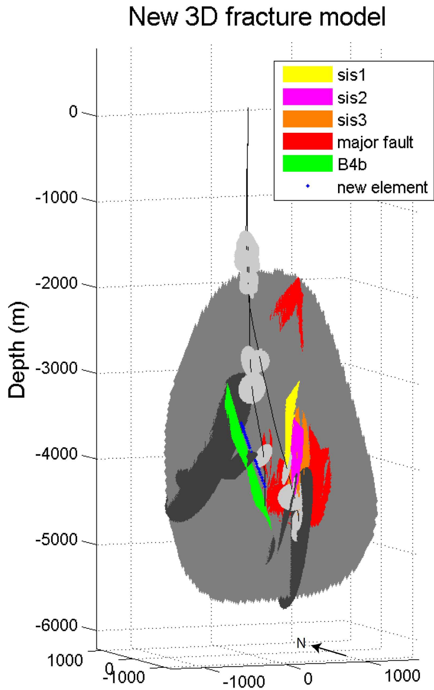
Figure 3.2.16: Modèle défini par Sausse et al. (2010) (noir et blanc) avec les structures issues des VSP (couleurs). On a le même code couleur que pour la figure 3.2.7.
