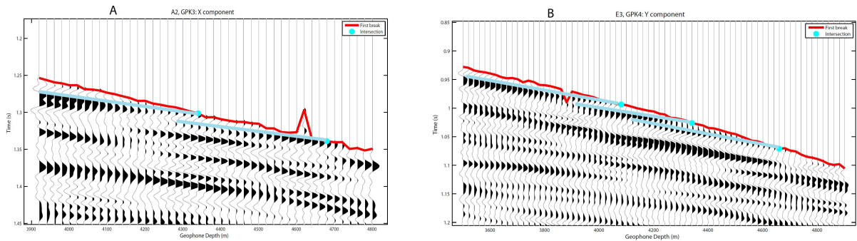
Figure 3.2.6: Intersection entre des arrivées réfléchies (droite bleue claire) et la première arrivée (droite rouge), a : champ réfléchi pour le tir A2 enregistré dans GPK3 sur une composante horizontale et b : champ réfléchi pour le tir E3 enregistré dans GPK4 sur l'autre composante horizontale.
