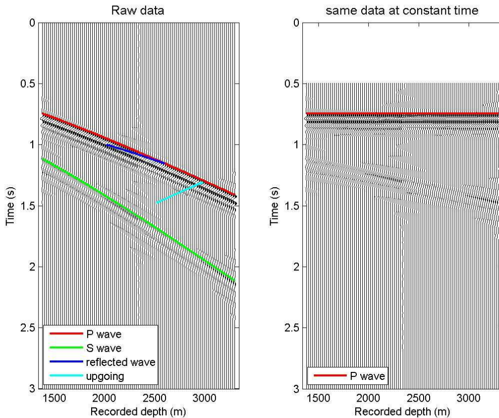
Figure 2.2.1: Données synthétiques sans bruits contenant les champs descendant P (ligne rouge) et S (ligne verte) et deux arrivées réfléchies (lignes bleues). Lorsque l'on aligne la première arrivée, les autres arrivées gardent bien un décalage en temps le long des traces.
