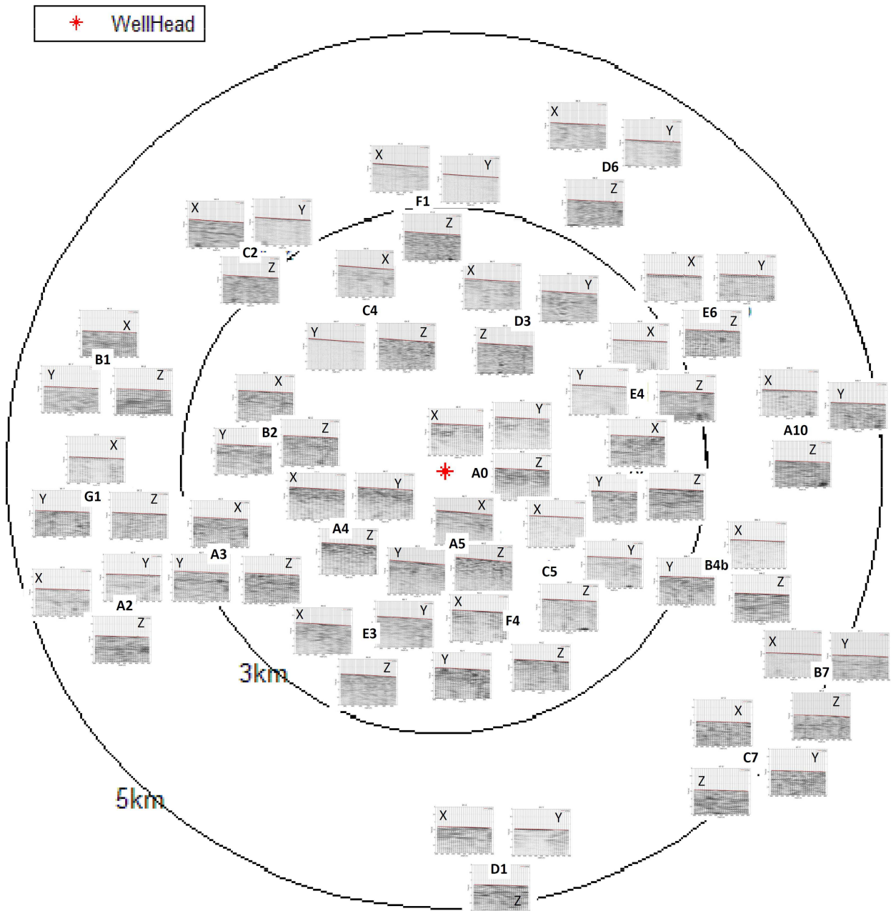
Figure 5.2.1: Ensemble des champs d'ondes P descendants extraits des enregistrements du puits GPK3.
