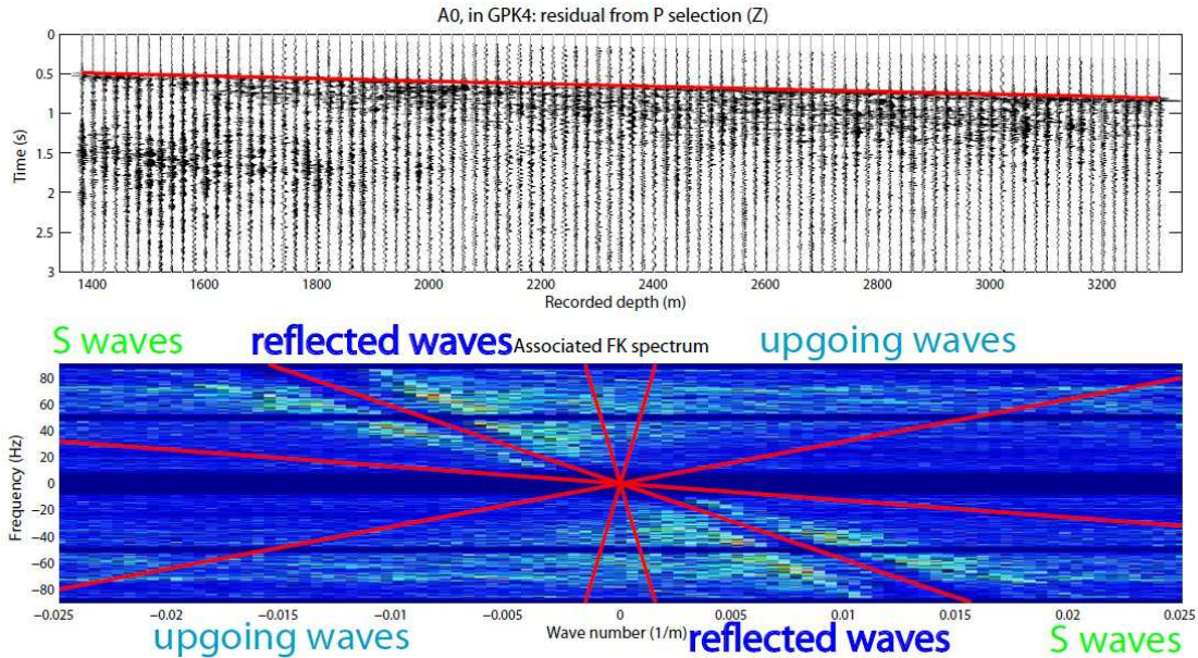
Figure 2.3.6: Résidu de l'extraction des ondes P pour le tir A0 enregistré dans le puits GPK4 avec son spectre FK associé.
