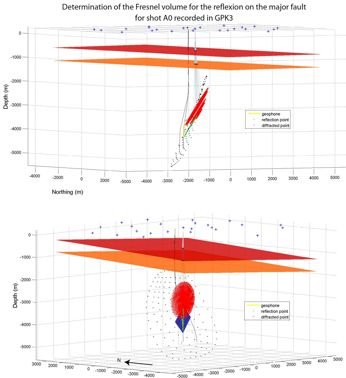
Figure 3.3.7: Volume de Fresnel pour un seul rai réfléchi de la réflexion sur la faille majeure pour le tir A0 enregistré dans GPK3. Le volume de Fresnel pour un rai englobe tous les points de réflexion extraits et également son épaisseur est du même ordre de grandeur ( \sim 100\text{m} ) que le volume total des réflexions extraites des VSP.
