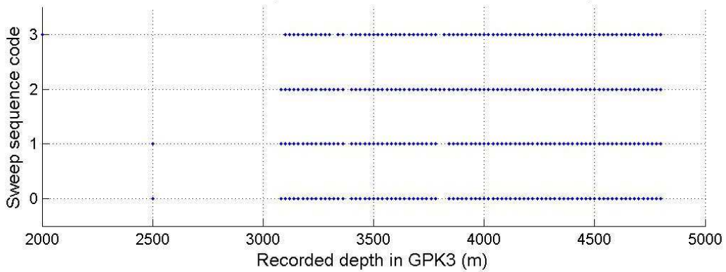
Figure 1.2.4: Profondeurs d'enregistrement en fonction de la séquence de tir pour le couple A0-E4 enregistré dans GPK3.
