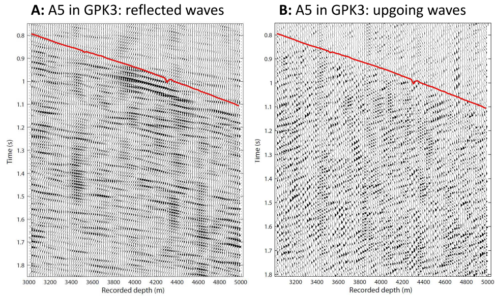
Figure 2.3.9: Décomposition du tir A5 enregistré dans le puits GPK3 sur la composante horizontale X avec les spectres FK associés, a : champ d'onde descendant réfléchi, zoom sur la première arrivée et d : champ d'onde montant, zoom sur la première arrivée.
