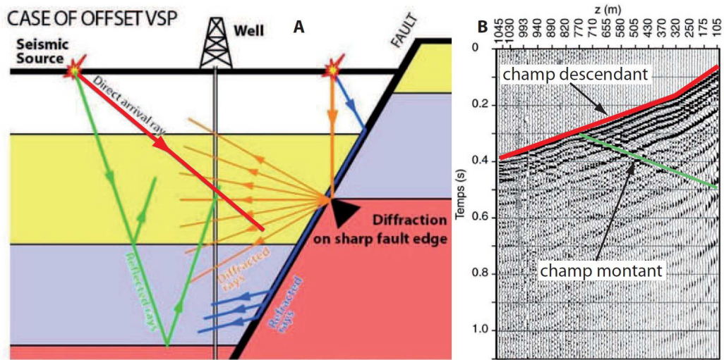
Figure 1.1.2: a : Principe d'une campagne de VSP avec un offset entre la source et la tête du puits d'enregistrement avec les principaux champs d'ondes étudiés. b : Exemple d'enregistrement de VSP avec le champ descendant associé à l'arrivée directe et le champ montant associé aux réflexions dans le milieu (document Gaz de France).
