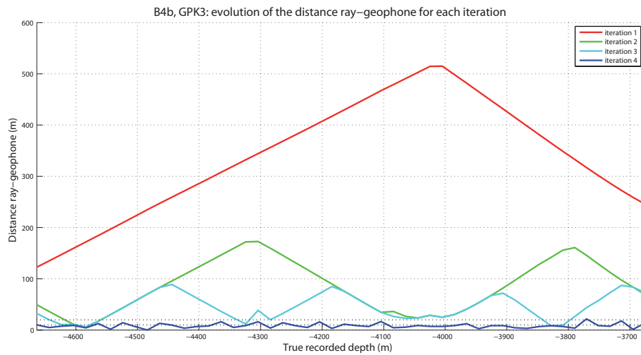
Figure 3.1.15: Écart entre les géophones et les rais sélectionnés pour le tir B4b enregistré dans le puits GPK3 pour les quatre itérations dans le cas d'une interface au socle non plane.
