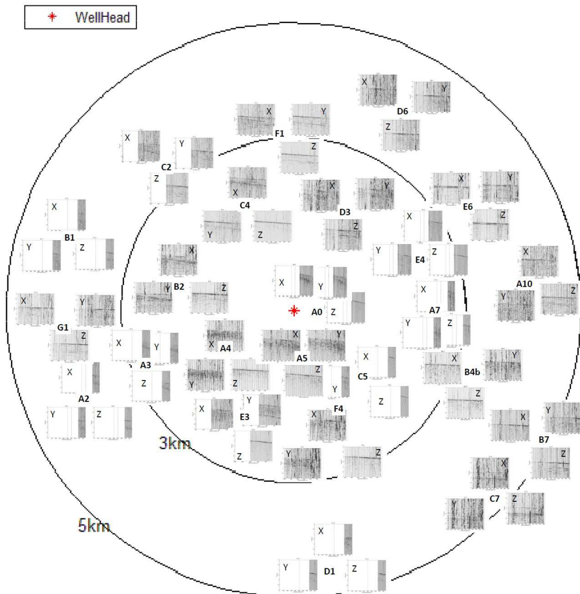
Figure 1.2.8: Ensemble des VSP normalisés enregistrés dans le puits GPK3 obtenus après corrélation, sommation et filtrage à 50Hz.
