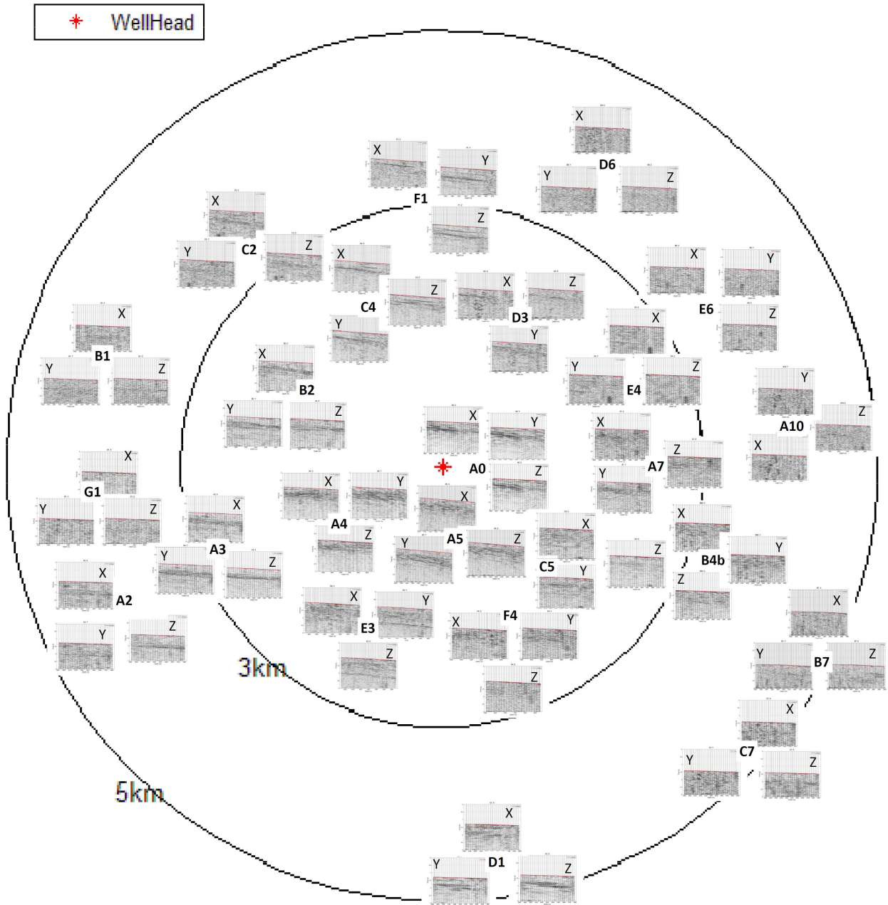
Figure 5.2.3: Ensemble des champs d'ondes S descendants extraits des enregistrements du puits GPK3.
