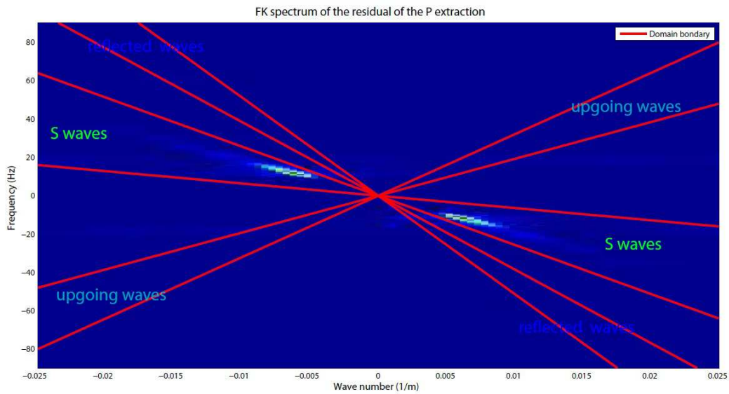
Figure 2.3.2: Spectre FK du résidu de l'extraction des ondes P avec les différents domaines de vitesse associés aux ondes S, réfléchies descendantes et montantes.
