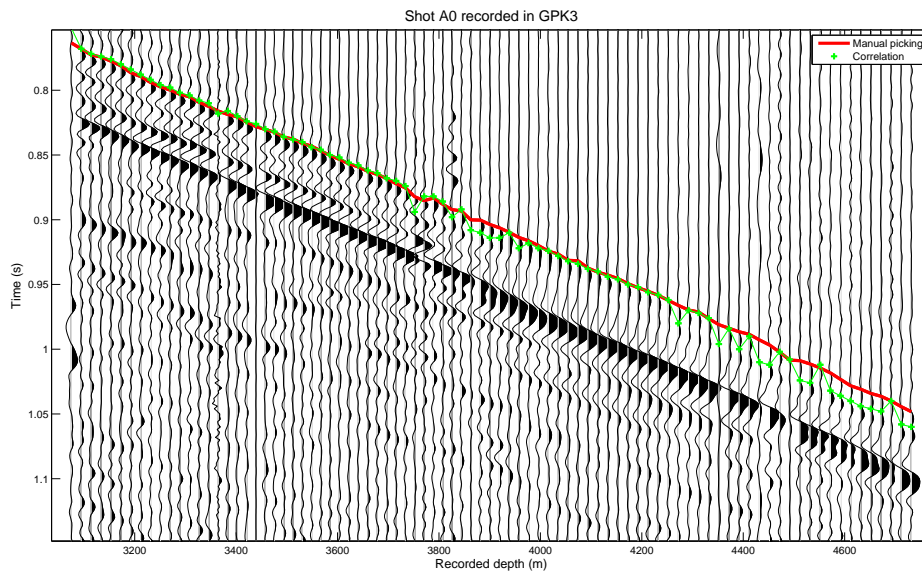
Figure 2.2.3: Tir A0 enregistré dans le puits GPK3. Le pointé manuel est représenté par la ligne rouge et le pointé par corrélation avec la source est représenté par les croix vertes.
