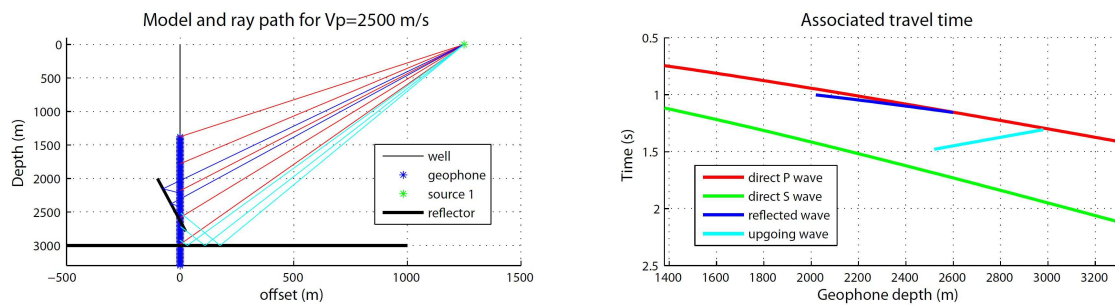
Figure 2.1.2: Modèle 1D avec une vitesse constante de 2500\text{m}\cdot\text{s}^{-1} avec les tracés de rais associés aux différents types d'onde enregistrés. Le graphique de droite représente les temps de trajet associés.
