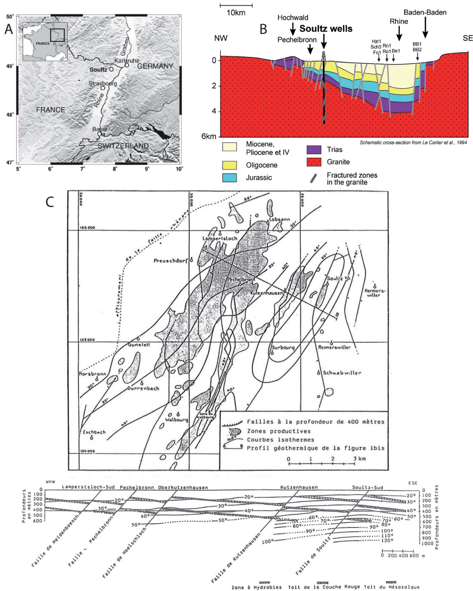
Figure 0.1.1: a : Localisation du site géothermique de Soutz-sous-Forêts, b : coupe NO-SE schématique du fossé rhénan (Le Carlier et al., 1994) passant par le site géothermique et c : Carte des isothermes à la profondeur de 400 m et profil thermique correspondant à la ligne AB (Gérard et al., 1984).
