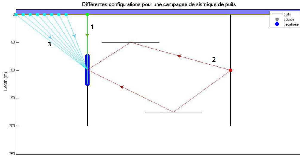
Figure 1.1.1: Différentes configurations pour une campagne de sismique de puits. Trajet 1 : VSP à départ nul, Trajet 2 : Profil puits à puits, Trajet 3 : VSP avec offset, dans le cas d'une ballade sismique.
