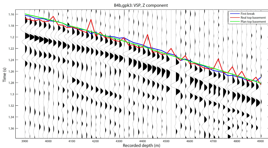
Figure 3.1.16: Comparaison des temps modélisés avec le modèle non plan (courbe rouge) et plan (courbe verte) et avec le pointé de la première arrivée pour le tir B4b enregistré dans le puits GPK3, zoom sur la première arrivée après correction statique.
