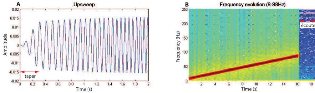
Figure 1.1.3: Sweep de 16 secondes plus trois seconde d'écoute dont la fréquence instantanée varie entre 8 et 88Hz. a : 2 premières secondes du sweep en temps, b : évolution de la fréquence instantanée sur les 19 secondes du signal.
