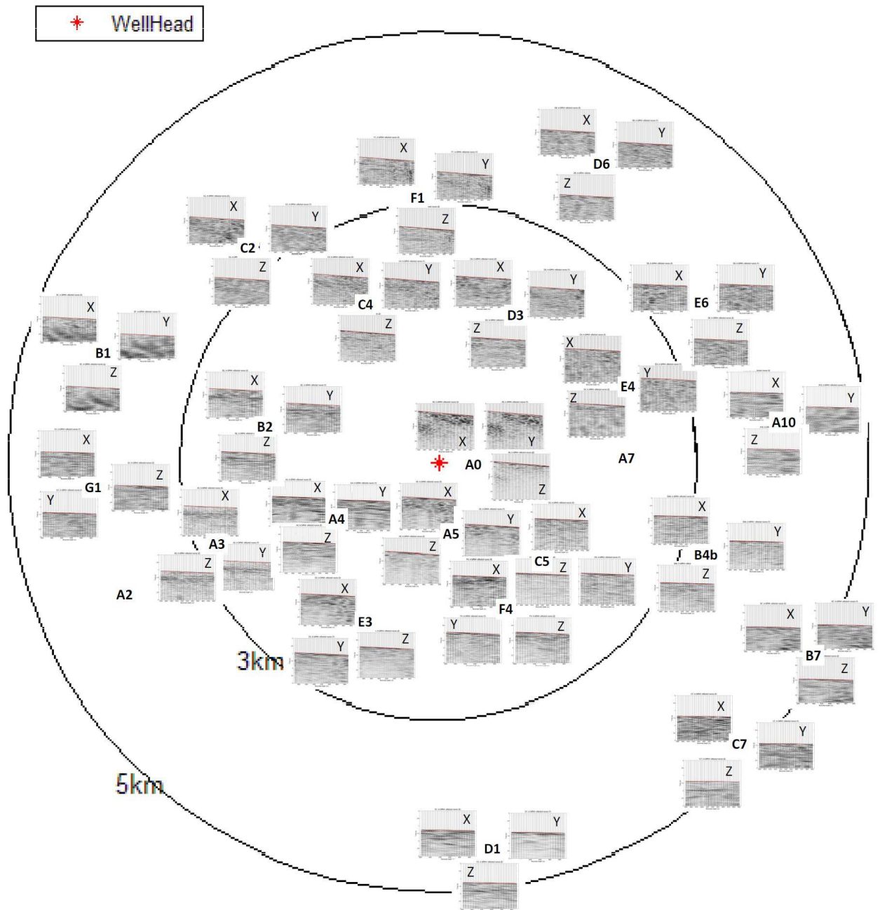
Figure 5.2.8: Ensemble des champs d'ondes réfléchies descendants extraits des enregistrements du puits GPK 4 . Les données pour des temps inférieurs à la première arrivée (ligne rouge) sont mises à zero
