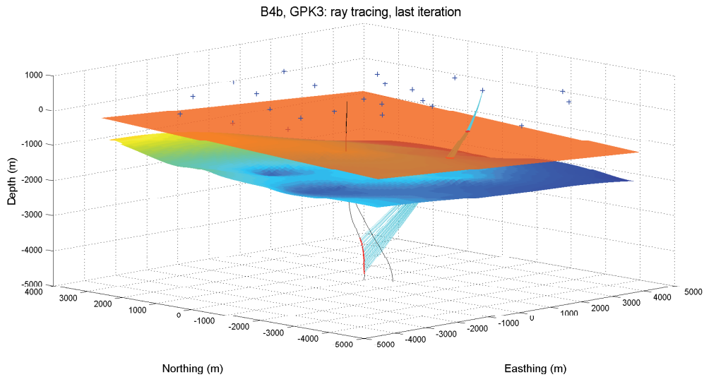
Figure 3.1.14: Tracé de rai pour le tir B4b enregistré dans le puits GPK3 avec le toit du socle non plan.
