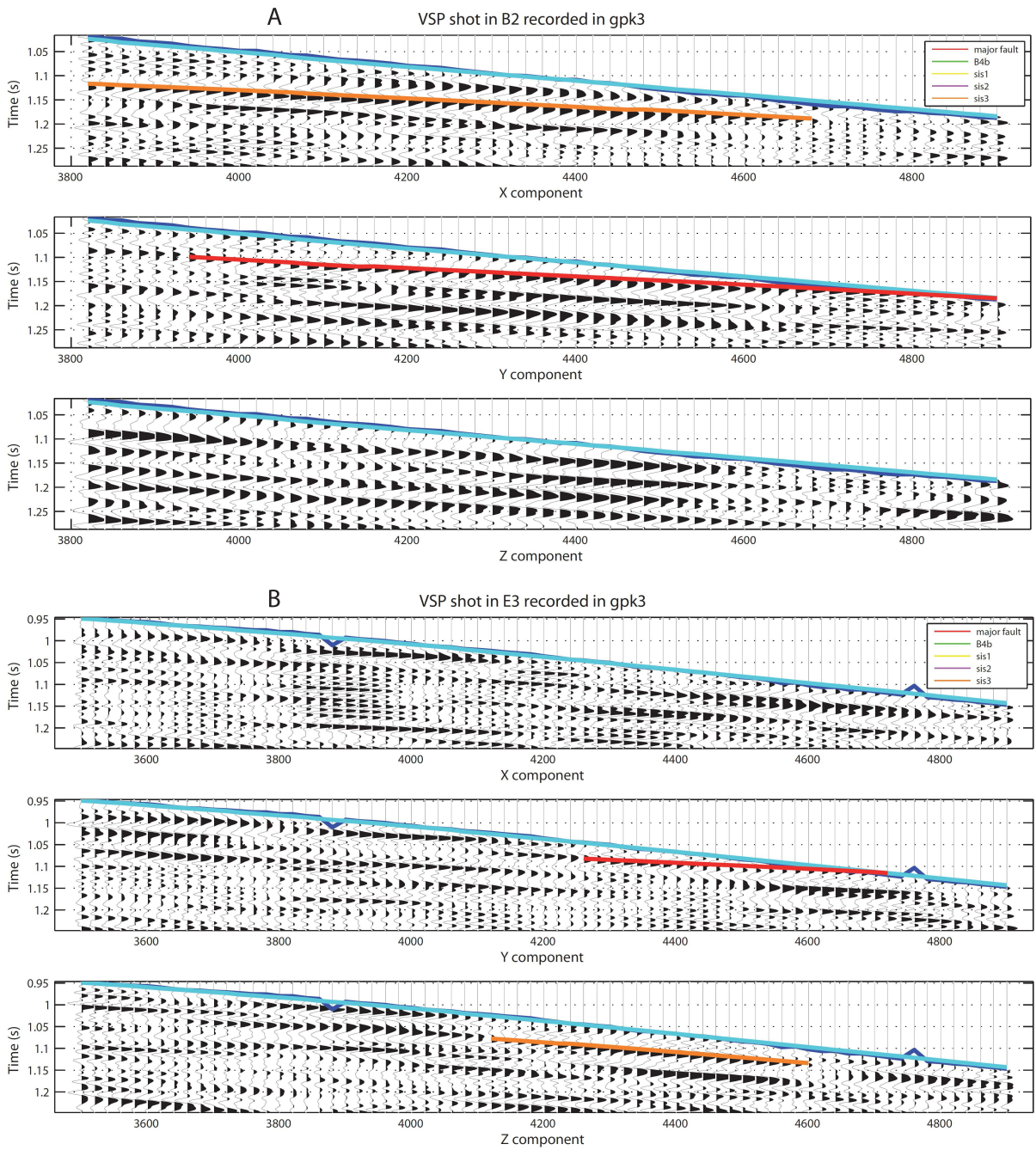
Figure 3.2.11: Temps de trajet modélisés pour les différents réflecteurs modélisés qui correspondent à des arrivées réfléchies observées sur les trois composantes des géophones, a : tir B2 enregistré dans le puits GPK3 et b : tir E3 enregistré dans le puits GPK3. Le code couleur pour les différentes structures est celui de la figure 3.2.7.
