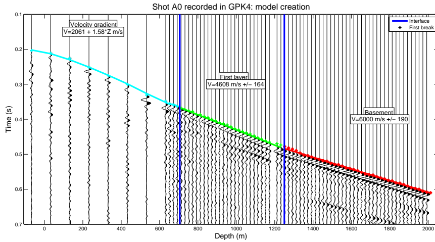
Figure 3.1.4: Tir A0 enregistré dans le puits GPK4 sur la composante verticale. Les trois sections du VSP correspondent à un gradient de vitesse (bleu clair), une couche sédimentaire homogène (vert) et au socle granitique homogène (rouge).
