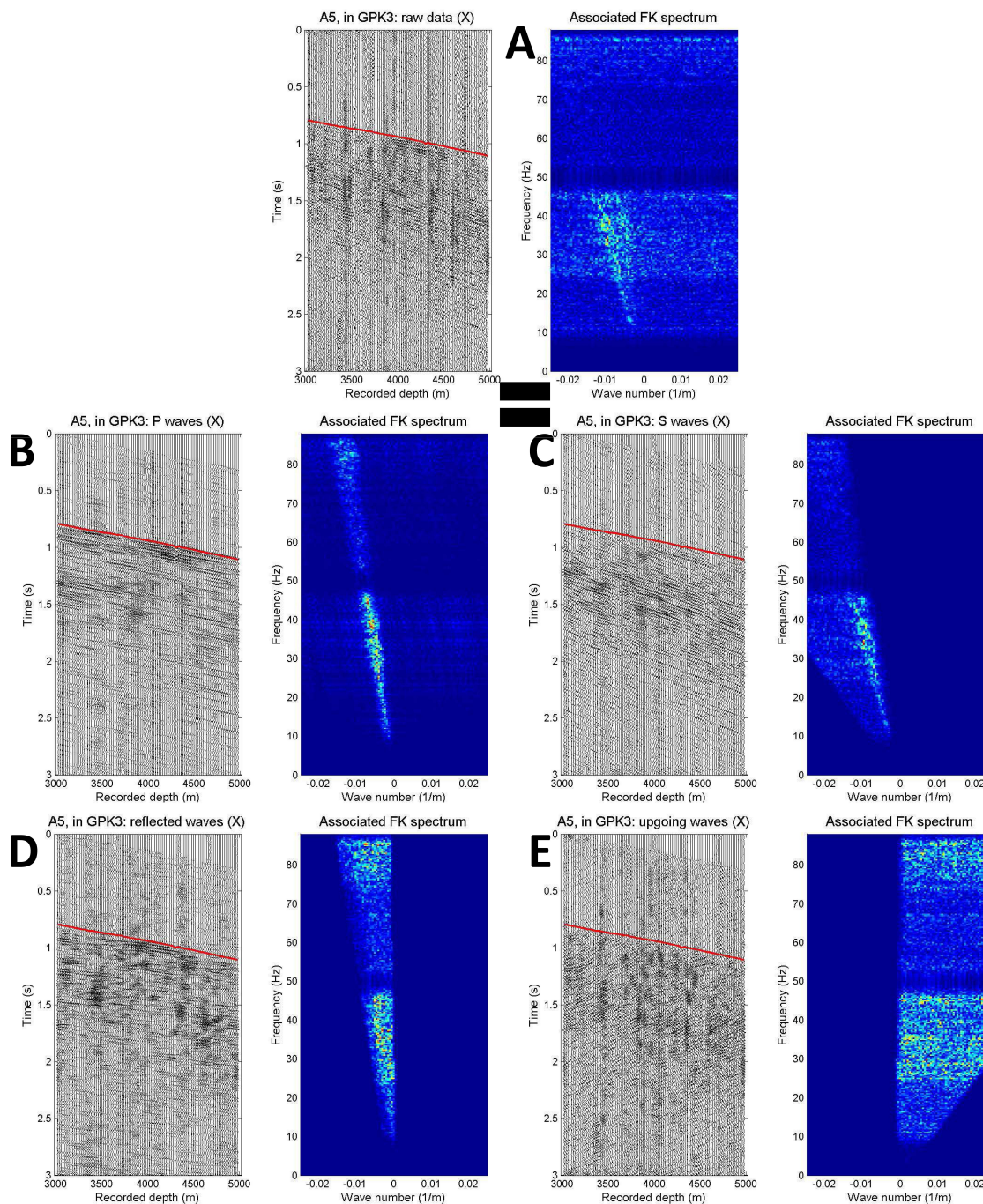
Figure 2.3.7: Décomposition du tir A5 enregistré dans le puits GPK3 sur la composante horizontale X avec les spectres FK associés, a : VSP brut, b : champ d'onde P descendant, c : champ d'onde S descendant, d : champ d'onde descendant réfléchi et e : champ d'onde montant. On a a = b + c + d + e .
