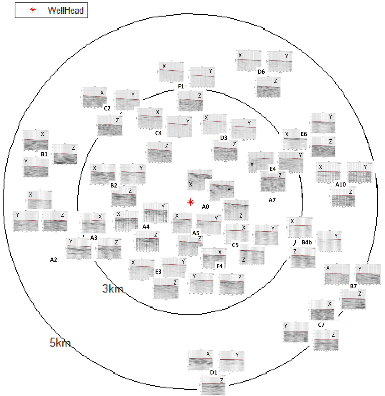
Figure 5.2.2: Ensemble des champs d'ondes P descendants extraits des enregistrements du puits GPK4.
