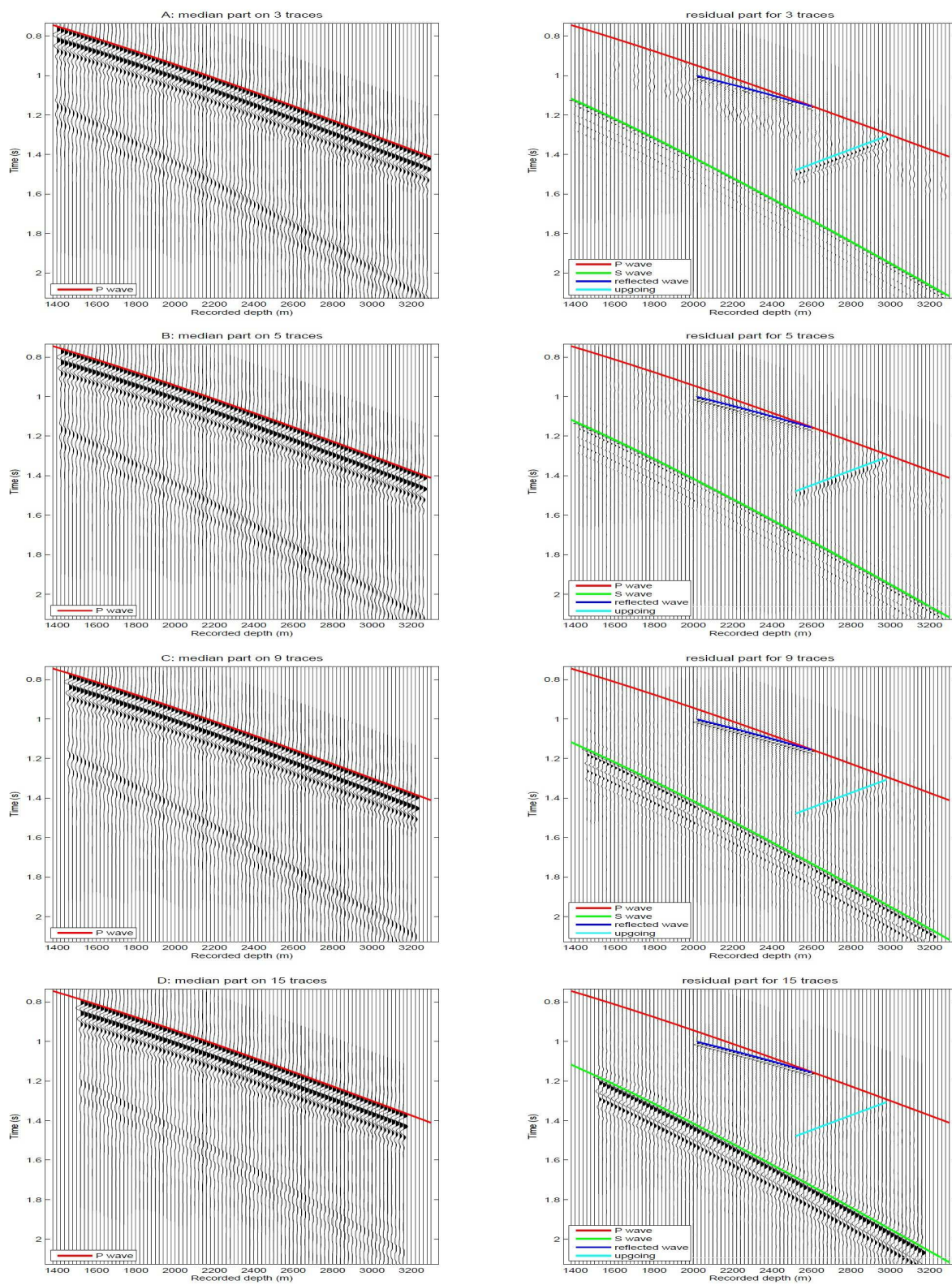
Figure 2.2.2: Partie médiane et résidu du filtrage médian après déhorizontalisation des données synthétiques. Nombre de traces de la fenêtre mobile, a : 3, b : 5, c : 9 et b : 15.
