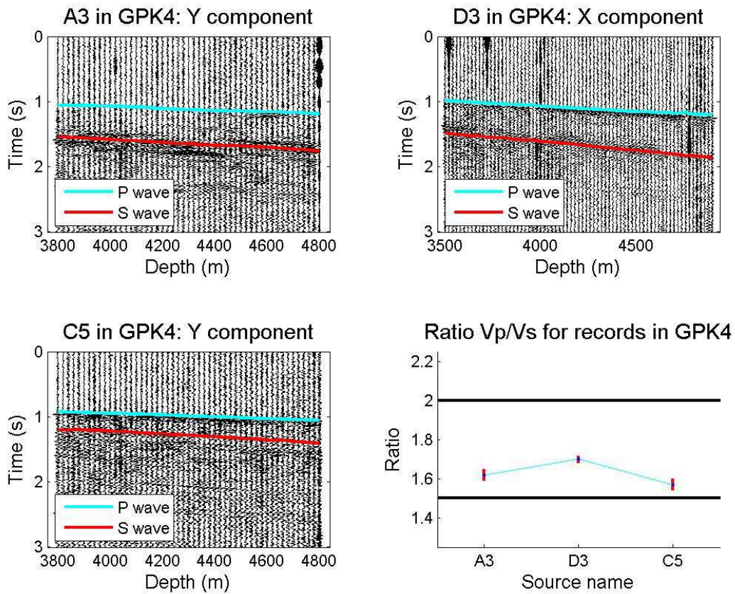
Figure 1.2.12: VSP A3 (composante Y), D3 (composante X) et C5 (composante Y) enregistrés dans le puits GPK4 avec les pentes des arrivées P et S, et le rapport V_p/V_s associé.
