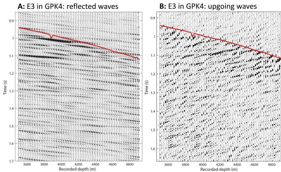
Figure 2.3.10: Décomposition du tir E3 enregistré dans le puits GPK4 sur la composante horizontale X avec les spectres FK associés, a : champ d'onde descendant réfléchi, zoom sur la première arrivée et d : champ d'onde montant, zoom sur la première arrivée.
