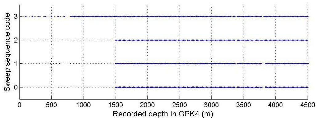
Figure 1.1.12: Profondeur d'enregistrement des 4 séquences de tir pour le couple de sources A0-E4 enregistré dans GPK4.
