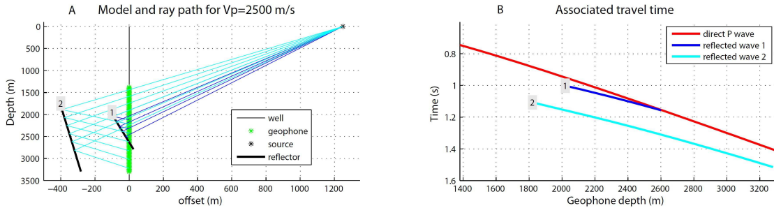
Figure 3.2.5: a : Tracé de rai des réflexions sur la faille 1 de pendage 81^\circ et la faille 2 de pendage 85.5^\circ dans un milieu homogène de vitesse 2500\text{m}\cdot\text{s}^{-1} , b : temps de trajet associés (courbe bleue foncée : faille 1, courbe bleue claire : faille 2) avec la première arrivée (courbe rouge).
