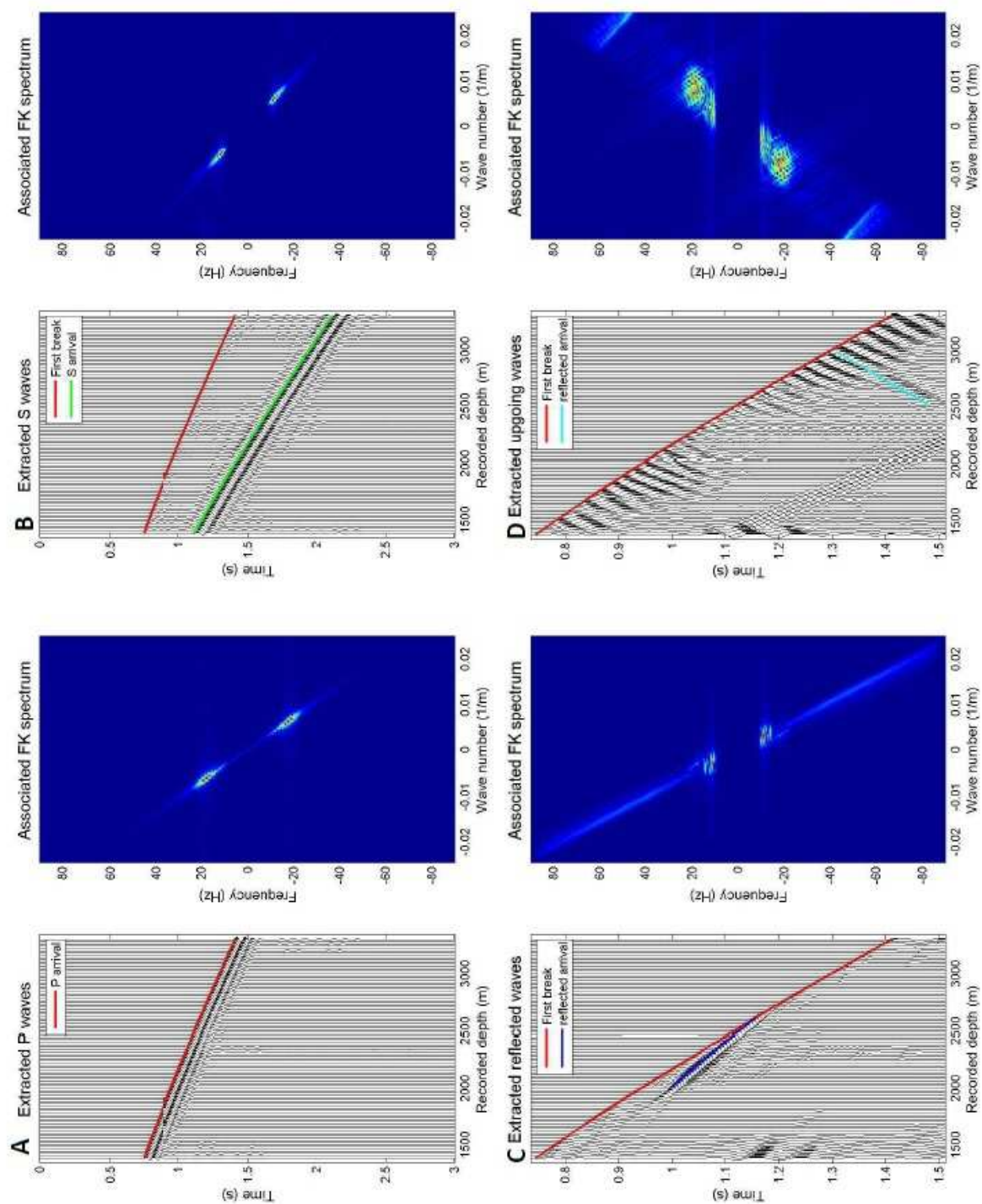
Figure 2.3.3: Résultats du filtrage FK, a : ondes P, b : ondes S, c : ondes réfléchies et d : ondes montantes.
