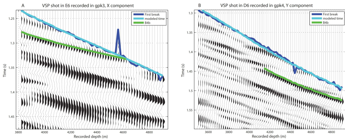
Figure 3.2.13: Arrivée réfléchie modélisée pour la structure B4b correspondant à des arrivées observées dans le champ réfléchi, a : tir E6 enregistré dans GPK3 enregistré sur une composante horizontale et b : tir D3 enregistré dans GPK4 enregistré sur la même composante horizontale.
