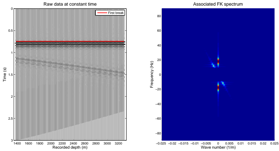
Figure 2.3.1: Données synthétiques horizontalisées et spectre FK associé. La première arrivée présente une vitesse apparente infinie.
