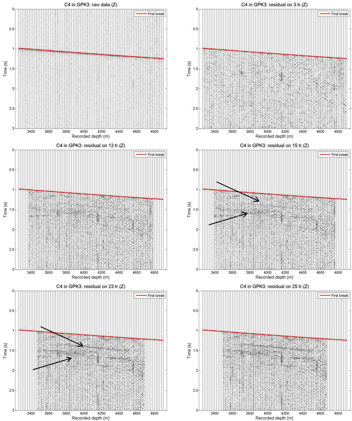
Figure 2.2.5: Filtrage médian du tir C_4 enregistré dans GPK3 sur la composante verticale avec des fenêtres mobiles comportant de 3, 13, 15, 23 et 25 traces. Les données ont été mises à zéro pour t < t_{pick} . Les flèches noires représentent le champ d'onde S descendant invisible initialement.
