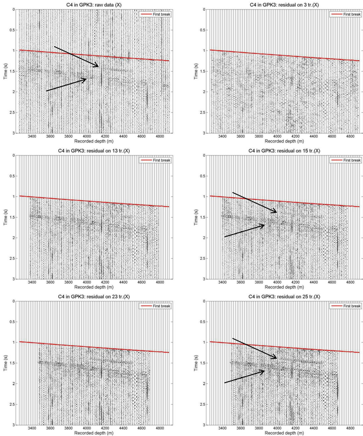
Figure 2.2.4: Filtrage médian du tir C4 enregistré dans GPK3 sur la composante horizontale X avec des fenêtres mobiles comportant de 3, 13, 15, 23 et 25 traces. Les données ont été mises à zéro pour t < t_{pick} . Les flèches noires représentent le champ d'onde S descendant.
