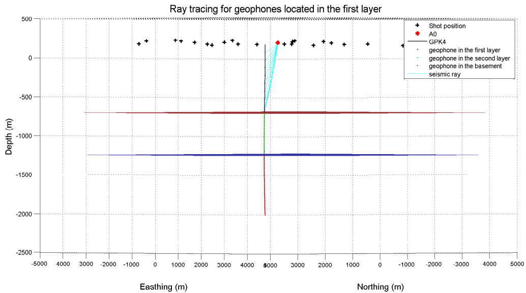
Figure 3.1.5: Tracé de rai pour le gradient de vitesse pour le tir A0 enregistré dans le puits GPK4. Le code couleur est le même que pour la figure 3.1.4. Le bloc 3D est vu à l'horizontale depuis le sud-est.
