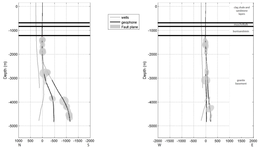
Figure 3.2.1: Plans de fractures à proximité des puits GPK3 et GPK4 à partir d'imagerie de puits, vue nord-sud et ouest-est.
