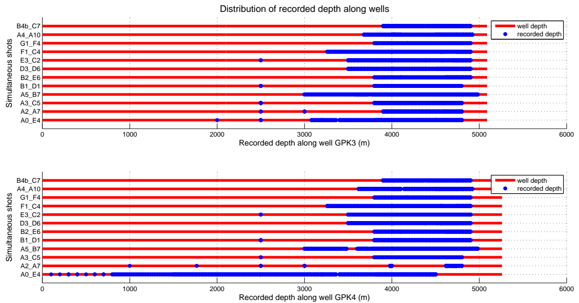
Figure 1.1.6: Distribution des profondeurs d'enregistrement dans les puits GPK3 et GPK4 pour tous les couples de sources simultanées.
