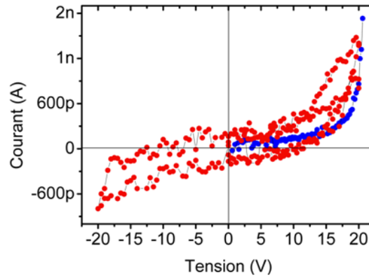
FIGURE 6.4 – Cycle d'hystérèse dans les caractéristique I(V) sur la jonction de référence Au/MgO/Fe entre [-20\text{V}, +20\text{V}] en rouge. Les caractéristique en bleu pour une tension positive.
