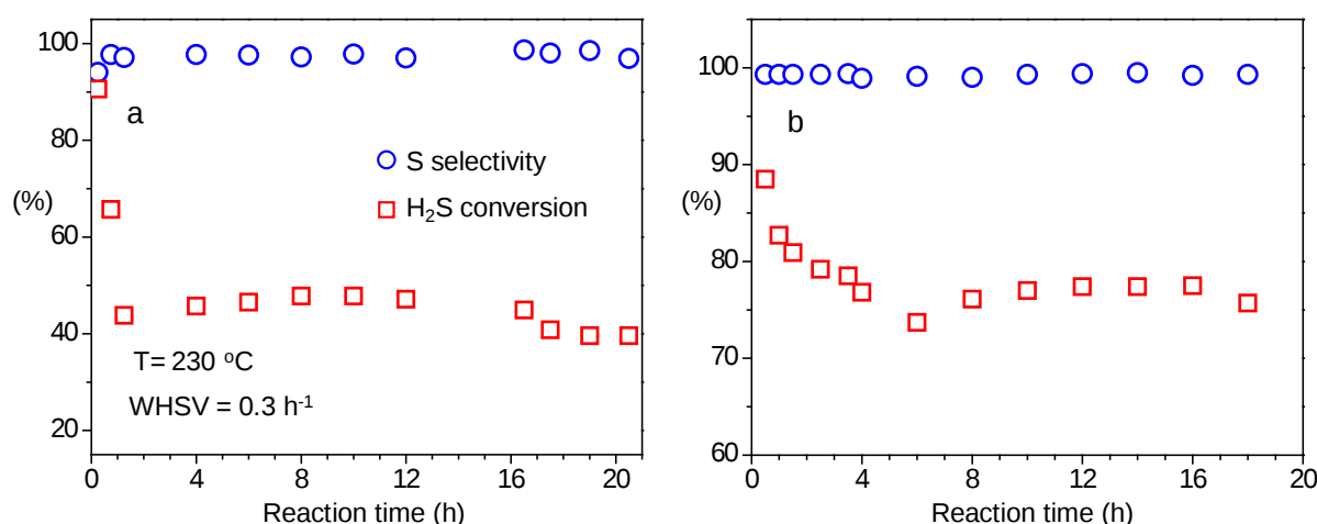
Figure 8. Performances (conversion et sélectivité) de 100 mg Au/SS5-C (a) et Au/SS5@Cu-C (b) dilués dans 200 mg de SiC en fonction du temps pour l'oxydation sélective de \text{H}_2\text{S} en Soufre à la température de 230 °C (conditions expérimentales)
