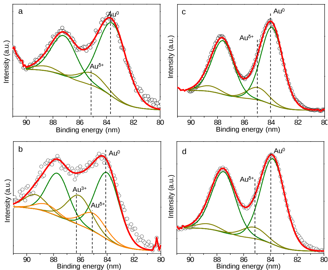
Figure 10. Spectres Au 4f XPS de Au/SS5-C et Au/SS5@Cu-C: (a-b) échantillon frais et utilisé Au/SS5-C, (c-d) échantillon frais et utilisé Au/SS5@Cu-C avant et après le test d'oxydation de \text{H}_2\text{S} . Les ronds sont les données initiales, et les lignes les courbes de dé-sommation et la courbe somme.
