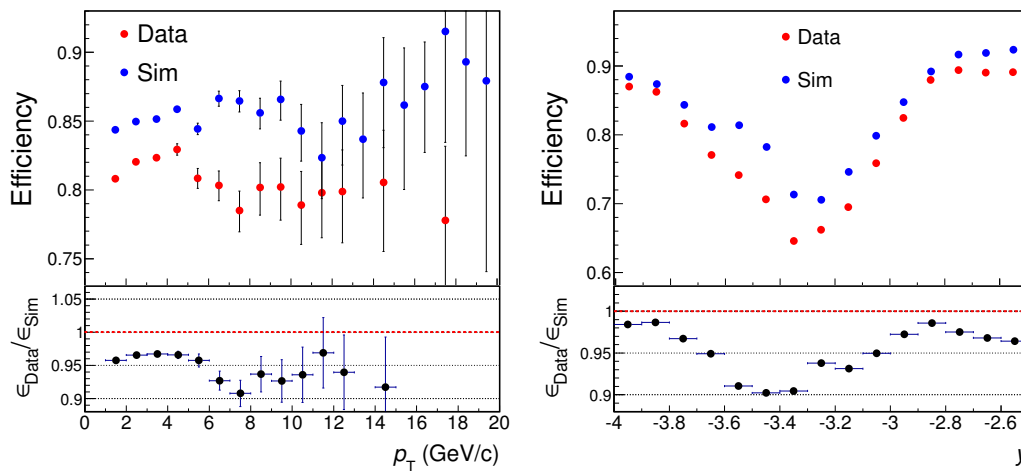
FIGURE 5.5 – Comparaison des distributions de l'efficacité de détection du trajectographe mesurée par la méthode des traces reconstruites dans les données et dans les simulations pures en fonction de l'impulsion transverse des muons (gauche) et de la rapidité des muons (droite).
