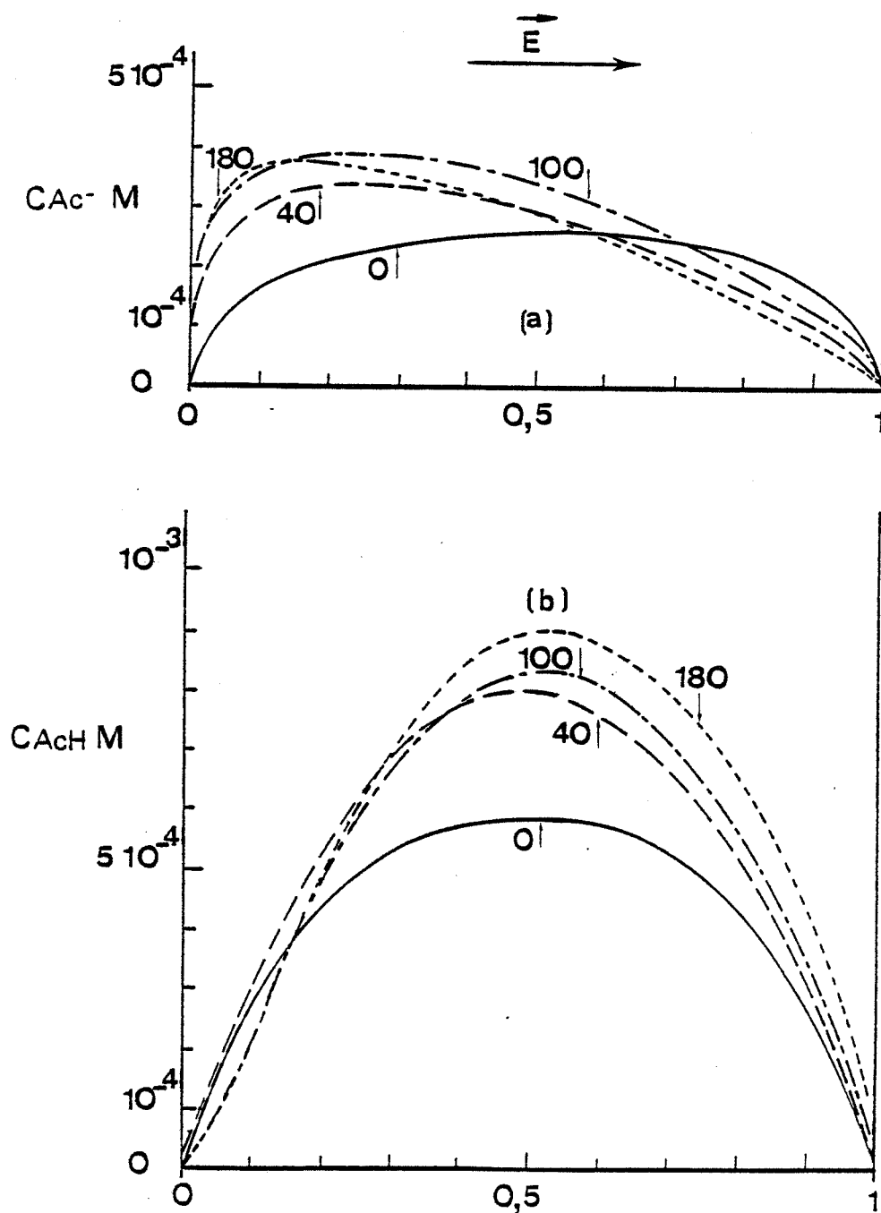
FIGURE 49 - Influence de la densité de courant sur les profils de concentration de \text{CH}_3 \cdot \text{COO}^- (Fig. 49a) et de \text{CH}_3\text{COOH} (Fig. 49b).
