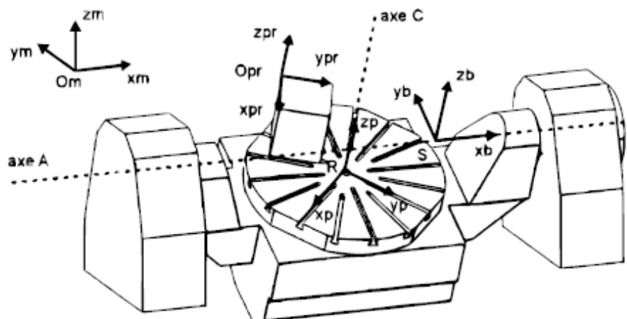
Figure D1 – Modélisation géométrique du centre d'usinage Mikron UCP 710
