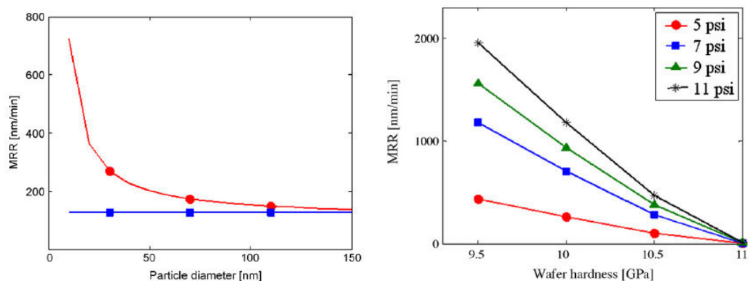
Figure 1.8 – Influence du diamètre des particules et de la dureté de la pièce [Oh et Seok (2009)]
