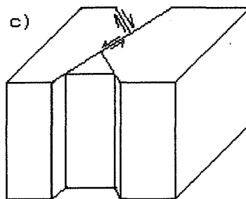
Dérochements (senestre, dextre).
