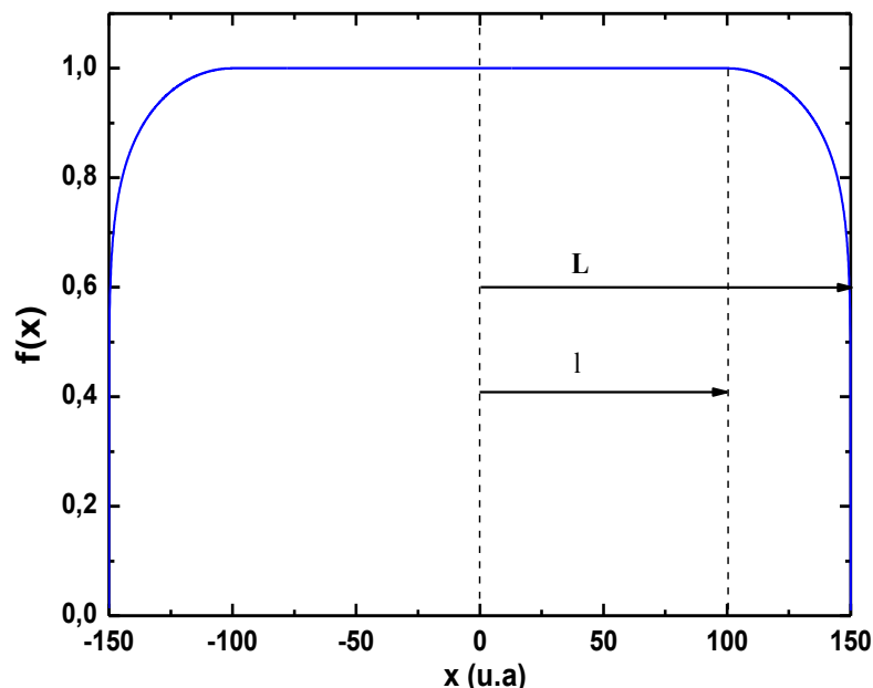
Figure 5.4 – Schéma de la fonction absorbant utilisée dans les calculs de la propagation temporelle. L est la moitié de la boîte unidimensionnelle, et L - l est la taille de l'absorbeur.
