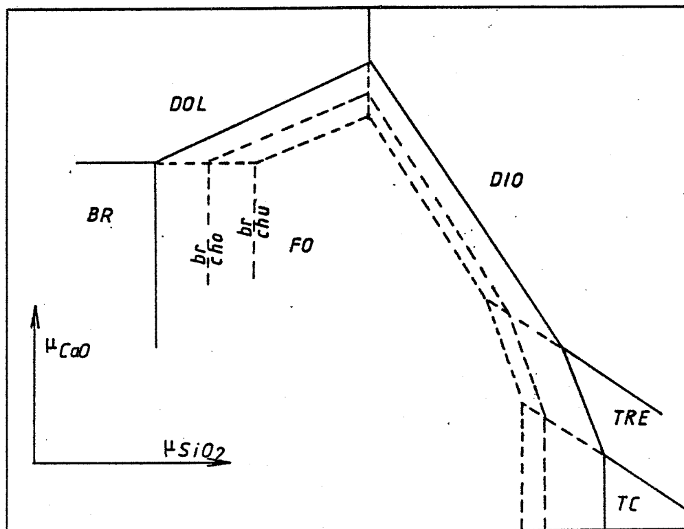
Fig. 6.2 Une des topologies solutions du système à P, T, \mu\text{CO}_2, \mu\text{H}_2\text{O} constants.
