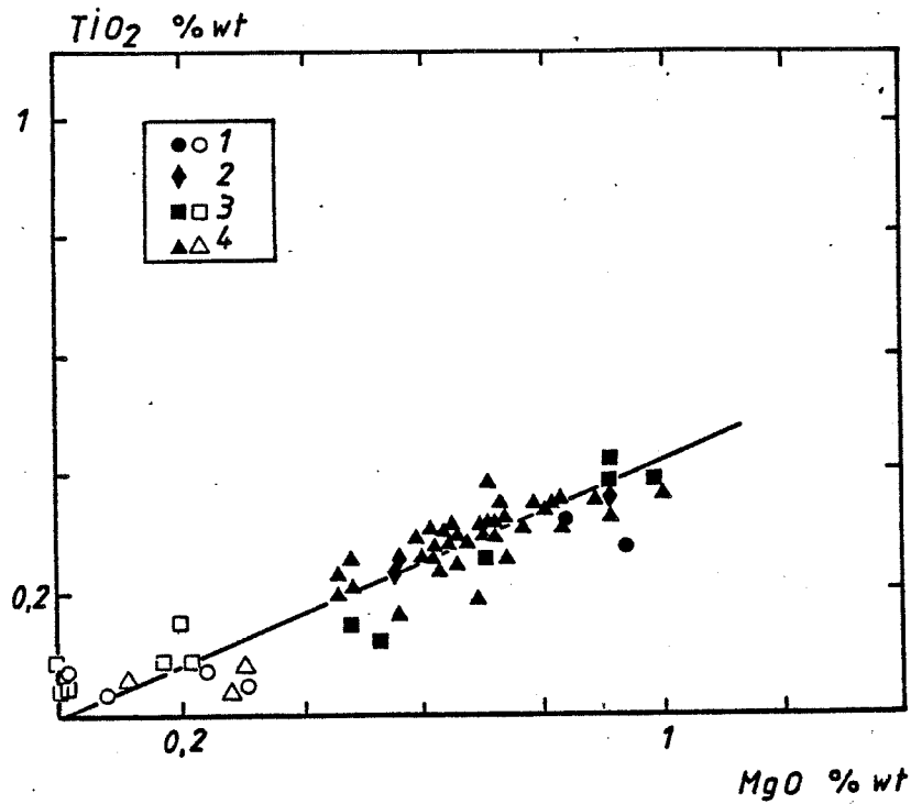
Fig. 1.2 Diagramme TiO_2:MgO des analyses du granite de Costabonne. Les figurés pleins concernent les granites à biotite, les figurés ouverts les roches sans biotites. (1): données personnelles, (2): Guitard et Laffitte (1958); (3): Le Guyader (1982); (4): Saleminck et al. (1984).
