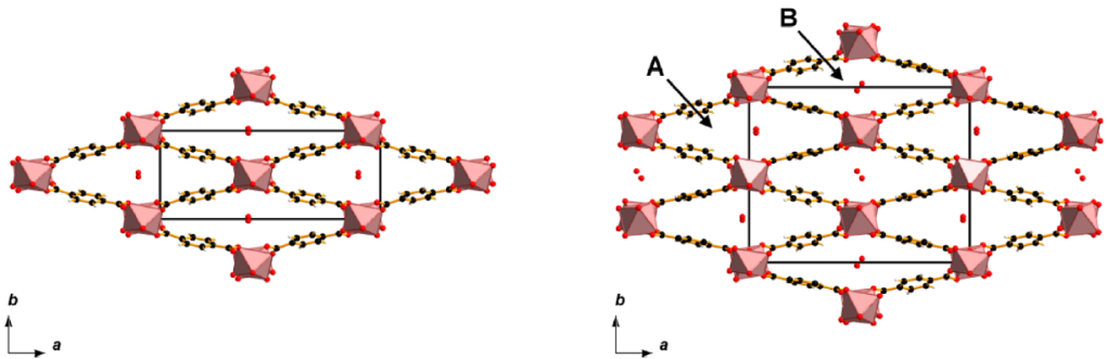
Figure 6.1 : Représentation de la structure cristallographique de la MIL-53-Ga(OH,F)-np-H 2 O (à gauche) et de la MIL-53(Ga)-np-H 2 O (à droite).
