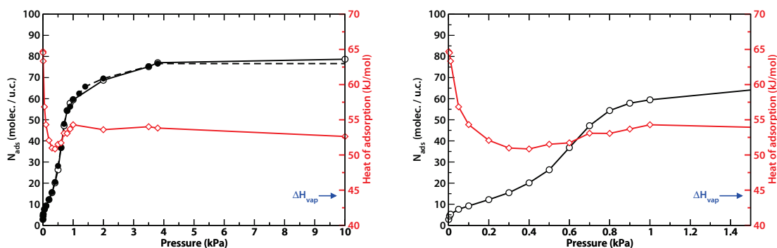
Figure 5.18 : Isothermes d'adsorption (symboles blancs) et de désorption (symboles noir) de l'intrusion d'eau dans la ZIF-90 à 300 K. La courbe rouge représente les chaleurs isothermiques d'adsorption et la flèche bleue indique l'enthalpie de vaporisation de l'eau bulk à 300 K.
