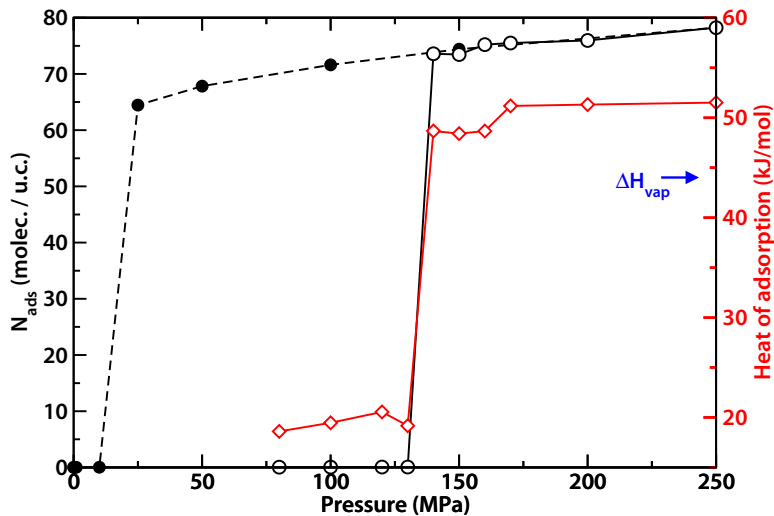
Figure 5.13 : Isothermes d'adsorption (symboles blancs) et de désorption (symboles noirs) de l'intrusion d'eau dans la ZIF-8 à 300 K. La courbe rouge représente les chaleurs isostériques d'adsorption et la flèche bleue indique l'enthalpie de vaporisation de l'eau bulk à 300 K.
