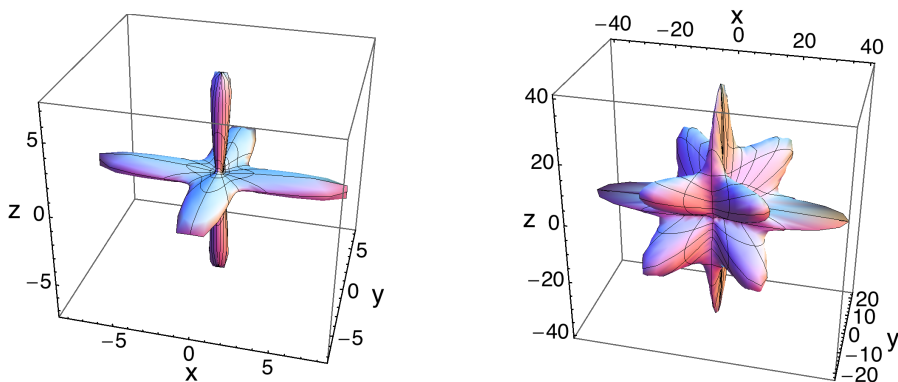
Figure 3.13 : Représentation 3D du module de cisaillement de la MIL-53(Al)-lp. Les modules de cisaillement minimal et maximal sont respectivement représentés à gauche et à droite. Les axes sont gradués en GPa.
