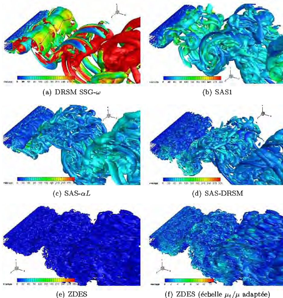
FIGURE 5.45 – Iso-surfaces du critère Q ( Q = -100 \text{ s}^{-2} ) colorées par le rapport de viscosité \mu_t/\mu sur le maillage 2
