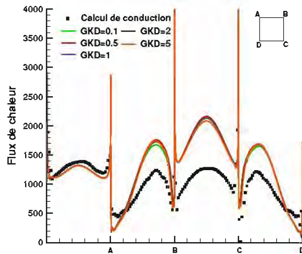
FIGURE 5.16 – Flux de chaleur pariétal ( W.m^{-2} ) moyenné en temps et en espace selon gkd
