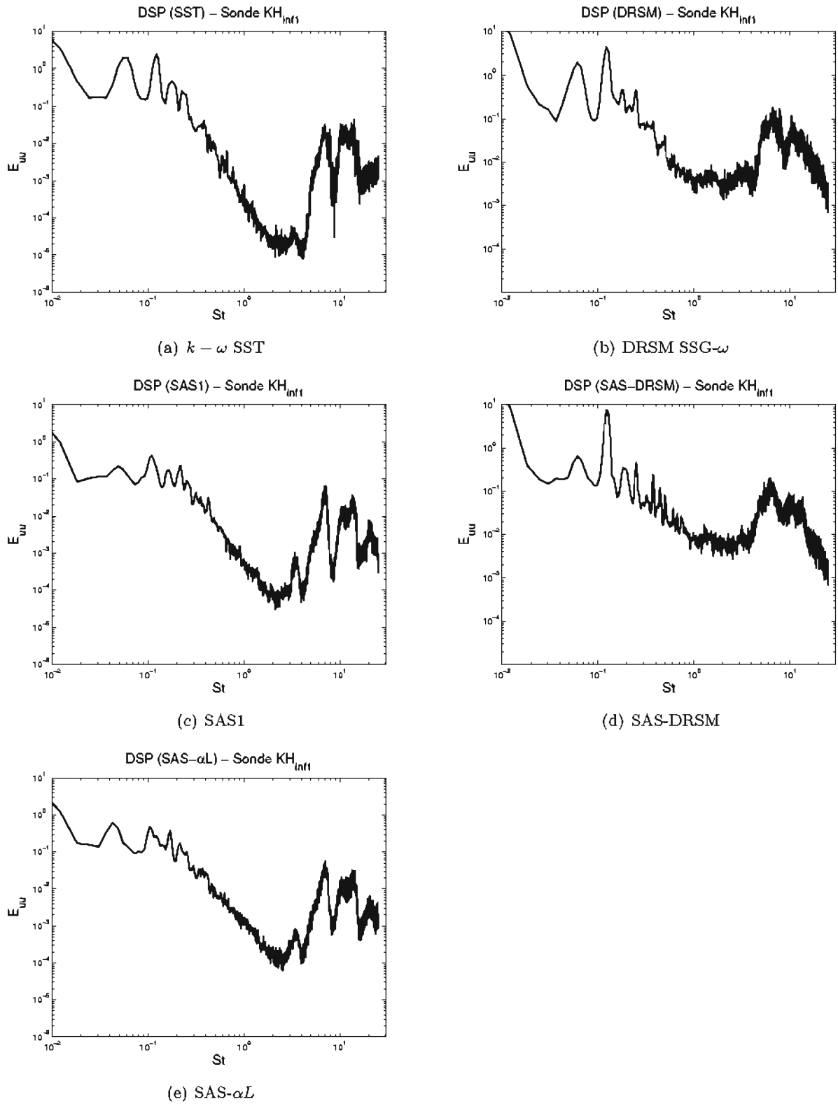
FIGURE 33 – Densités spectrales de puissance de v'_1 u'_1 obtenues à la sonde KH_{inf1} en fonction du nombre de Strouhal sur le maillage 1
