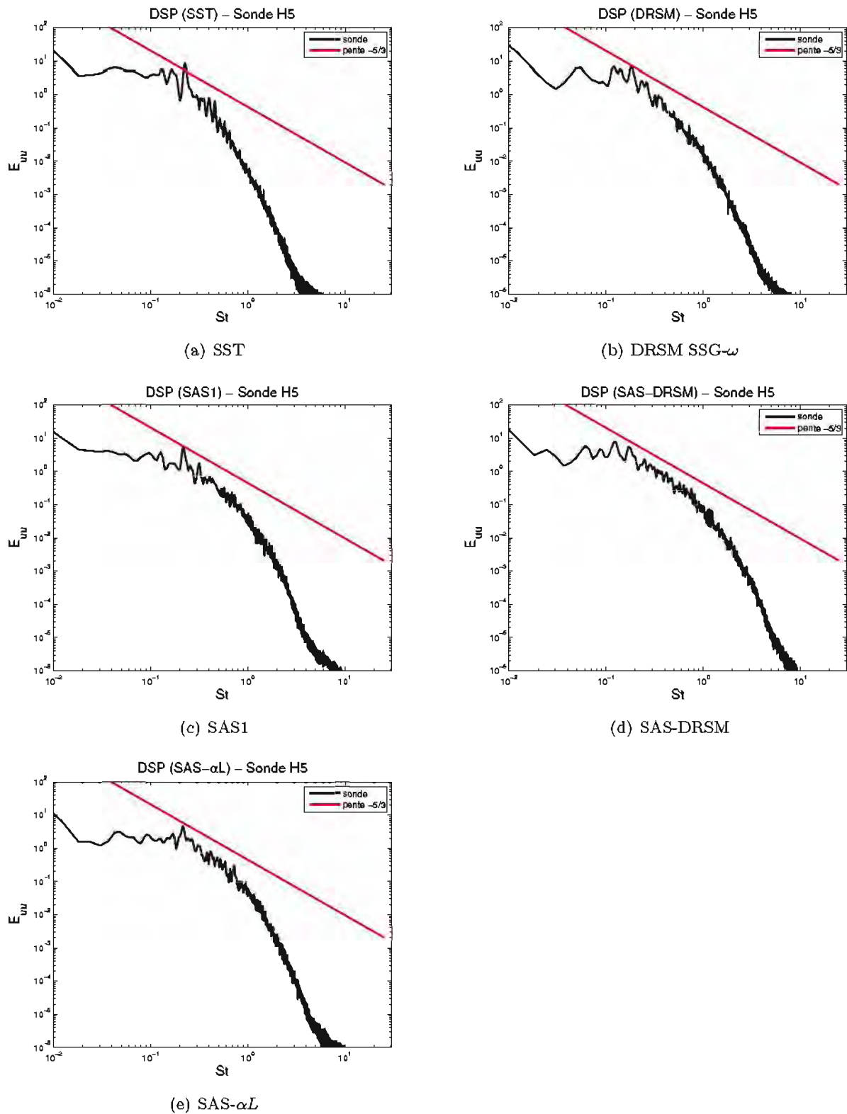
FIGURE 5.36 – Densités spectrales de puissance de u'_1 u'_1 obtenues à la sonde H5 en fonction du nombre de Strouhal sur le maillage 1
