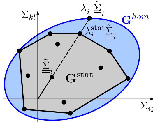
FIGURE 4.3 – Approche statique par l'intérieur du domaine de résistance macroscopique.
