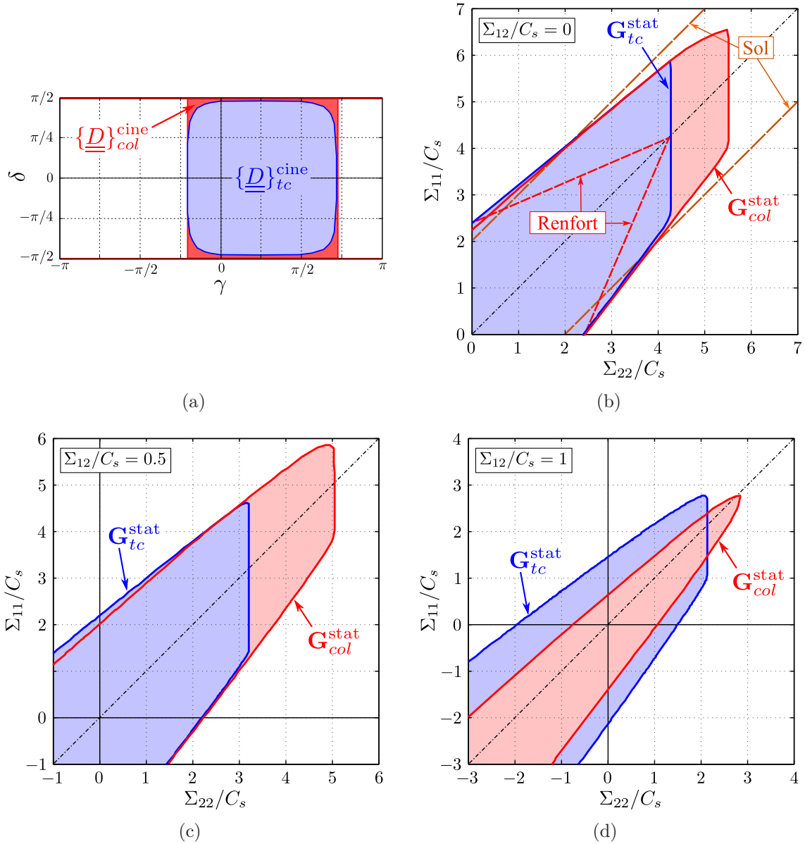
FIGURE 7.15 – Comparaison de \mathbf{G}_{col}^{stat} et \mathbf{G}_{tc}^{stat} pour différentes valeurs de \Sigma_{12}/C_s .
