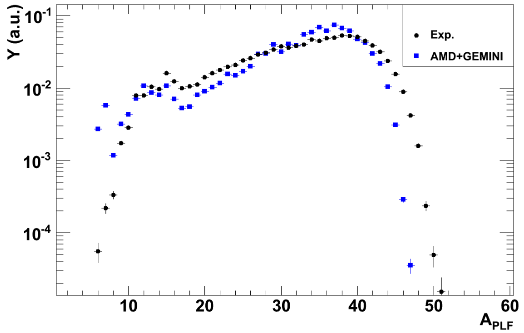
FIGURE 3.27 – Comparison des distributions normalisées avec l'aire sous la courbe en masses des PLF pour le système ^{48}\text{Ca}+^{48}\text{Ca} .
