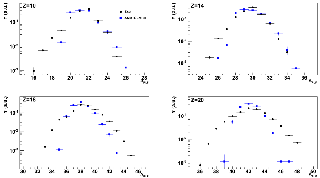
FIGURE 3.28 – Comparison des distributions isotopiques des PLF pour le système ^{48}\text{Ca}+^{48}\text{Ca} .
