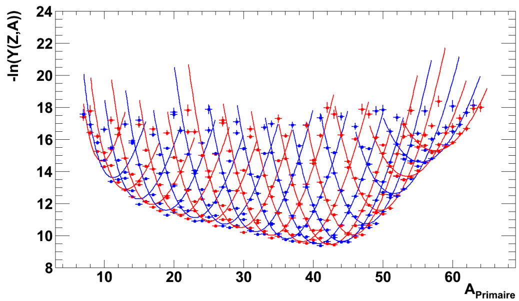
FIGURE 5.41 – Distribution -\ln(Y(Z,A)) pour le système ^{48}\text{Ca} + ^{48}\text{Ca} et avec l'ajustement fait sur chaque charge. Les points rouges correspondent aux charges impaires alors que les points bleus correspondent aux charges paires.
