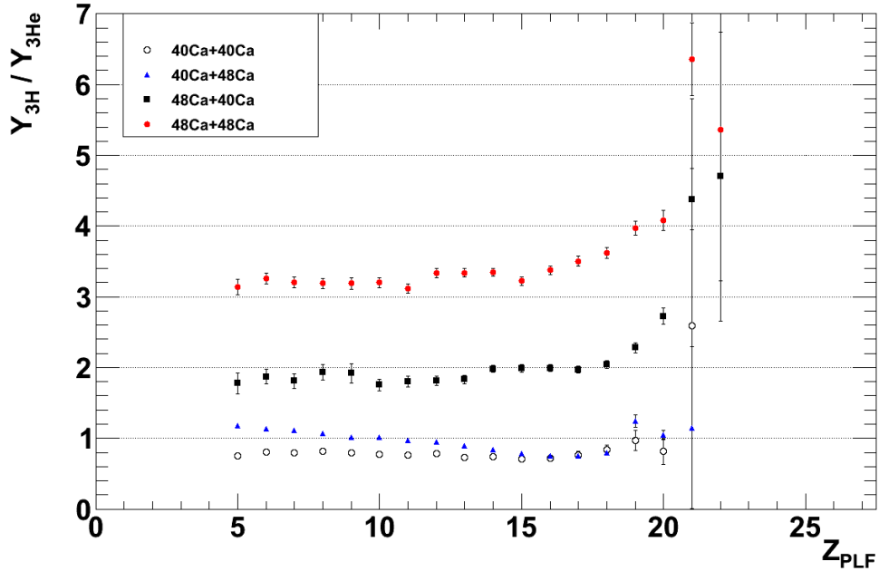
FIGURE 5.14 – Rapport des multiplicités de ^3H et de ^3He pour les différents systèmes.
