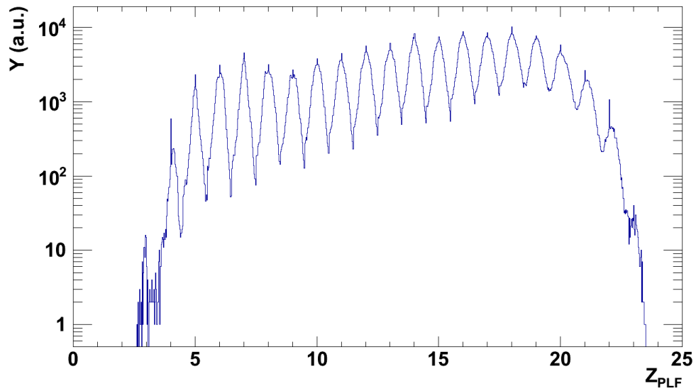
FIGURE A.10 – Distribution en Z pour le système ^{48}\text{Ca}+^{48}\text{Ca} .
