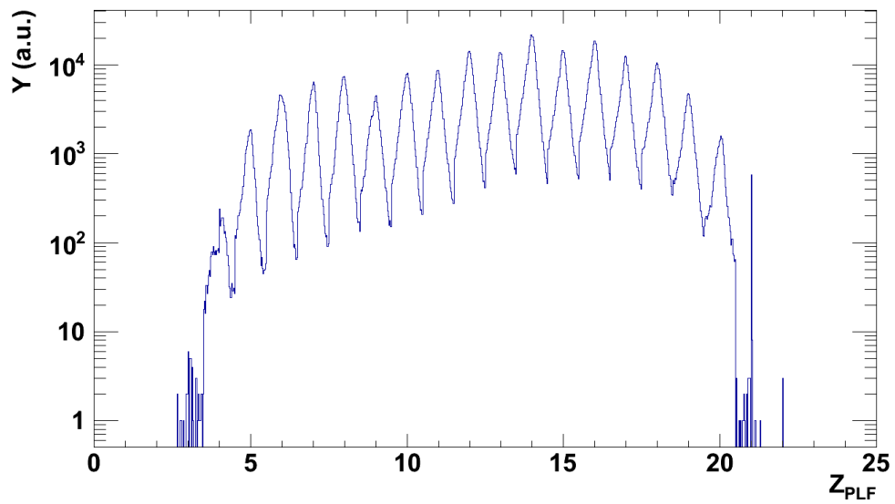
FIGURE A.4 – Distribution en Z pour le système ^{40}\text{Ca}+^{48}\text{Ca} .
