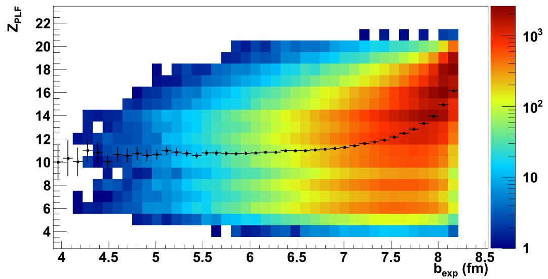
FIGURE B.5 – Charge PLF en fonction du paramètre d'impact expérimental pour le système ^{40}\text{Ca}+^{40}\text{Ca} .
