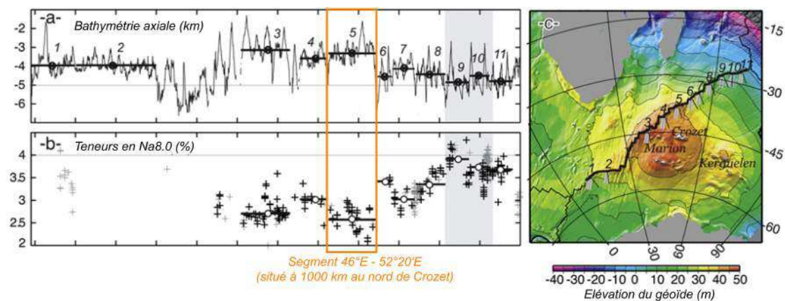
FIGURE 1.6 – a) bathymétrie à l’axe de la ride sud-ouest indienne, b) teneurs en \text{Na}_{8,0} à l’axe de la ride sud-ouest indienne et c) carte d’anomalie du géoïde centrée sur le plateau de Crozet. Figure issue de l’étude de Cannat et al. (2008) (fig. 1) et mise en évidence sur les figures a) et b) du segment de ride 46^\circ\text{E} - 52^\circ 20'\text{E} (segment 5 en fig. a et c) concerné par l’interaction potentielle avec le point chaud de Crozet (Cannat et al., 2008; Sauter et al., 2009).
