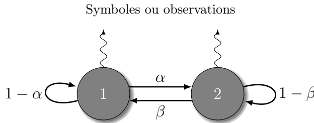
Fig 1.5 – Modèle de Markov Caché à deux états.
