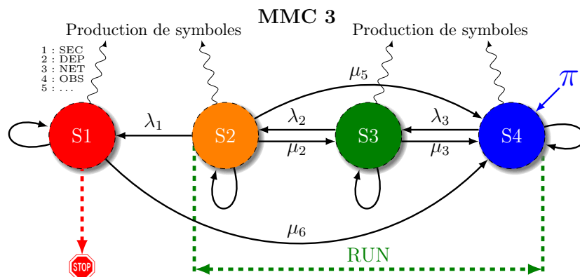
Fig 4.15 – Modèle de Markov Caché, topologie 3.
