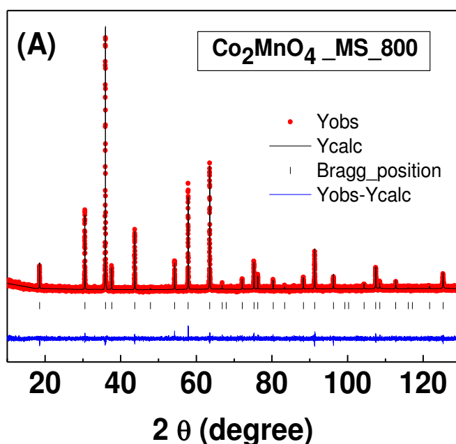
Figura 44: Refinamento de Rietveld realizado usando o programa Fullprof Suite para o composto \text{Co}_2\text{MnO}_4 , sintetizado via rota MS e tratado na temperatura de 800°C.
