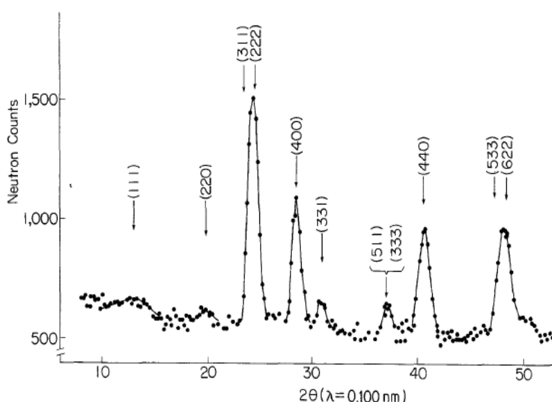
Figura 01: Perfil de difração de nêutrons do composto policristalino \text{MnCo}_2\text{O}_4 , em temperatura ambiente, preparados via métodos úmidos em T = 80^\circ\text{C} . (YAMAMOTO et al., 1983).
