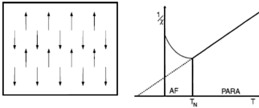
Figura 17: Alinhamento dos momentos magnéticos de um material antiferromagnético (AFM). Magnetização e inverso da susceptibilidade magnética ( 1/\chi ) dependentes da temperatura ( T ) de um material AFM (HILL, 2000) (GUIMARÃES e OLIVEIRA, 1998).
