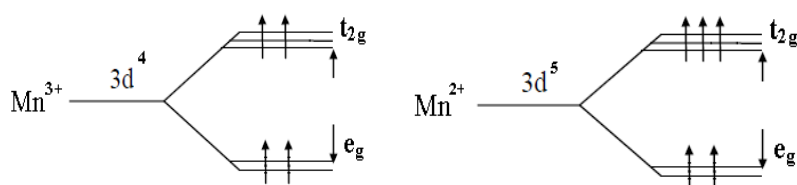
Figura 69: Esquema de distribuição dos elétrons nos níveis de energia t_{2g} e e_g , de acordo com a teoria do Campo Cristalino para os cátions Mn^{3+} e Mn^{4+} (BORDENEUVE, 2009) (CHEN; WU e SELLONI, 2011).
