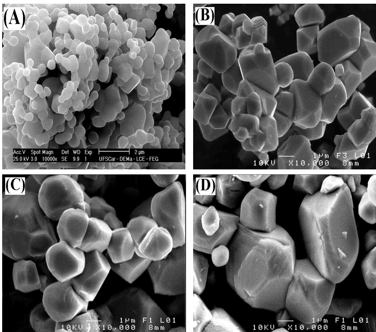
Figura 51: Imagens de MEV das amostras (A) \text{Co}_2\text{MnO}_4 , (B) \text{Bi}_{0,1}\text{Co}_{1,9}\text{MnO}_4 , (C) \text{Bi}_{0,2}\text{Co}_{1,8}\text{MnO}_4 e (D) \text{Bi}_{0,3}\text{Co}_{1,7}\text{MnO}_4 , com resolução de aumento de 10000 vezes.
