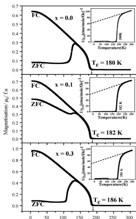
Figura 05: Dados de magnetização ZFC e FC , em função da temperatura, para \text{Bi}_x\text{Co}_{2-x}\text{MnO}_4 ( x = 0,0; 0,1; 0,2 e 0,3 ). O insert mostra as curvas de susceptibilidade magnética em função de T (RAJEEVAN et al., 2009).
