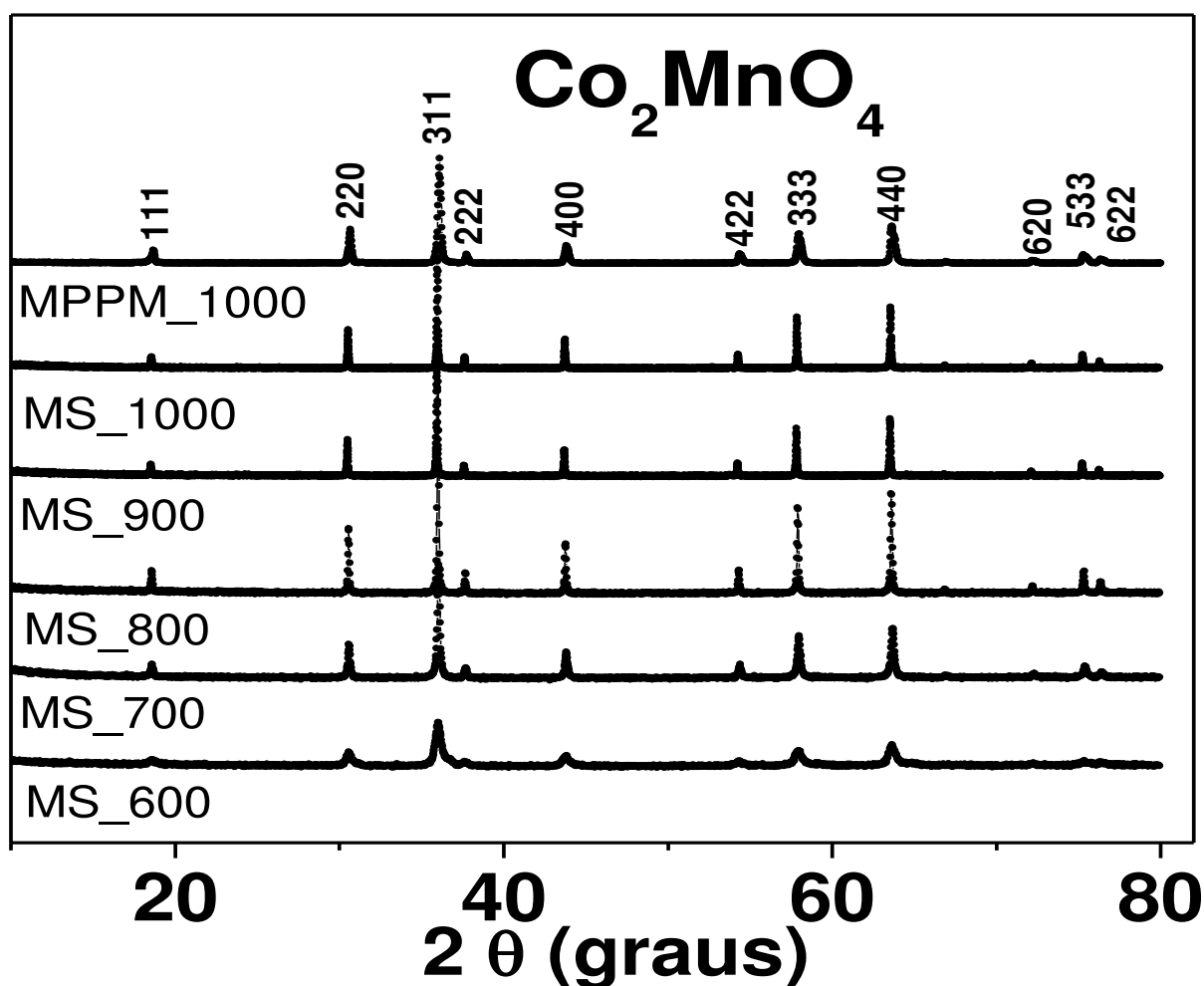
Figura 43: Perfis de difração de raios X para \text{Co}_2\text{MnO}_4 indexados com o grupo espacial Fd3m (227), sintetizados via método MS e tratados nas temperaturas de 600°C, 700°C, 800°C, 900°C e 1000°C, por 12h e comparados com uma amostra sintetizada via MPPM tratada a 1000°C, por 24h.
