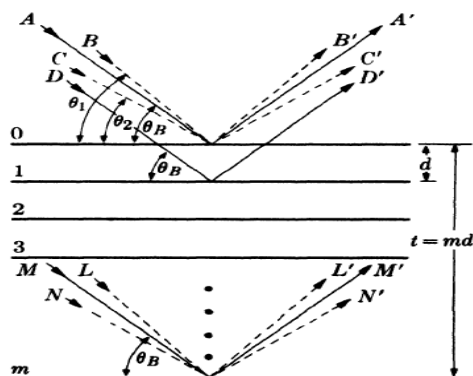
Figura 71: Modelo ilustrativo de um cristal na dedução da equação de Scherrer (CULLITY e STOCK, 2001).
