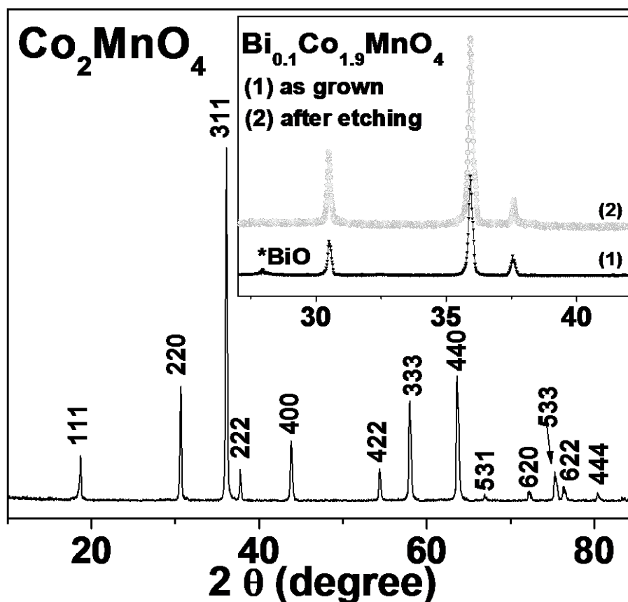
Figura 58: Perfil de DRX, \text{Cu-K}_{\alpha 1} , \lambda = 1.5418 \text{ \AA} , para \text{Co}_2\text{MnO}_4 termicamente tratada em 1000^\circ\text{C} por 12h. Insert: Perfil de XRD de \text{Bi}_{0.1}\text{Co}_{1.9}\text{MnO}_4 , antes (1) e depois do ataque químico (2), no intervalo de ângulos de Bragg de 27^\circ - 42^\circ . O símbolo * corresponde à presença do pico referente à fase \text{BiO} .
