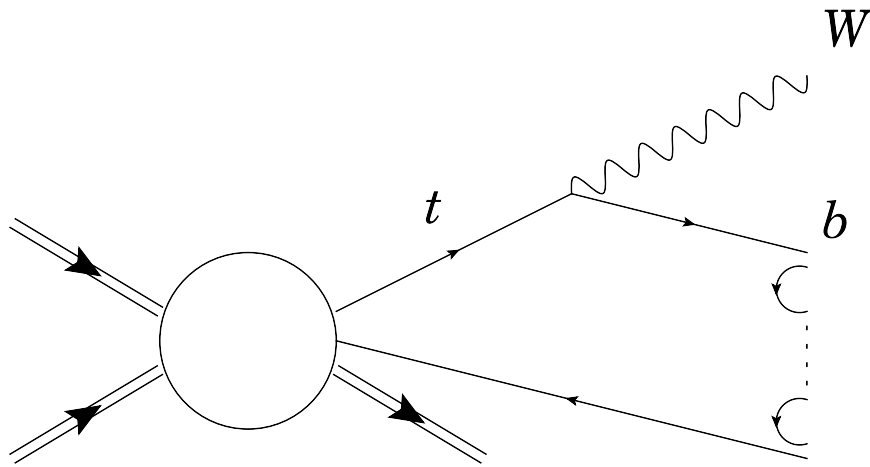
FIGURE 1.3 – Désintégration d’un quark top en QCD non perturbative.
