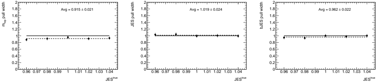
(a) Largeur des résidus de m_{\text{top}} .
