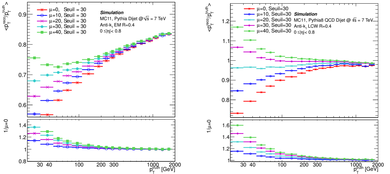
(a) Réponse des jets à l'échelle EM ( R=0.4 ) à différentes valeurs de \mu , seuil=30.
