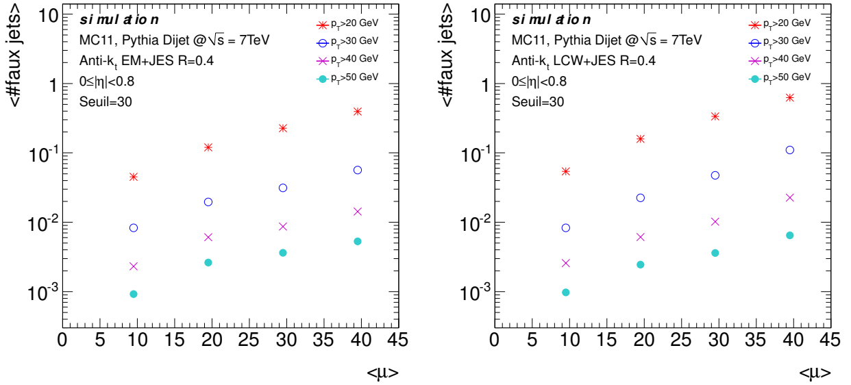
(a) Anti- k_t EM R=0.4, seuil=30
