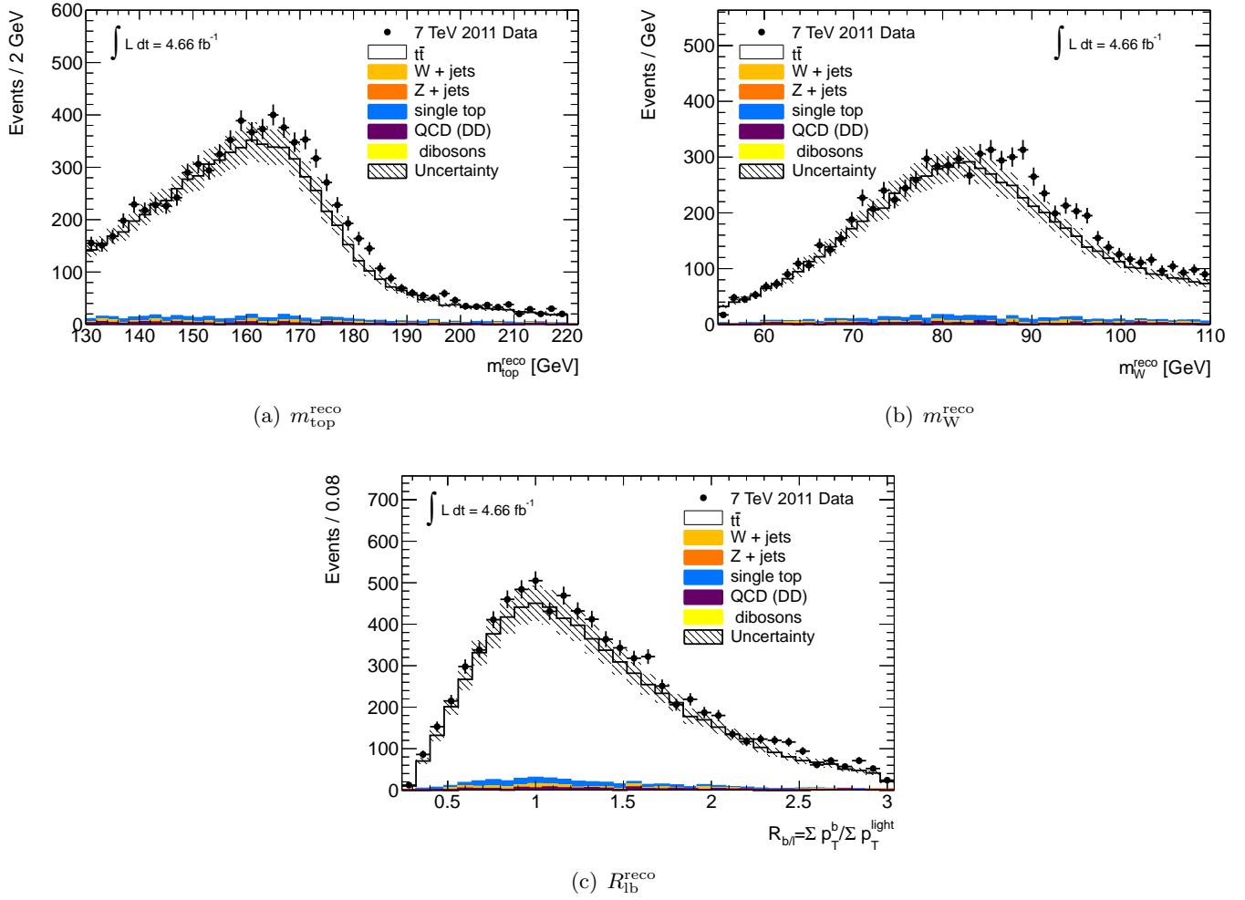
FIGURE 4.12 – Distributions des trois observables utilisées pour la mesure, après sélection finale, dans les données et dans la simulation.
