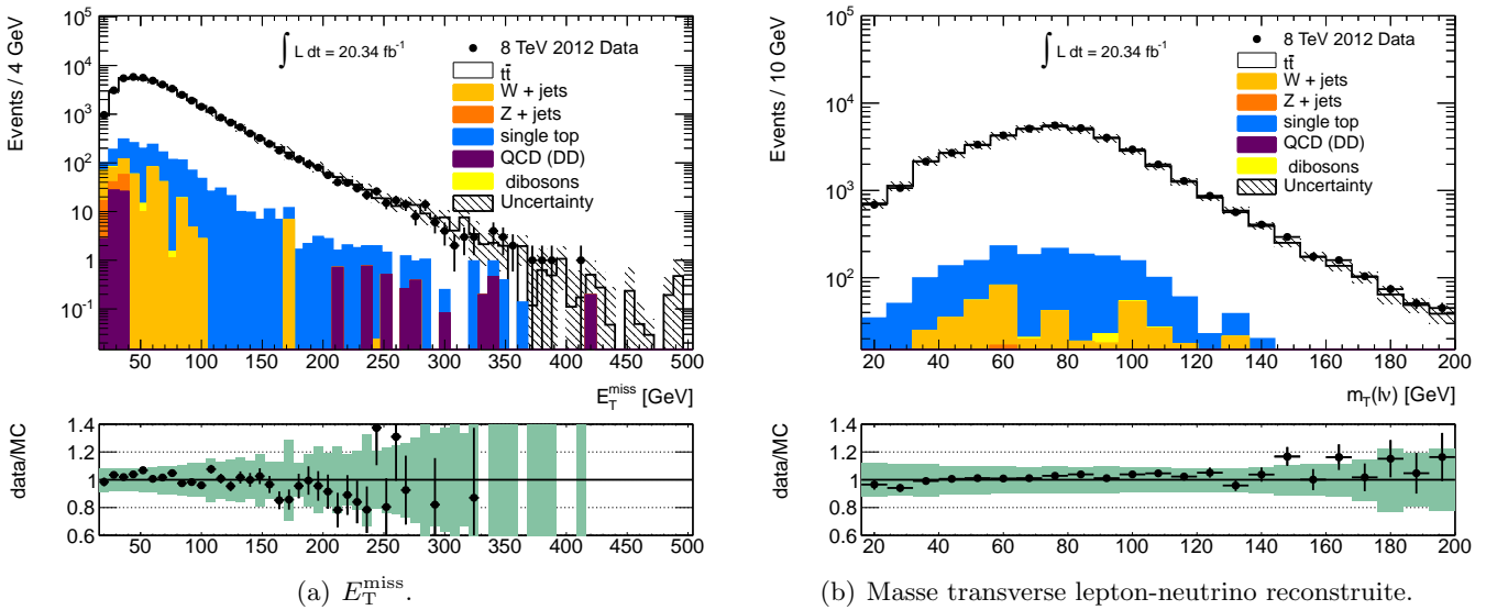
FIGURE 5.16 – Énergie transverse manquante E_T^{\text{miss}} et masse transverse m_{\text{W}}^{\text{T}} .
