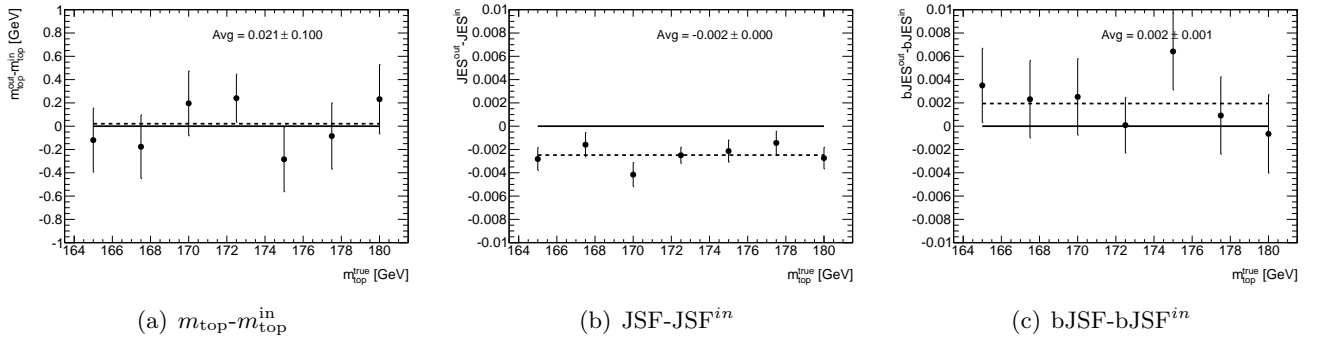
FIGURE 4.21 – Différence entre la valeur des paramètres mesurés et leur vraie valeur en fonction de la valeur d'entrée de masse du quark top dans la simulation m_{\text{top}}^{\text{in}} . Les valeurs de \text{JSF}^{\text{in}} et de \text{bJSF}^{\text{in}} sont toutes deux fixées à 1.
