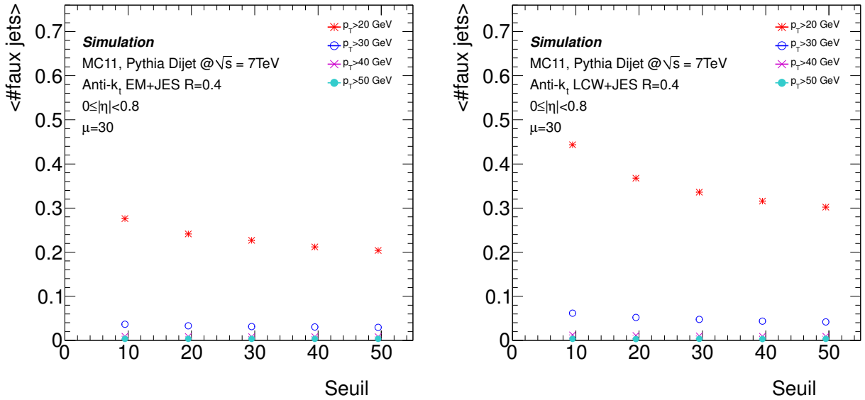
(c) Anti- k_t EM R=0.4, \mu=30
