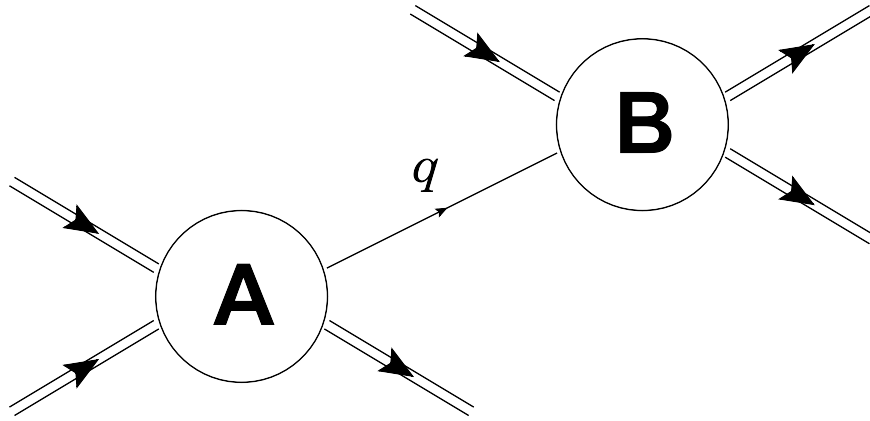
FIGURE 1.2 – Processus diffusif dont l’amplitude possède un pôle à la masse d’un quark. Les lignes externes des sous-amplitudes sont des états singlets de couleur. Un tel processus est interdit par la conservation de couleur de la QCD.
