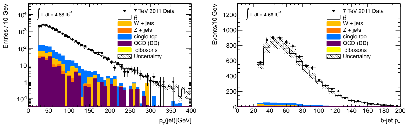
(a) p_T des jets assignés aux W issus des tops hadroniques.
