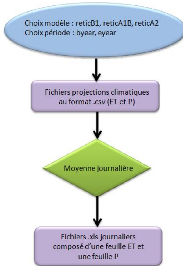
Figure 5.9 Schéma de l'algorithme du script permettant le calcul des moyennes journalières au format .xls à partir du fichier .csv regroupant toutes les données
