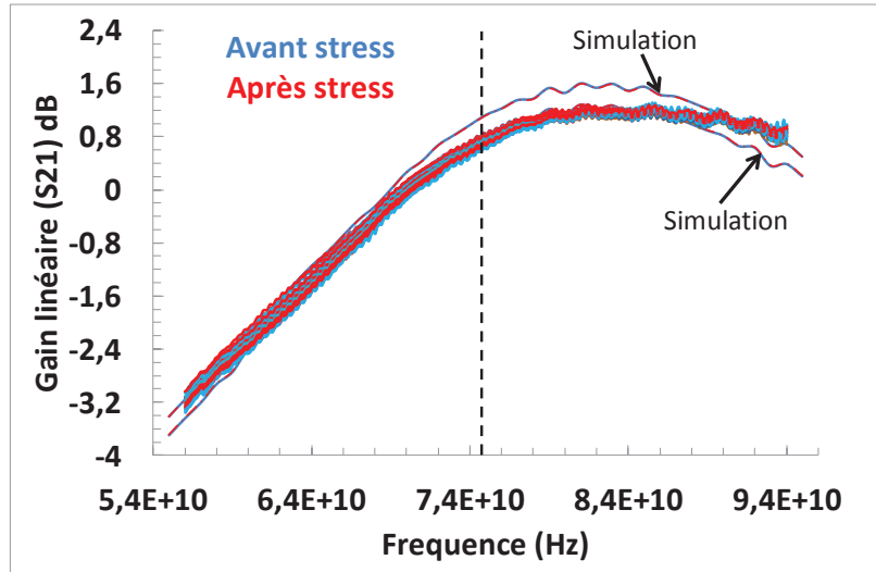
Figure 134 : Comparaison du paramètre du gain petit signal S21 avant et apres stress.
