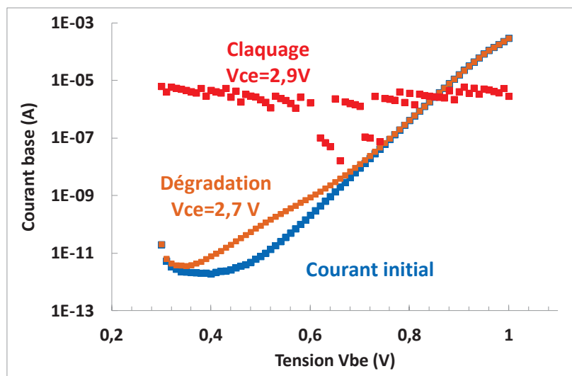
Figure 102 : Evolution des mesures de Gummel lors des rampes en tension V_{CE} .
