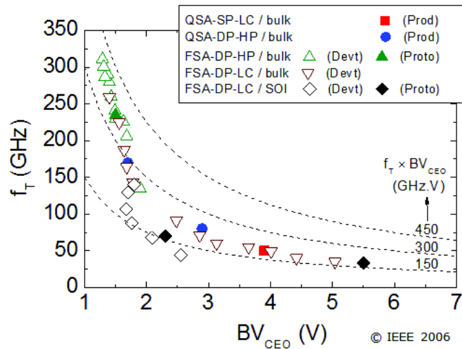
Figure 4 : Evolution de la fréquence de transition en fonction de la tension de claquage de la jonction collecteur émetteur en base ouverte.
