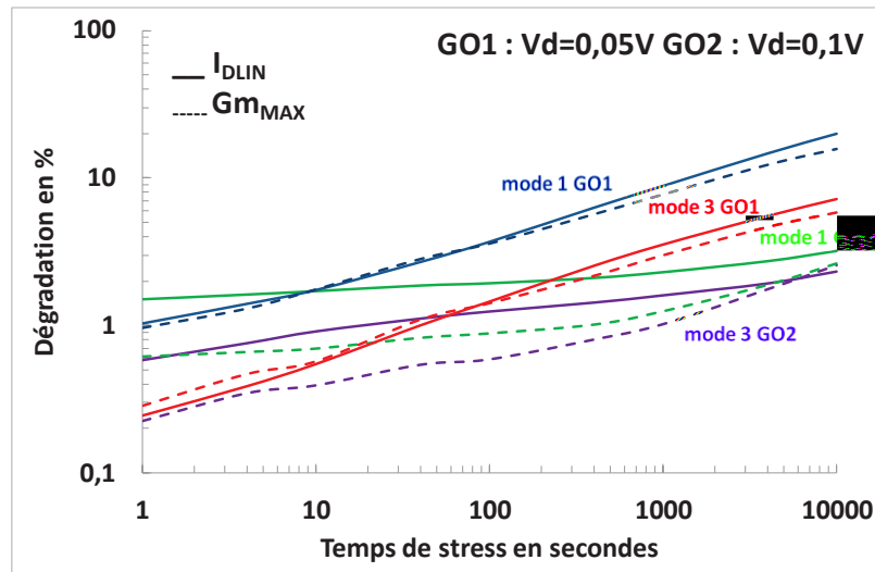
Figure 67 : Comparaison de l'évolution de la transconductance maximale et du courant de drain linéaire des transistors MOS de type GO1 et GO2 sous stress par porteurs chauds suivant le mode 1 et 3.
