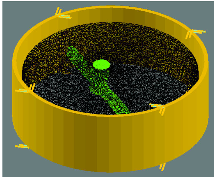
Figure 4.2 : Maillage électromagnétique avec la bobine non-maillée.
