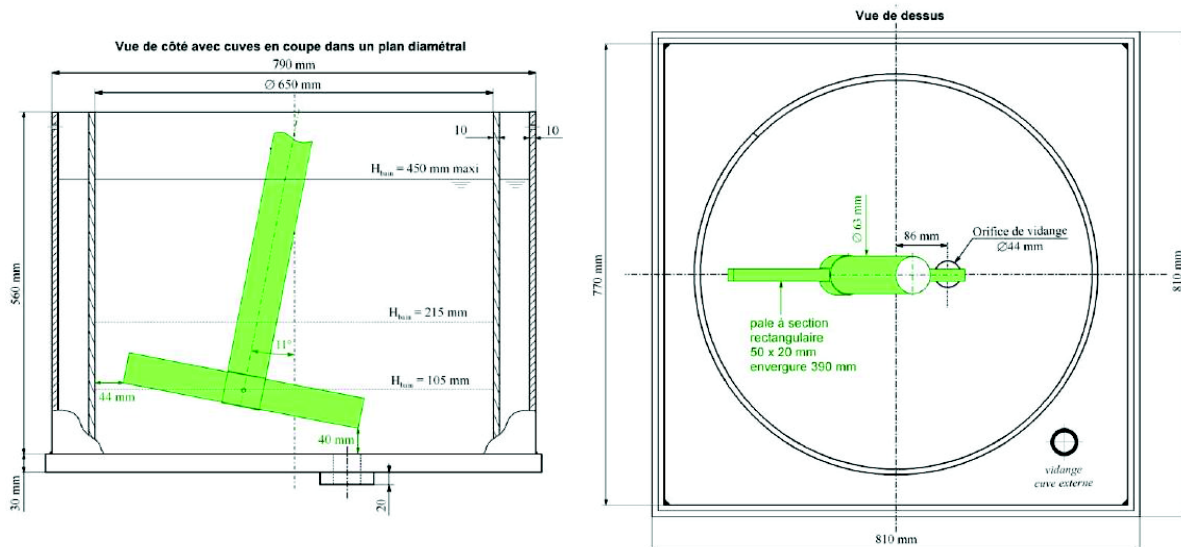
Figure 2.4 : Vue latérale et supérieure de la cuve de \text{Ø}650 mm.
