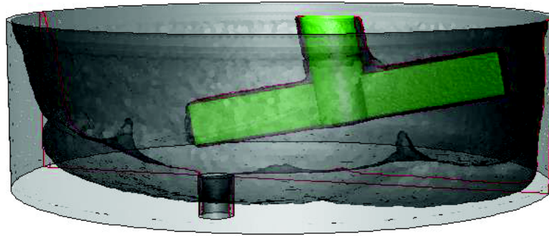
Figure 4.12 : Visualisation tridimensionnelle (en gris) et sur le plan-xz (en rouge) de l'autocresset pour t = 8,4 s. Viscosité du verre entre 10 et 10^4 Pa.s.
