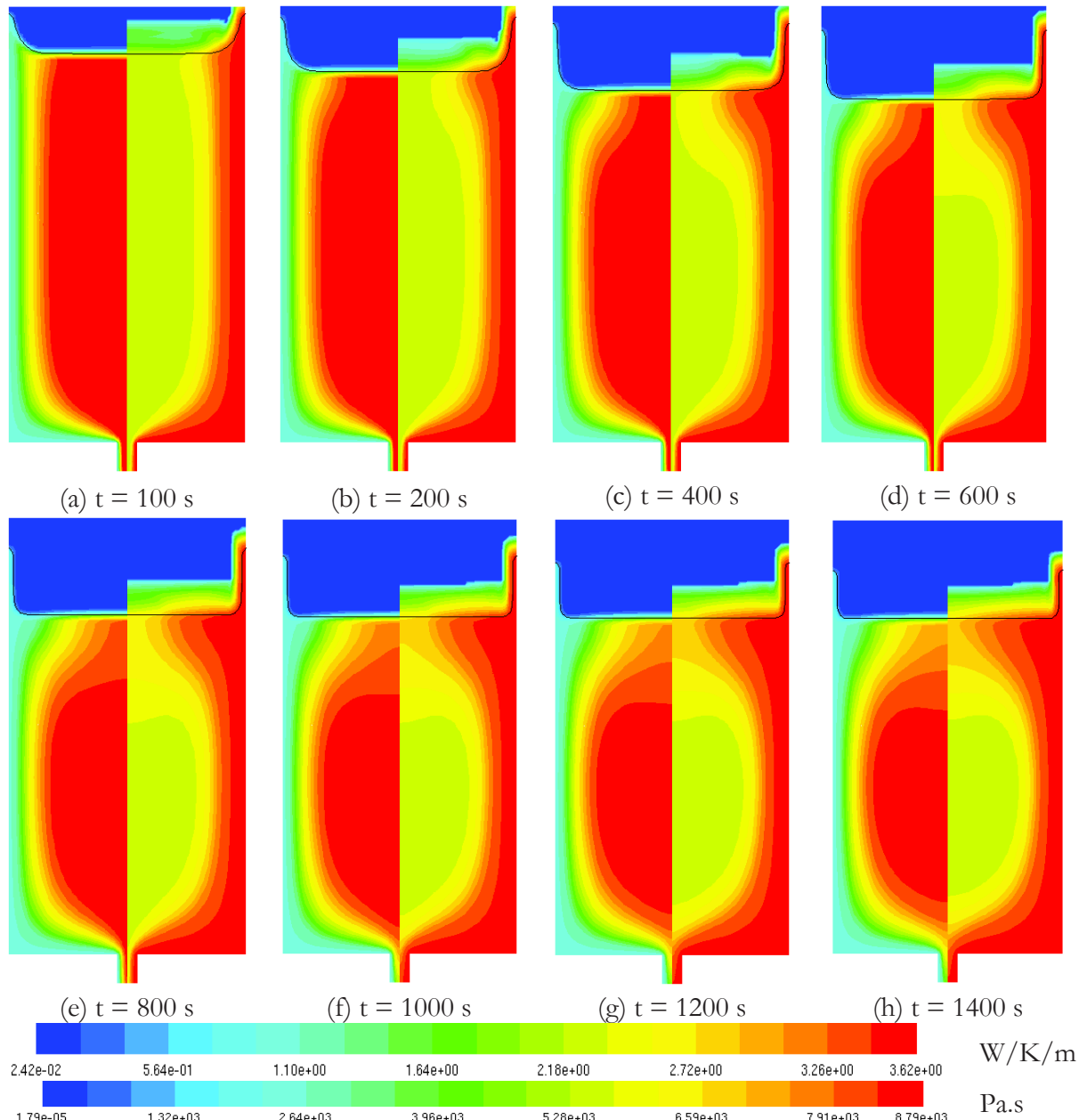
Figure 3.15 : Profil de la conductivité thermique (côté gauche) et de la viscosité (côté droit). Visualisation dans le plan-xz.
