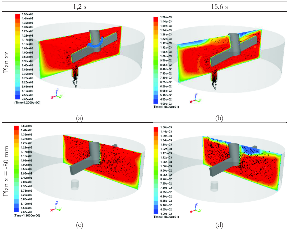
Figure 4.18 : Champ de température sur les plans « x,z » et « x = -80 mm » superposé par des vecteurs de vitesse pour les instants de 1,2 et 15,6 s. 50 tr/mn – sens horaire (flèche bleue).
