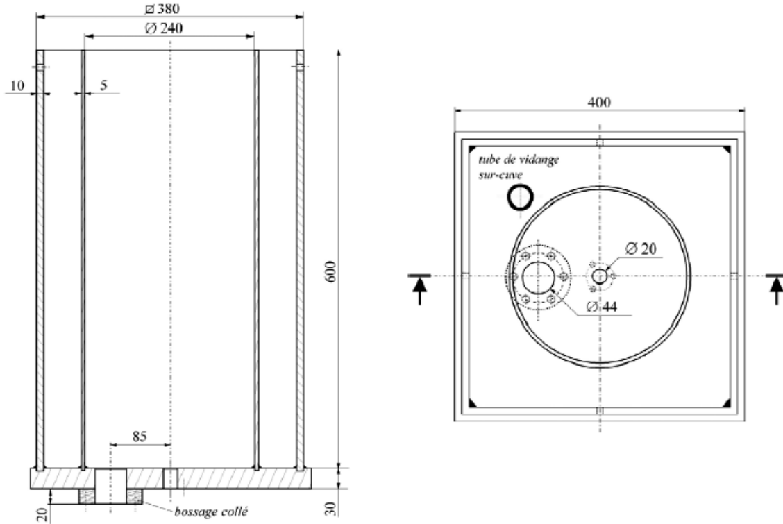
Figure 2.3 : Vue latérale et supérieure de la cuve de \text{Ø}240 mm.
