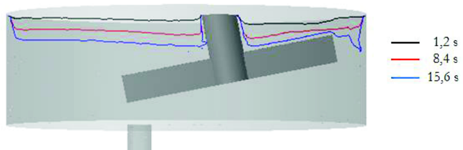
Figure 4.13 : Déplacement de la surface libre sur le plan-xz pour t = 1,2 ; 8,4 et 15,6 s.
