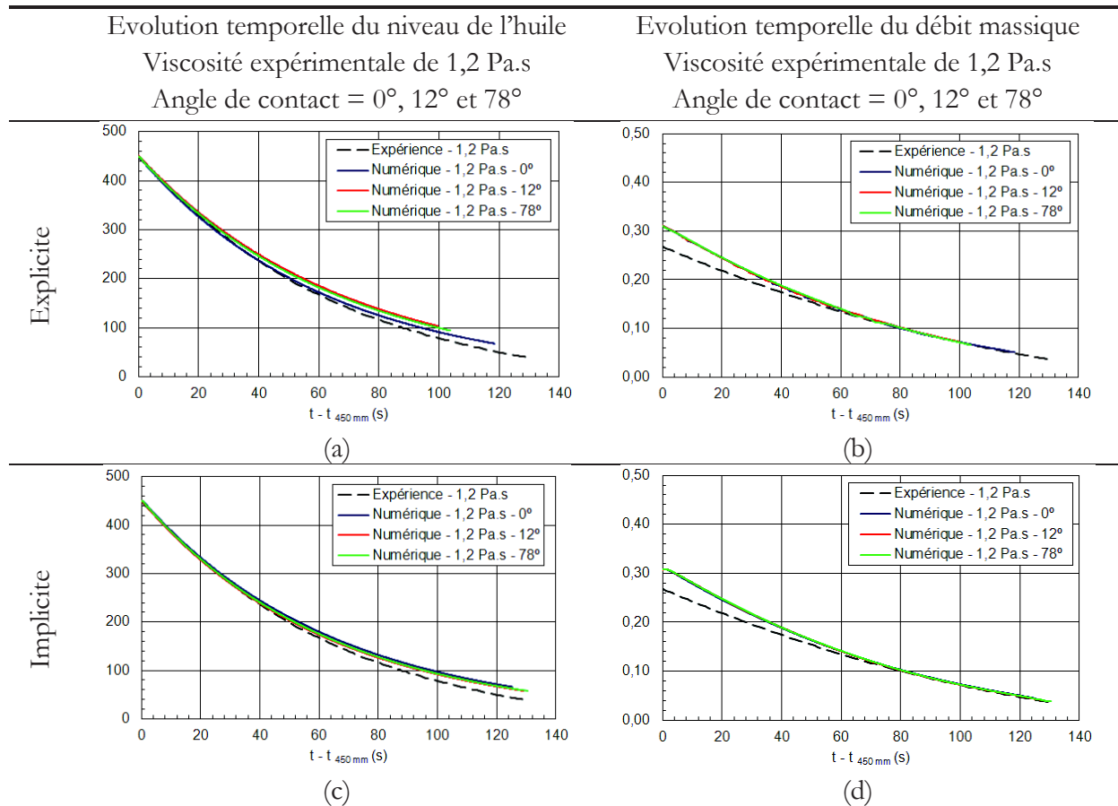
Figure 2.16 : Comparaison entre les essais expérimentaux (en noir), et les modèles numérique pour les angles de contact de 0° (en bleu), 12° (en rouge) et 78° (en vert) pour la viscosité expérimentale de 1,2 Pa.s. Echelle du niveau de l'huile en mm. Echelle du débit massique en kg/s.
