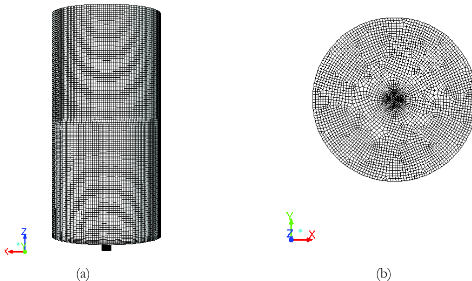
Figure 2.14 : Visualisation du maillage de la cuve \text{Ø}240 mm avec un orifice de coulée \text{Ø}20 \times 30 mm, en position centrale. Vue latérale (a). Vue supérieure (b).
