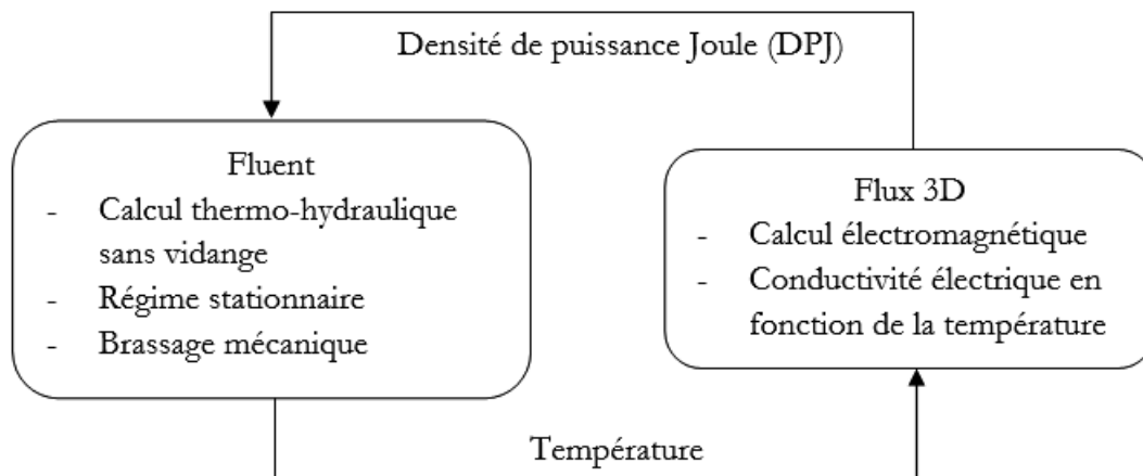
Figure 4.3 : Schéma du couplage entre les sous-systèmes thermique et électromagnétique dans l'étape d'initialisation du calcul de la vidange du four avec agitation mécanique : calcul thermo-hydraulique du flux de verre et calcul thermo-hydraulique de la vidange du four
