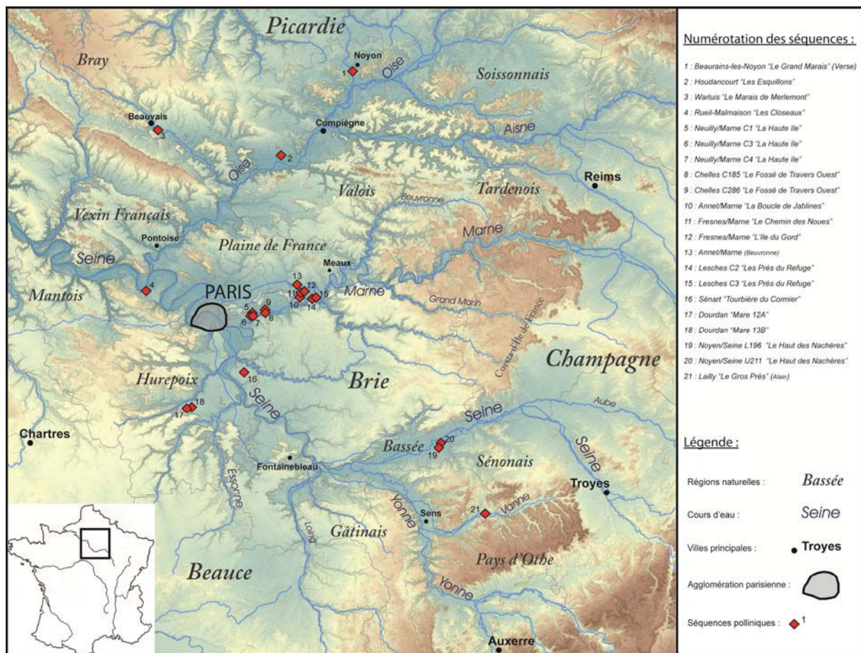
Fig. 3 : Relief, réseau hydrographique et régions naturelles du Bassin parisien
