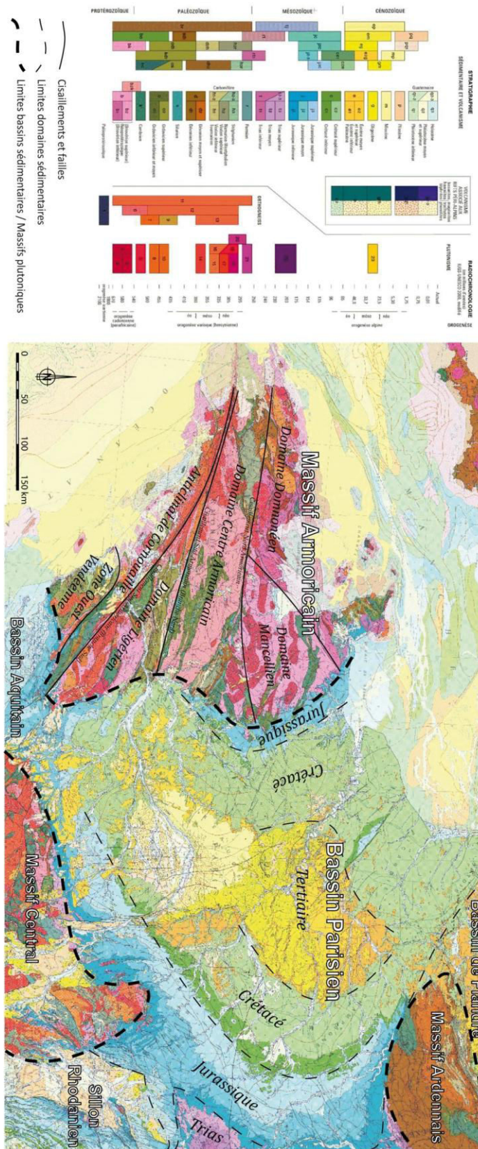
Fig. 1 : Carte géologique du Nord-Ouest de la France (Modifiée d'après BRGM)
