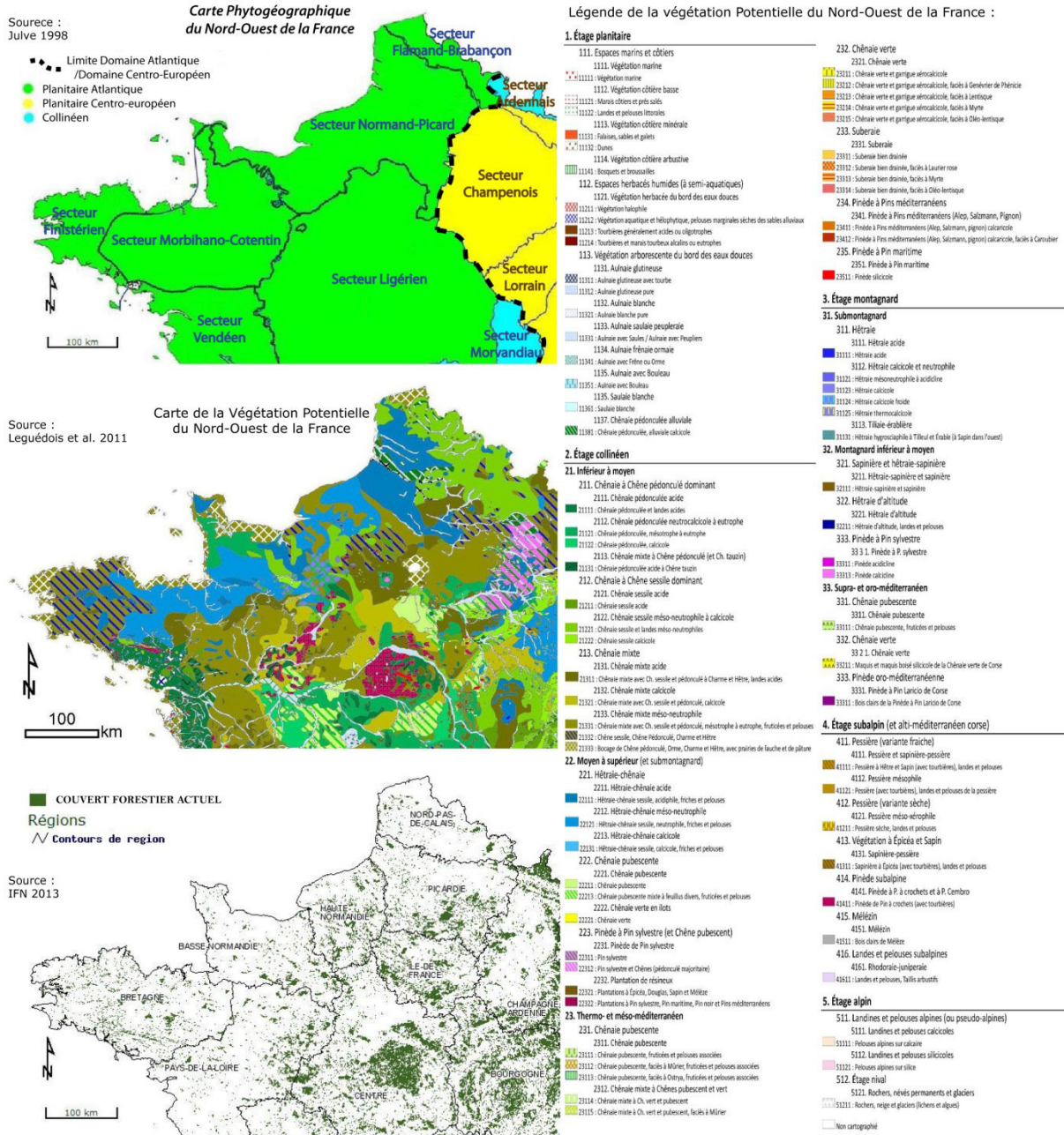
Fig. 5 : Phytogéographie, végétation potentielle, et couvert forestier actuel dans le nord-ouest de la France (Modifié d'après Julve 1998 ; Leguédols et al. 2011 ; IFN ; http://inventaire-forestier.ign.fr/carto/carto/afficherCarto/ )
