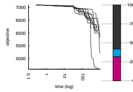
1.109 vrp_A-n62-k8.vrp with EBLNS
