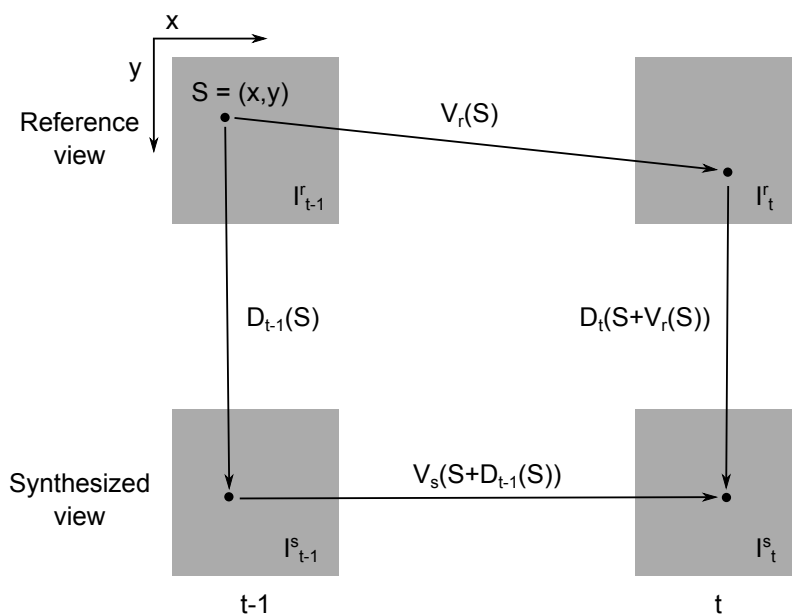
Figure 22: Contrainte épipolaire
