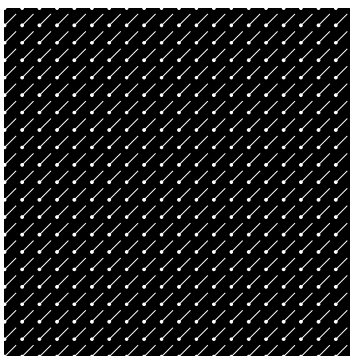
Représentation du poussé en avant d'un champ de vecteurs à partir du plan à la surface
