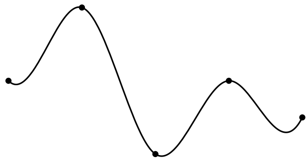
Représentation d'une spline cubique à travers 5 points de données (forme non paramétrique)
