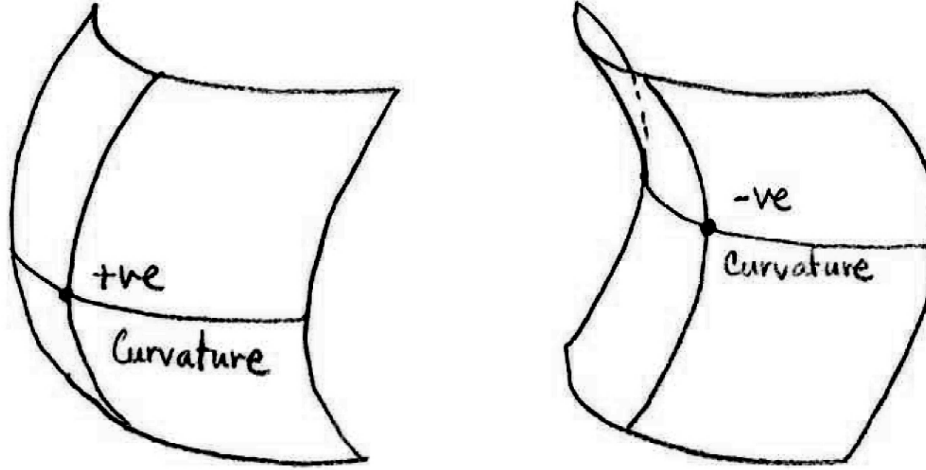
Représentation de courbure gaussienne positive et négative
