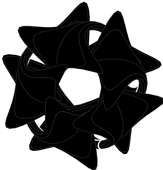
Représentation d'une surface tube autour d'un noeud de tore
