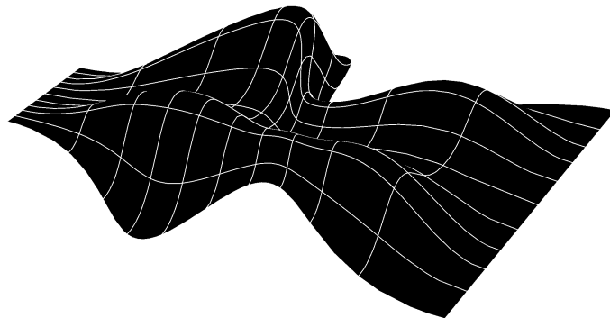
Représentation de la famille de surfaces homéomorphes au plan \mathbb{R}^2 (non graph)
