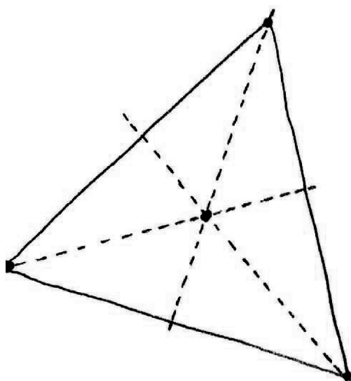
Représentation du groupe de symétrie ponctuelle discrète C_3 du triangle équilatéral
