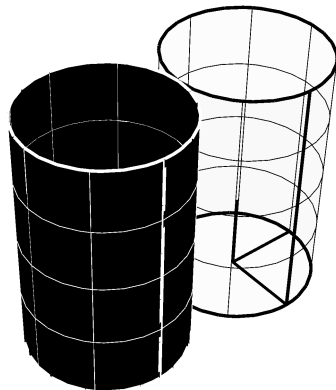
Représentation d'une réflexion d'un cylindre dans l'espace euclidien \mathbb{R}^3
