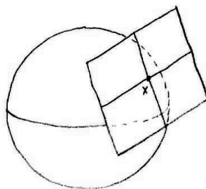
Représentation de la sphère (variété de deux dimensions) et son espace tangent
