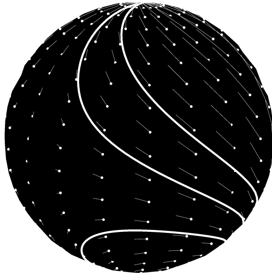
Représentation du flot d'un champ de vecteurs non linéaire du plan et son poussé en avant sur la surface
