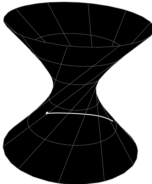
Représentation de la courbe géodésique sur une surface régulière
