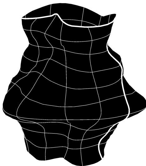
Représentation de la surface adapté à l'aide de l'homotopie
