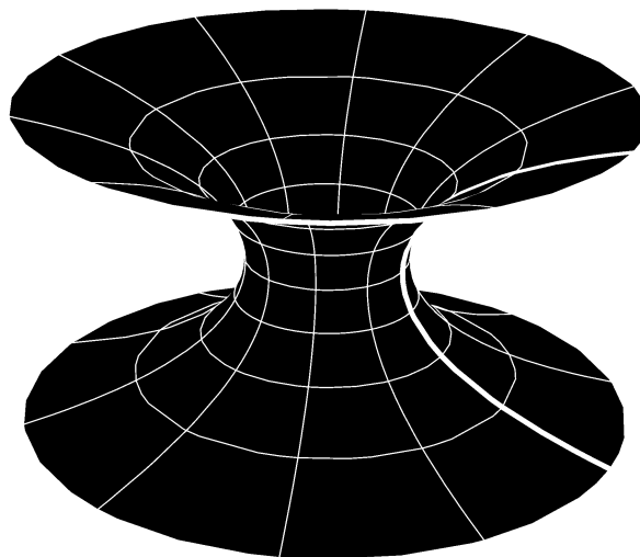
Représentation d'une surface de révolution (caténoïde)
