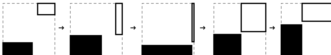
Représentation de la convergence vers le centre du carré
