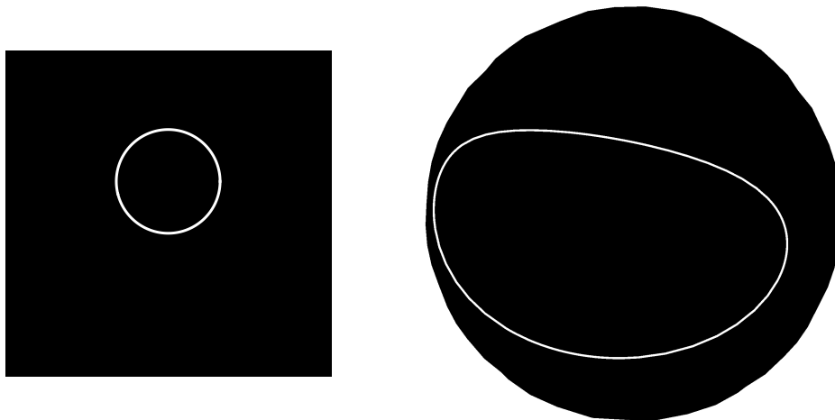
Représentation de l'envoi d'une courbe du plan à une surface régulière
