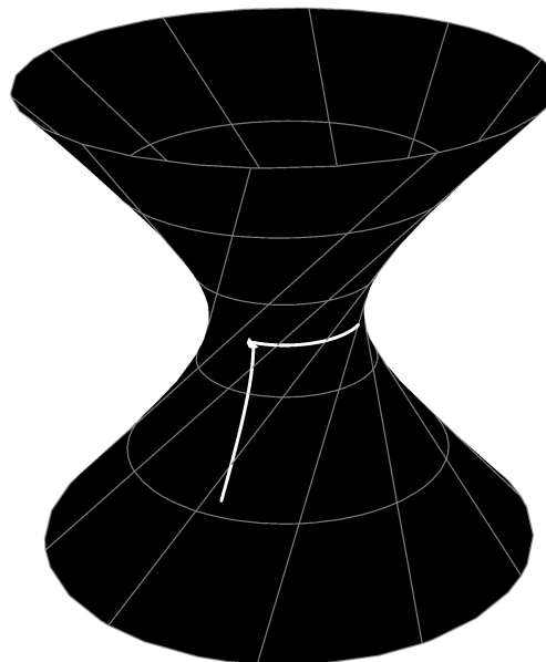
Représentation des courbes principales d'une surface régulière
