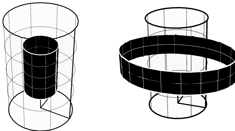
Représentation d'une homothétie et une mise à l'échelle non uniforme d'un cylindre dans l'espace euclidien \mathbb{R}^3
