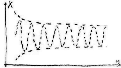
(X, d) n'est pas complet
